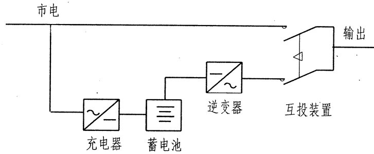
EPS应急电源系统方框图
