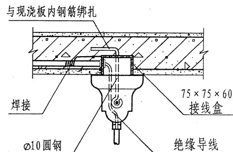
现浇楼板上安装
