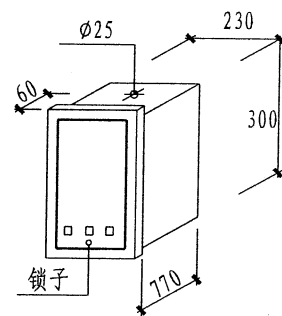
控制按钮箱
