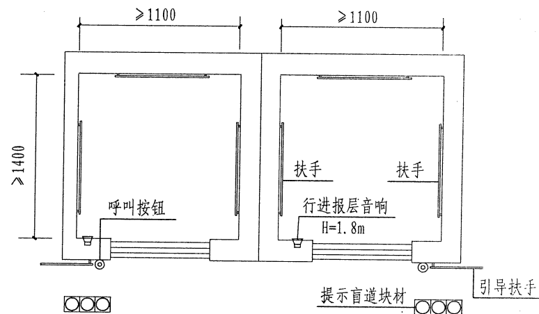
双电梯平面
