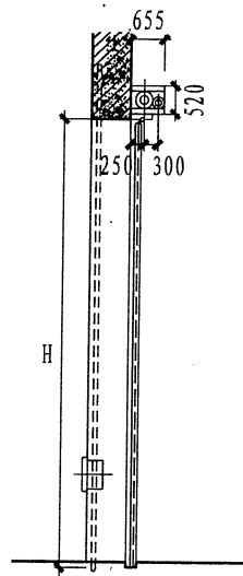
剖面
