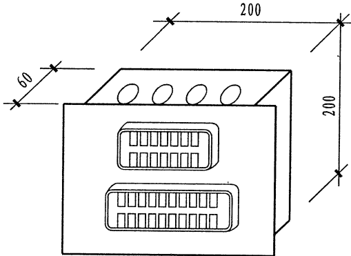
DY-DZ3端子箱 (14线+20线)
