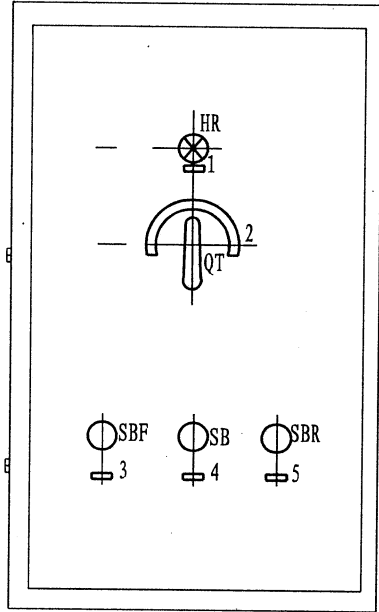
箱门正视图
