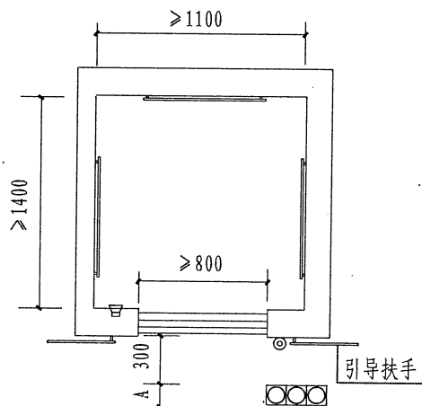
单电梯平面
