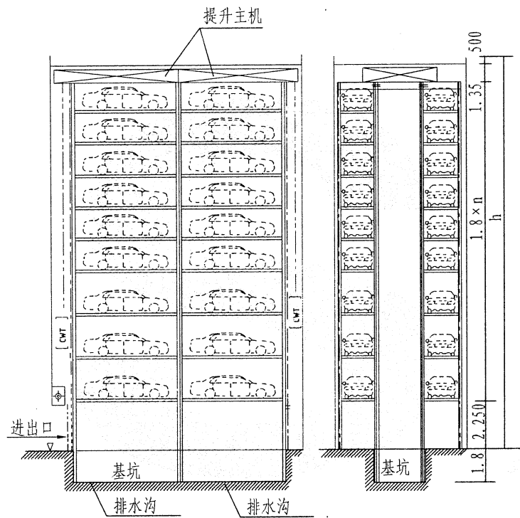
双塔纵列型
