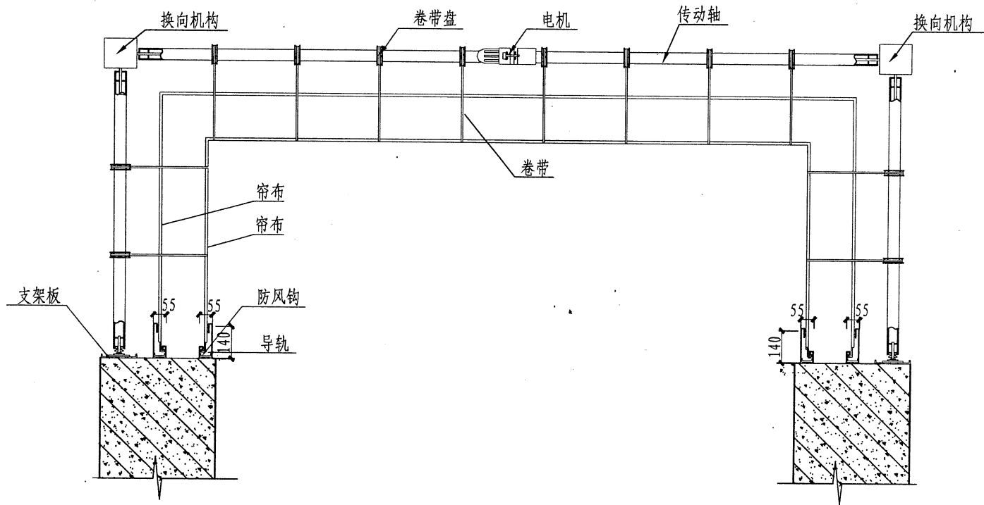
平面示意图
