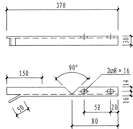
角钢支架
