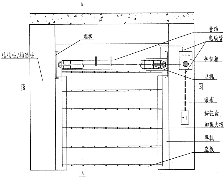
立 面
