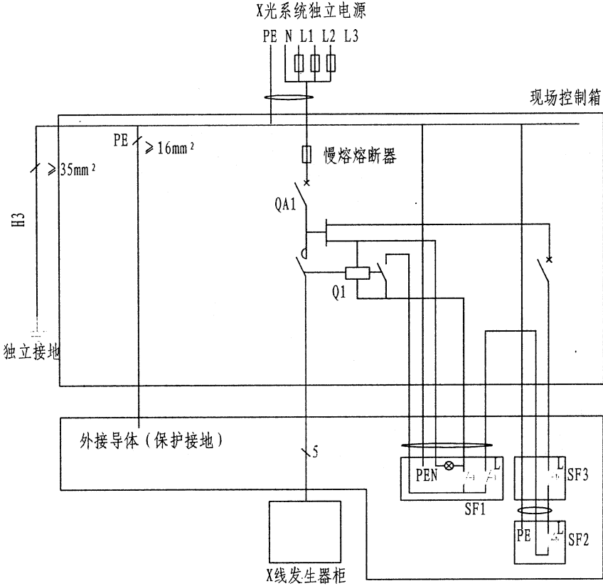
数字肠胃检查室系统示例
