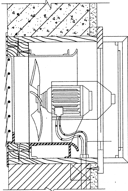
1-1剖面
