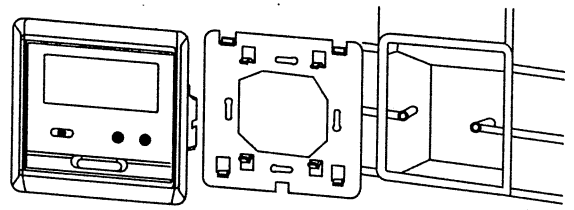
温控器安装组合图
