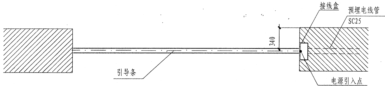
无轨单开门无掩体示意图
