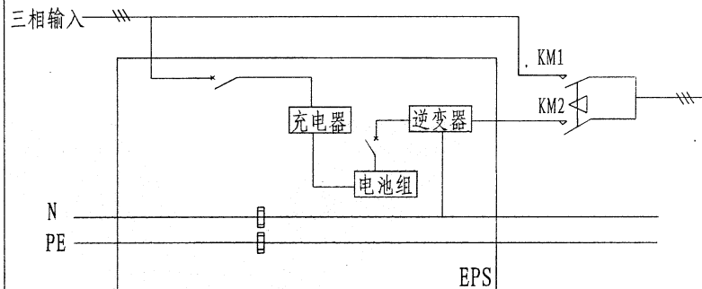
YJS三相双电源原理图
