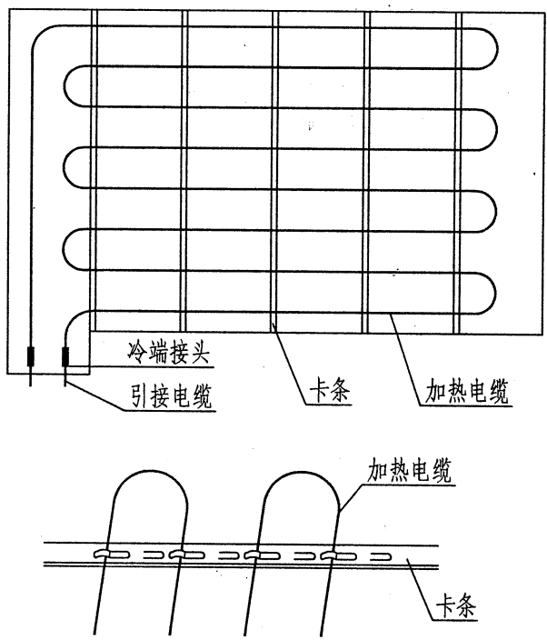
加热电缆坡道防滑安装示意图
