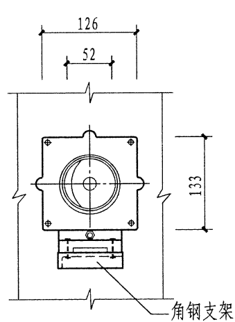
电 笛
