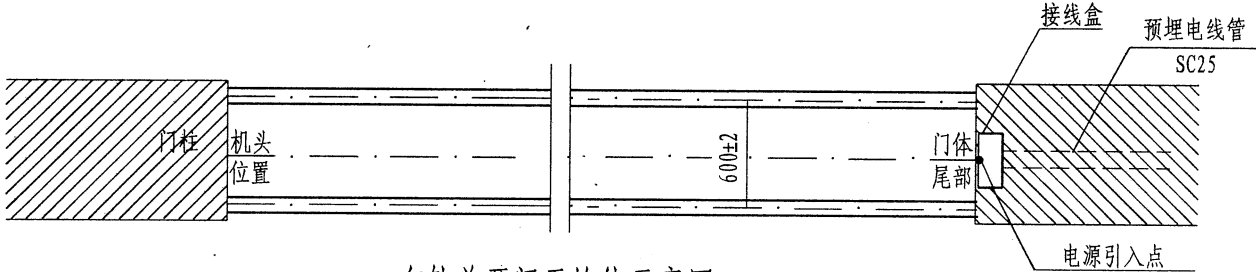
有轨单开门无掩体示意图
