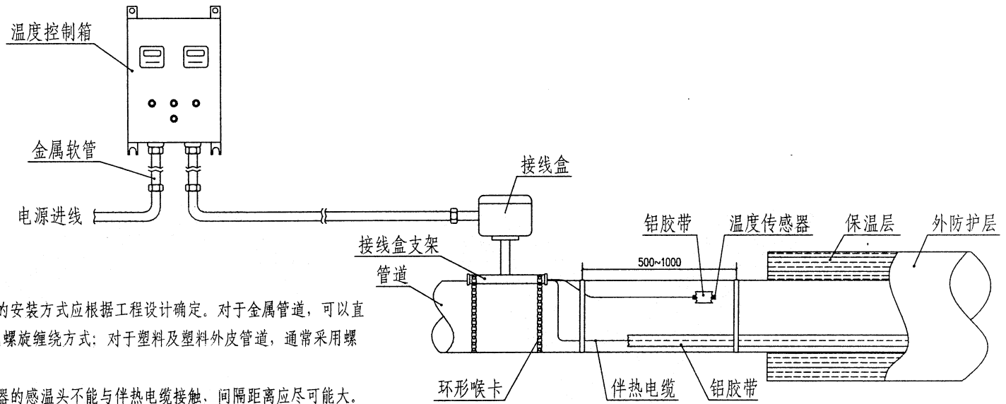
伴热电缆采用铝胶带固定
