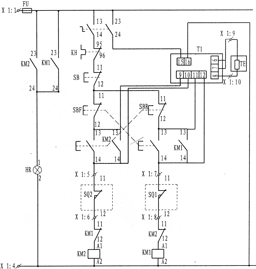
控制回路
