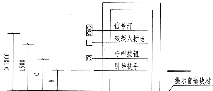
单电梯立面
