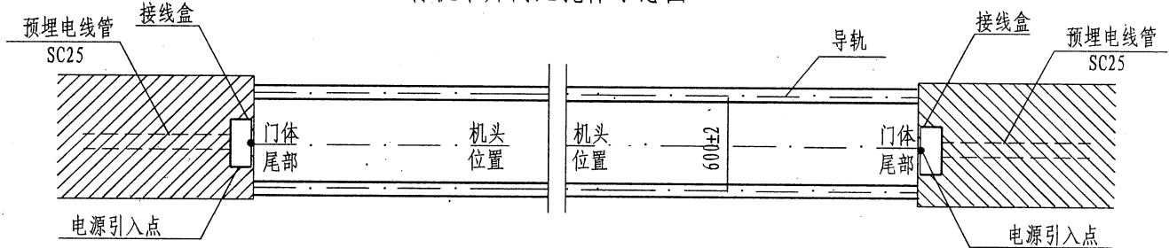
有轨双开门无掩体示意图
