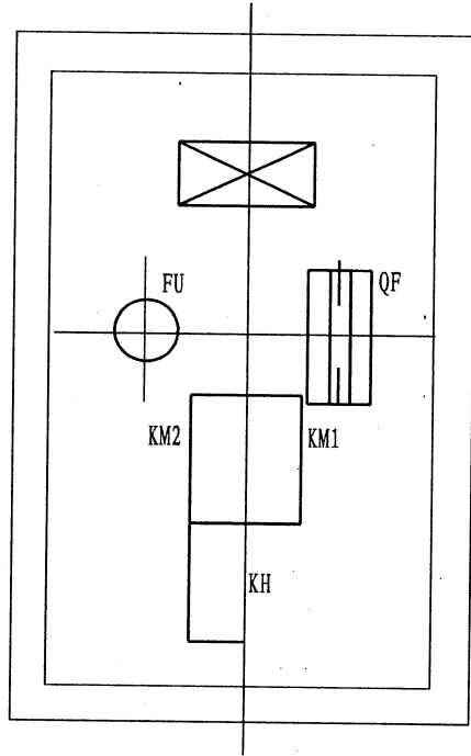
无门正视图
