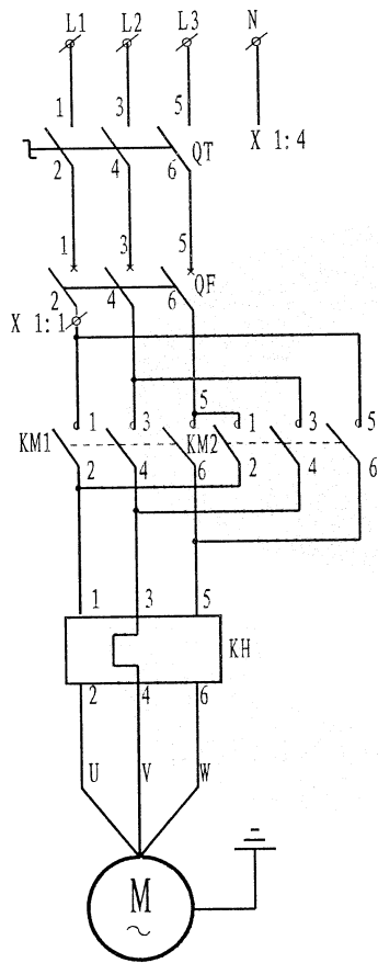
主回路
