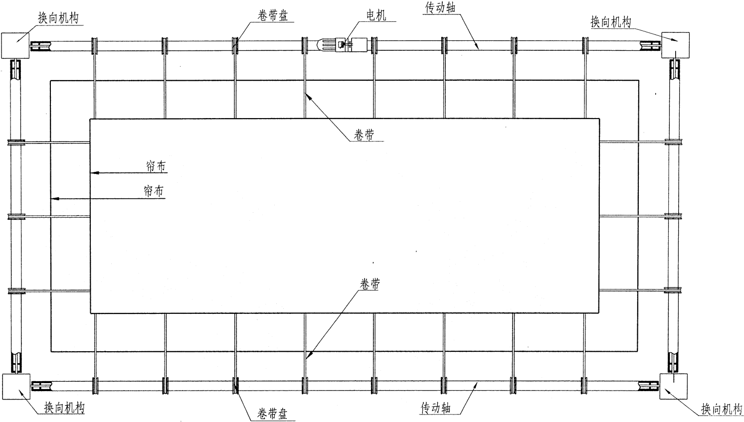
平面示意图
