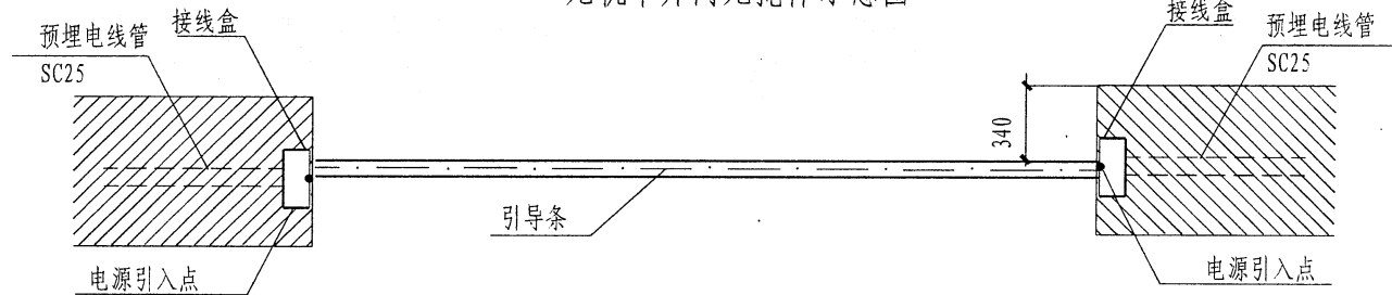
无轨双开门无掩体示意图
