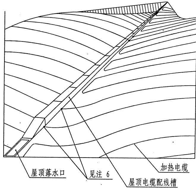
加热电缆屋顶融雪安装示意图
