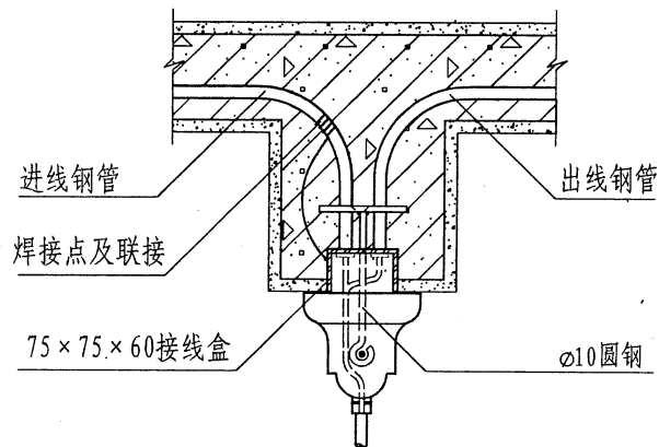
现浇梁上安装
