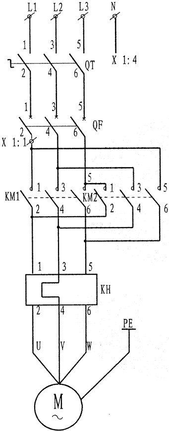
主回路
