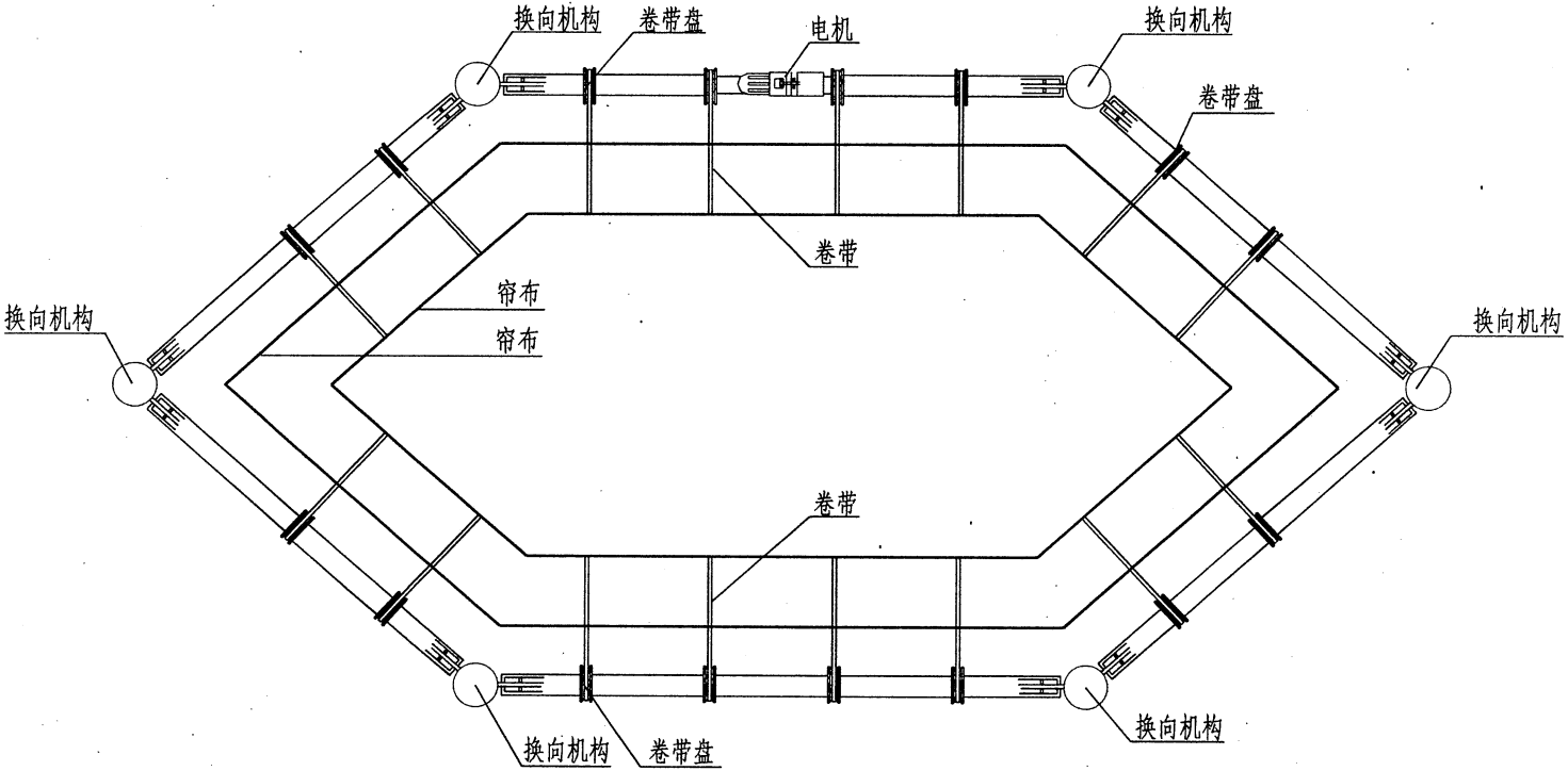
平面示意图
