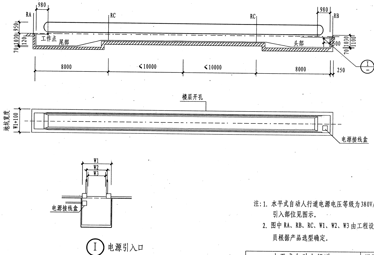
水平式自动人行道 电源引入部位示意图
