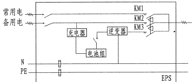
YJS三相双电源原理图
