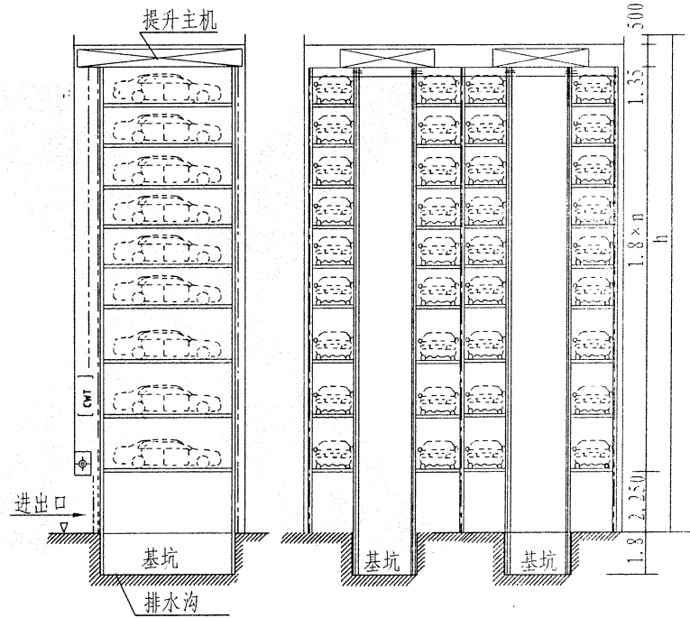
双塔并列型
