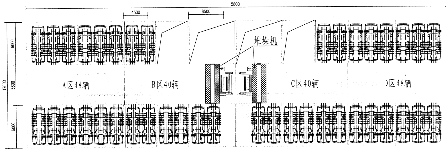
地下一、二层平面图
