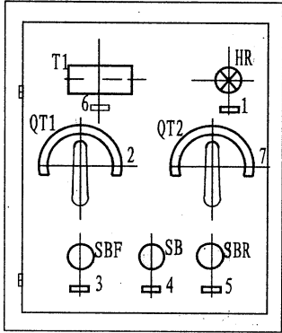
箱门正视图
