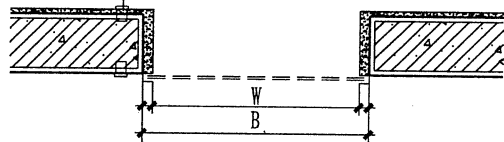
平面
