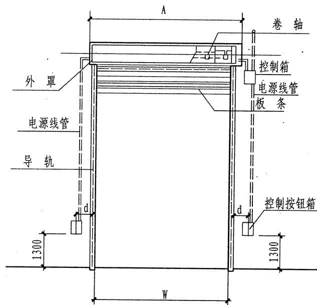
立面
