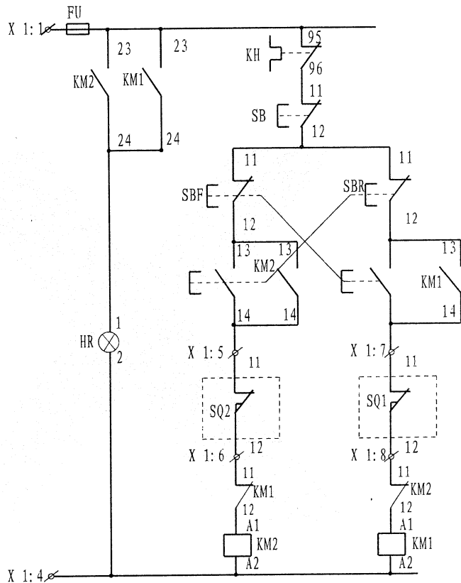
控制回路
