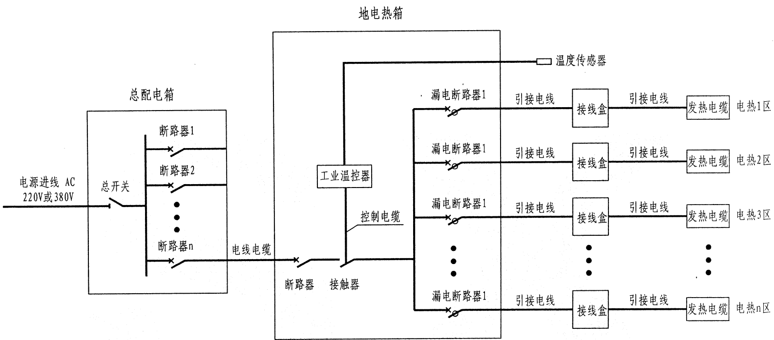
加热带地面辐射供热系统电气系统框图（二）
