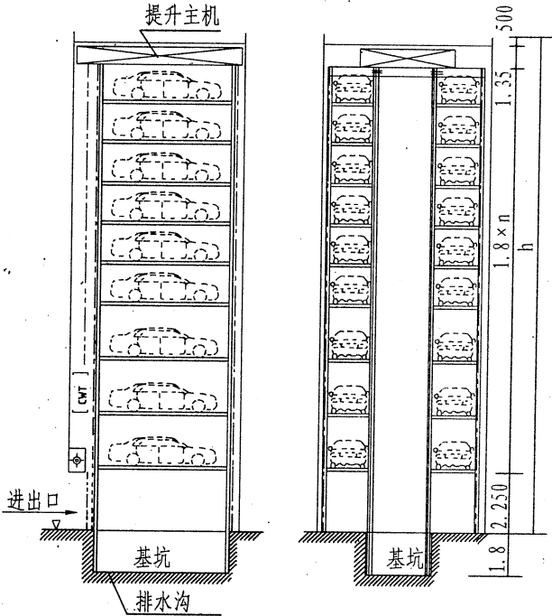
单塔单列型
