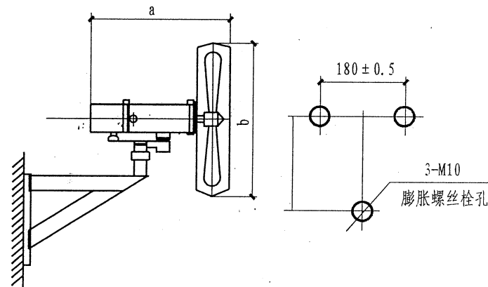
摇头扇壁装
