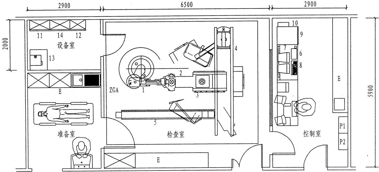
DSA检查室平面布置示例
