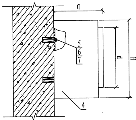
数据采集器箱墙上明装
