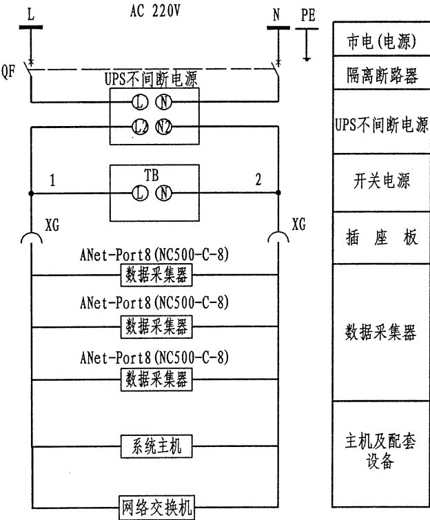
系统管理控制柜电源接线图
