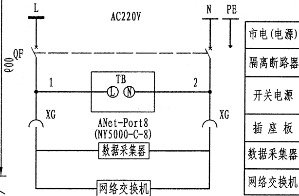
数据采集器箱电源接线图
