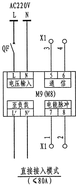
接线端子图
