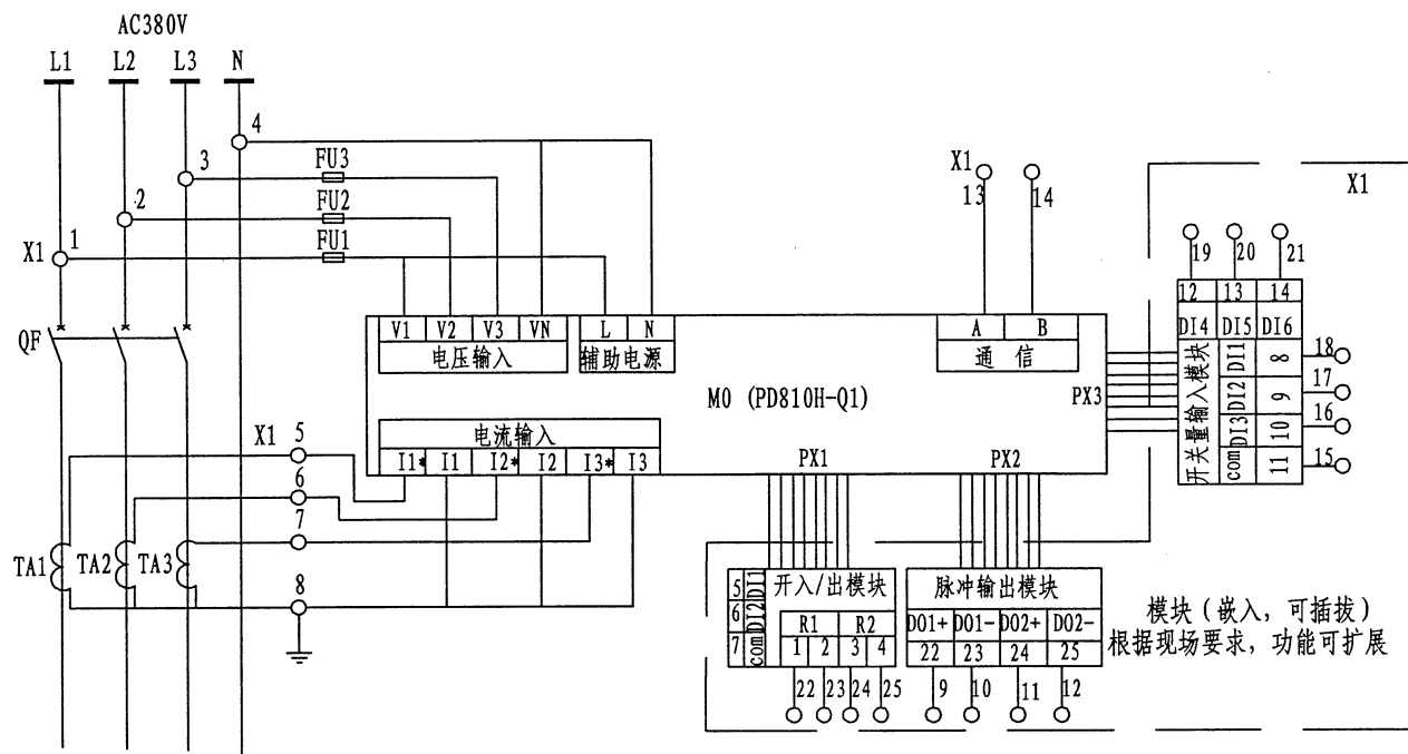
互感器接入模式
