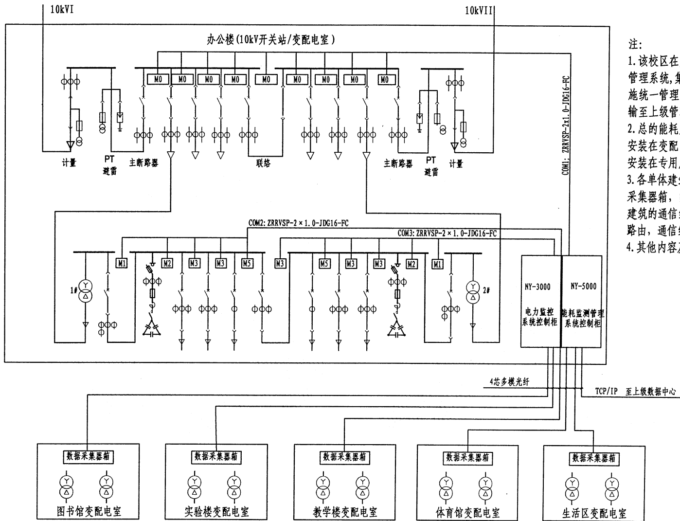
某校区建筑能耗监测系统组网图
