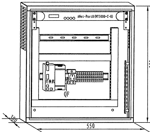
数据采集器箱组装示意图
