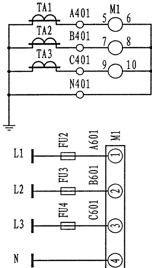
电流测量回路 电压测量回路
