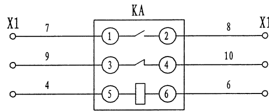
外部继电器接线图
