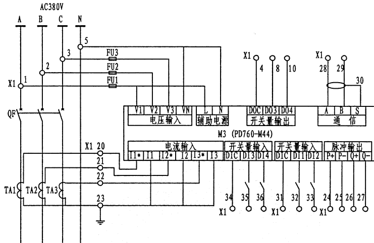
互感器接入模式
