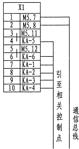
接线端子图
