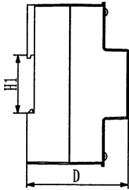
导轨式侧视图
