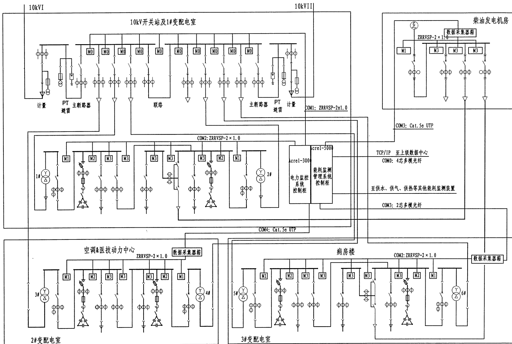
某医疗单位能耗监测系统组网图 (一)
