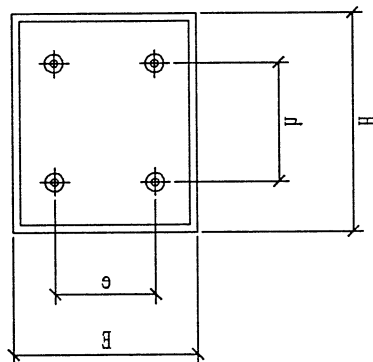
数据采集器箱外形安装尺寸
