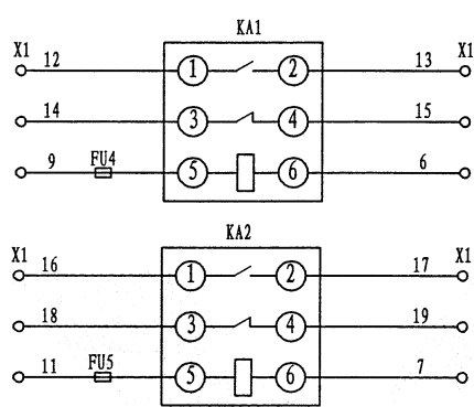
外配继电器接线图
