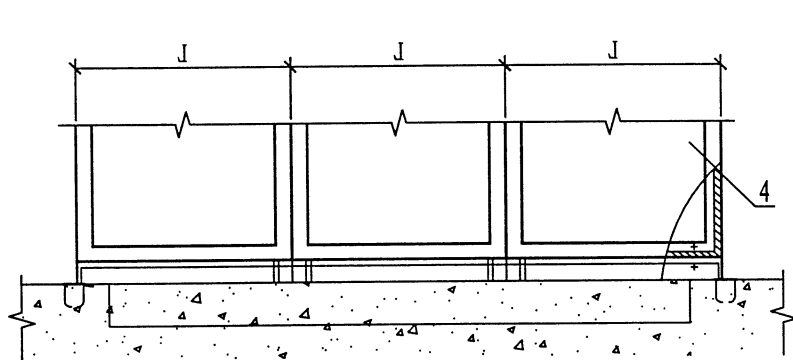
系统管理控制柜落地安装（多台）
