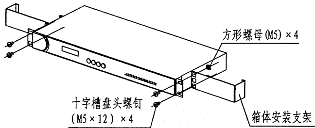
数据采集器与箱体组装示意图
