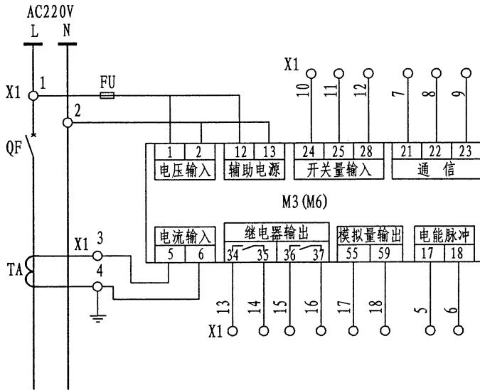
互感器接入模式
