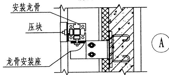
阳台光伏组件安装详图
