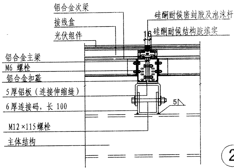
主、次梁连接节点
