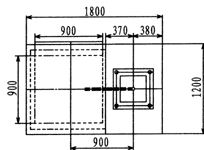
路灯基础俯视图
