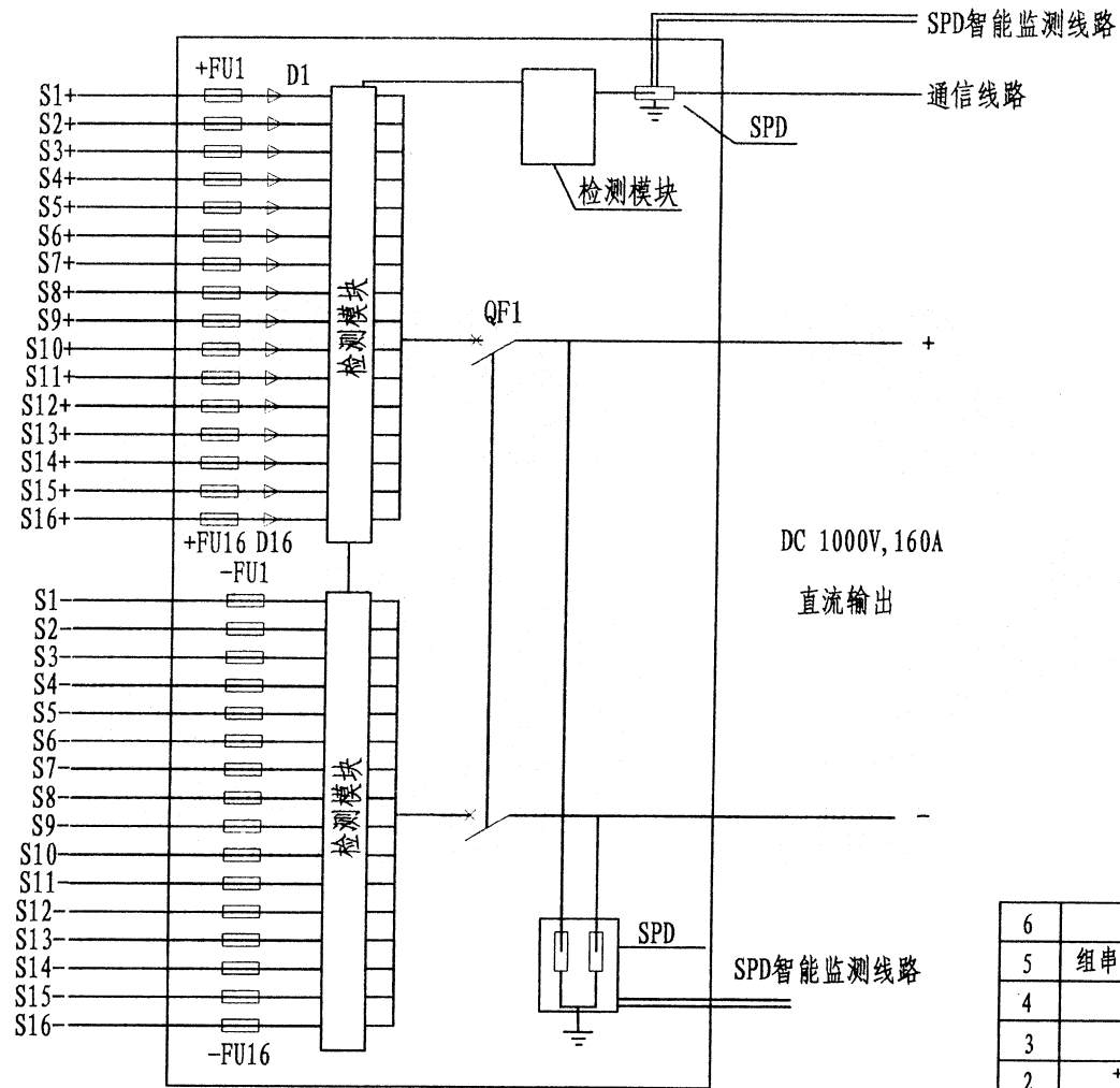
智能光伏防雷汇流箱系统图
