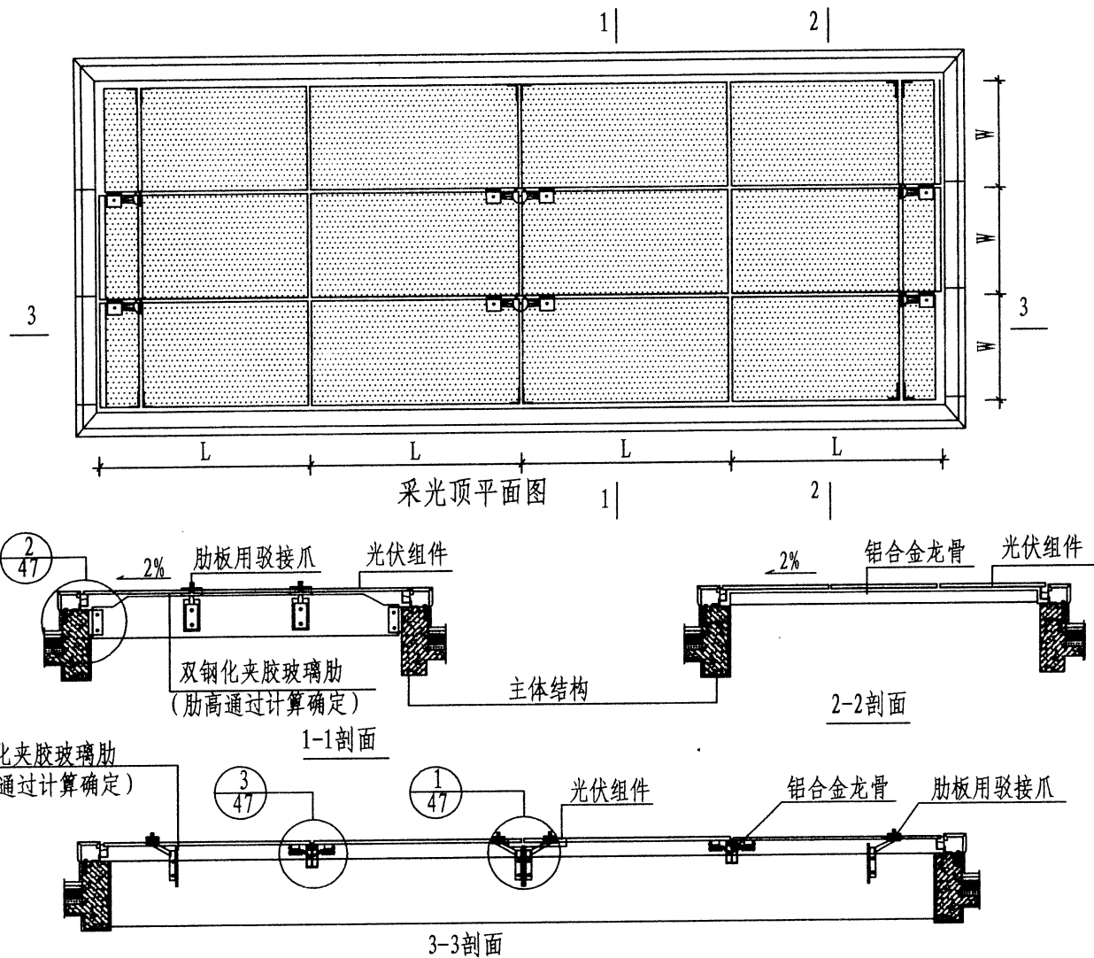
肋点式光伏采光顶组（构）件布置图
