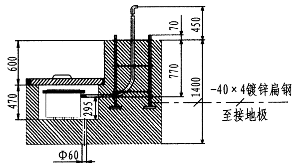
路灯基础剖面图
