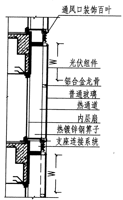
1-1 剖面图
