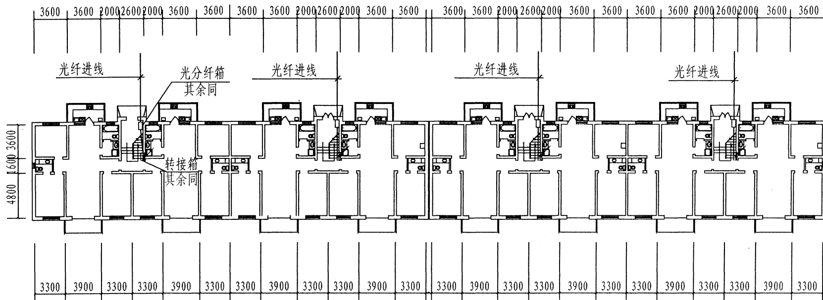
楼层平面图
