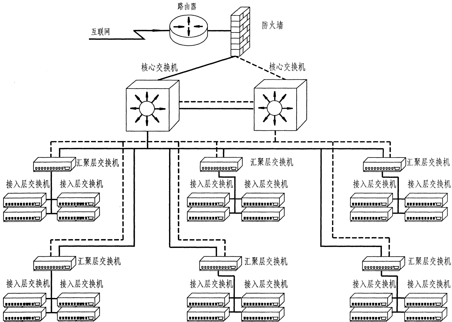
双核心网络结构图
