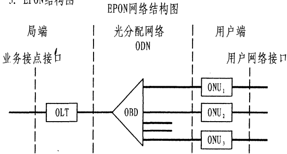
EPON网络树型结构图 I
