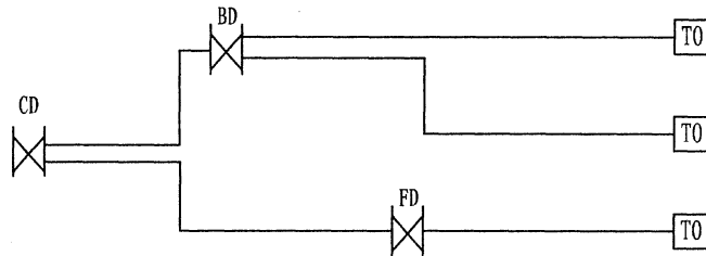
综合布线子系统构成 (a)
