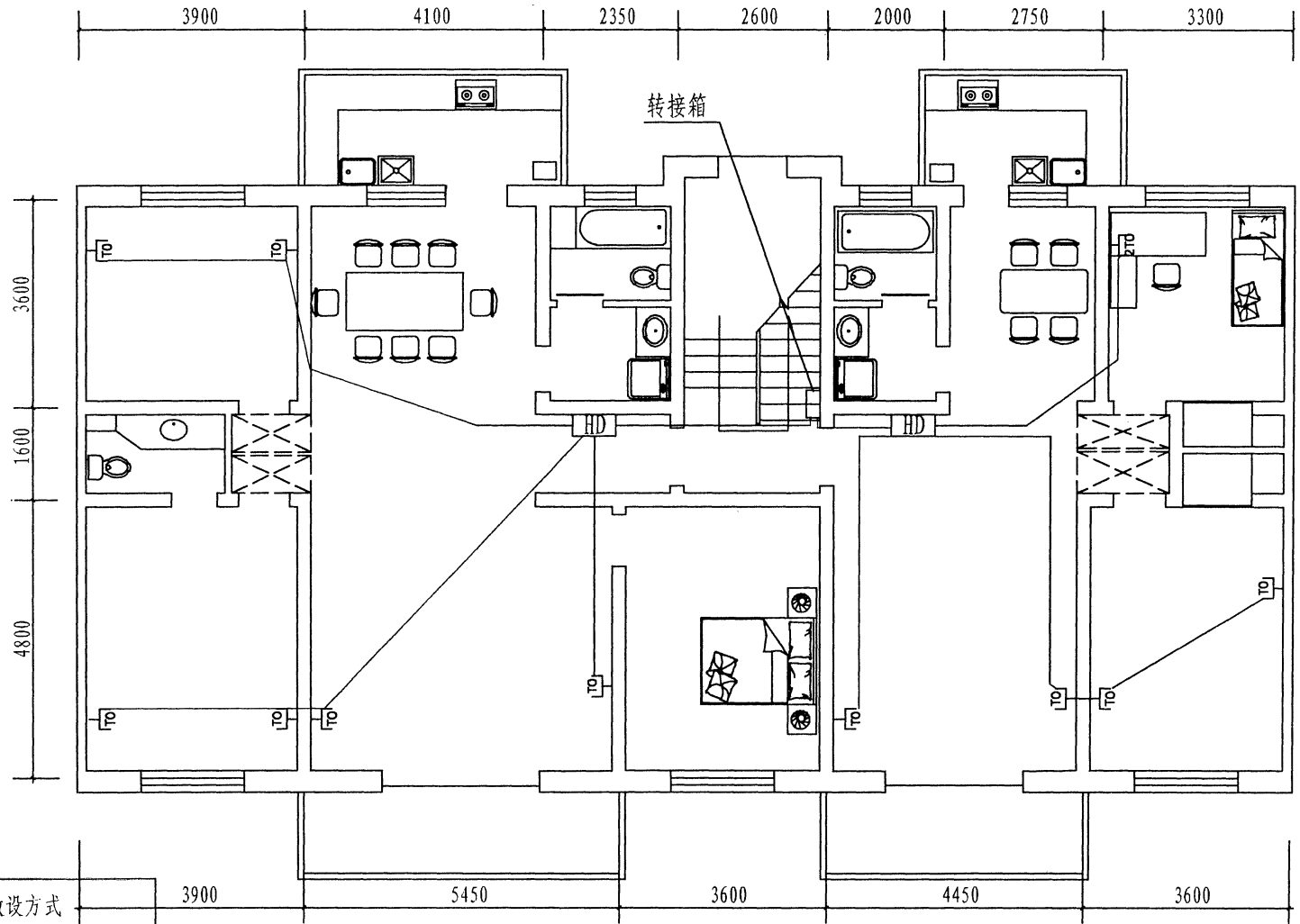
单元平面图
