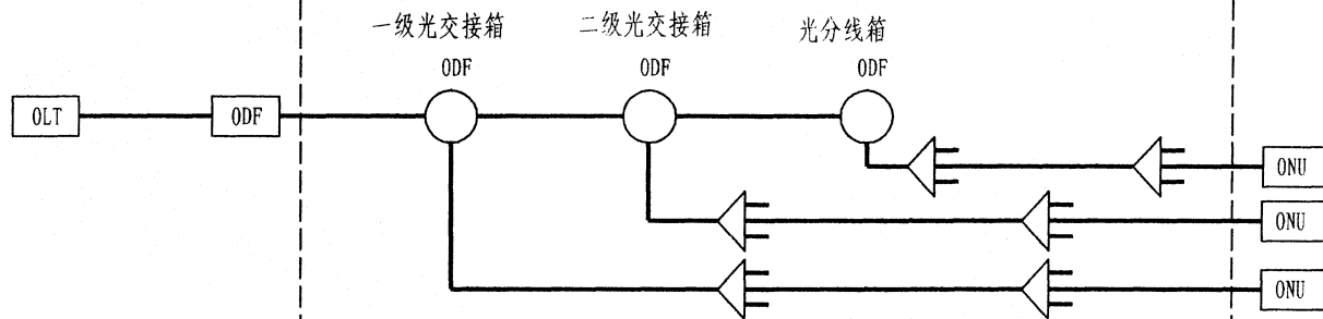
二级分光无源光网络结构图 I
