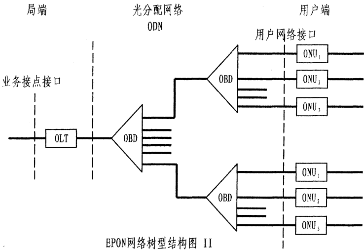
EPON网络树型结构图 II
