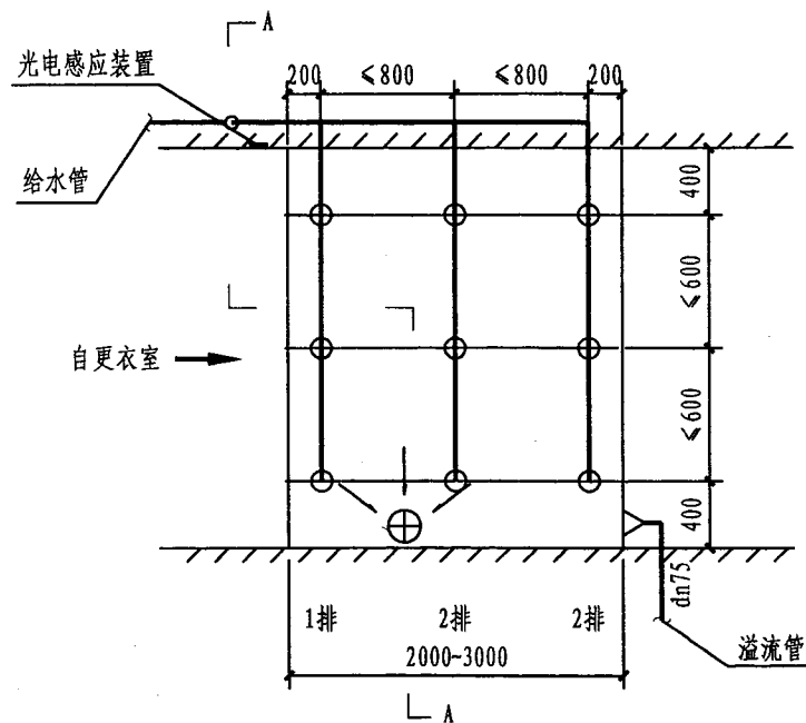
平面图
