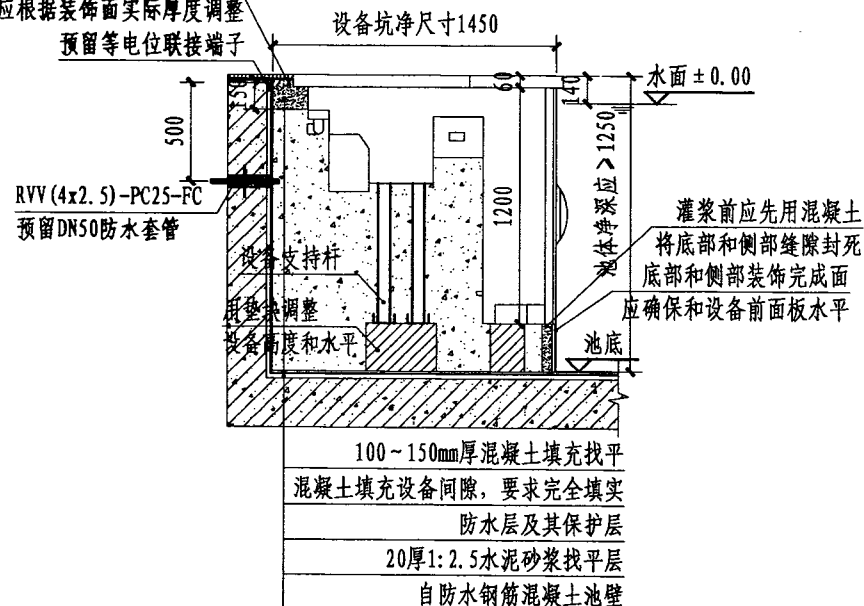
A-A 剖面图
