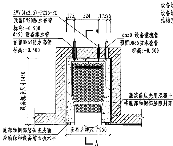
设备坑平面图
