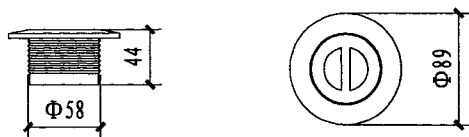
WL-ACW01吸污口
