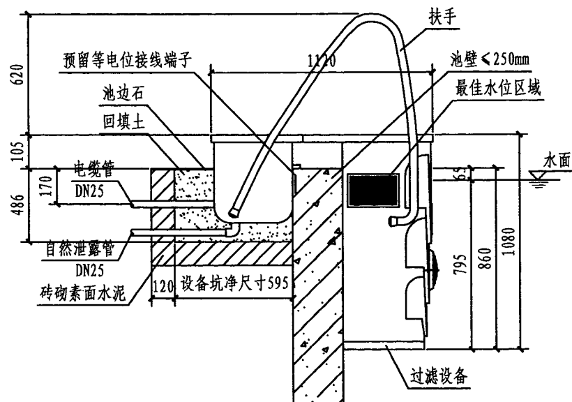
A-A 剖面图
