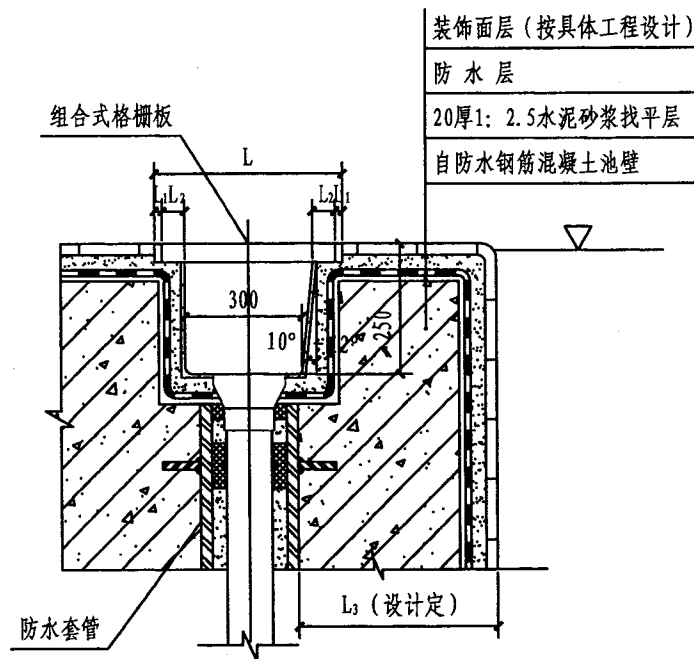
溢流回水槽格栅板、回水口安装图
