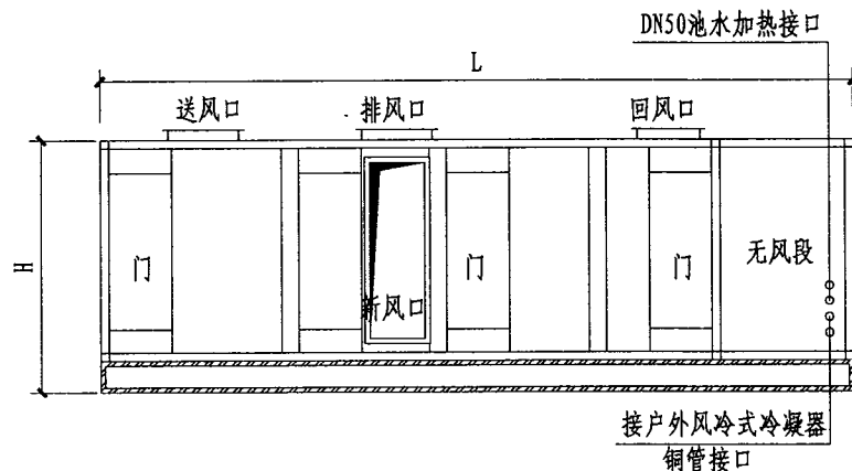
A-A 立面图
