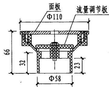
A-A
