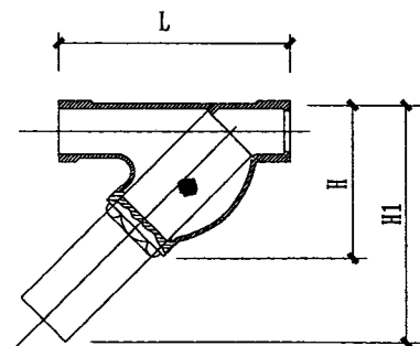
SG11H型
