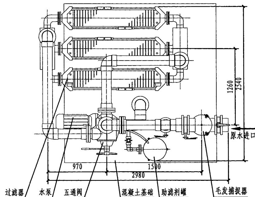
平面图
