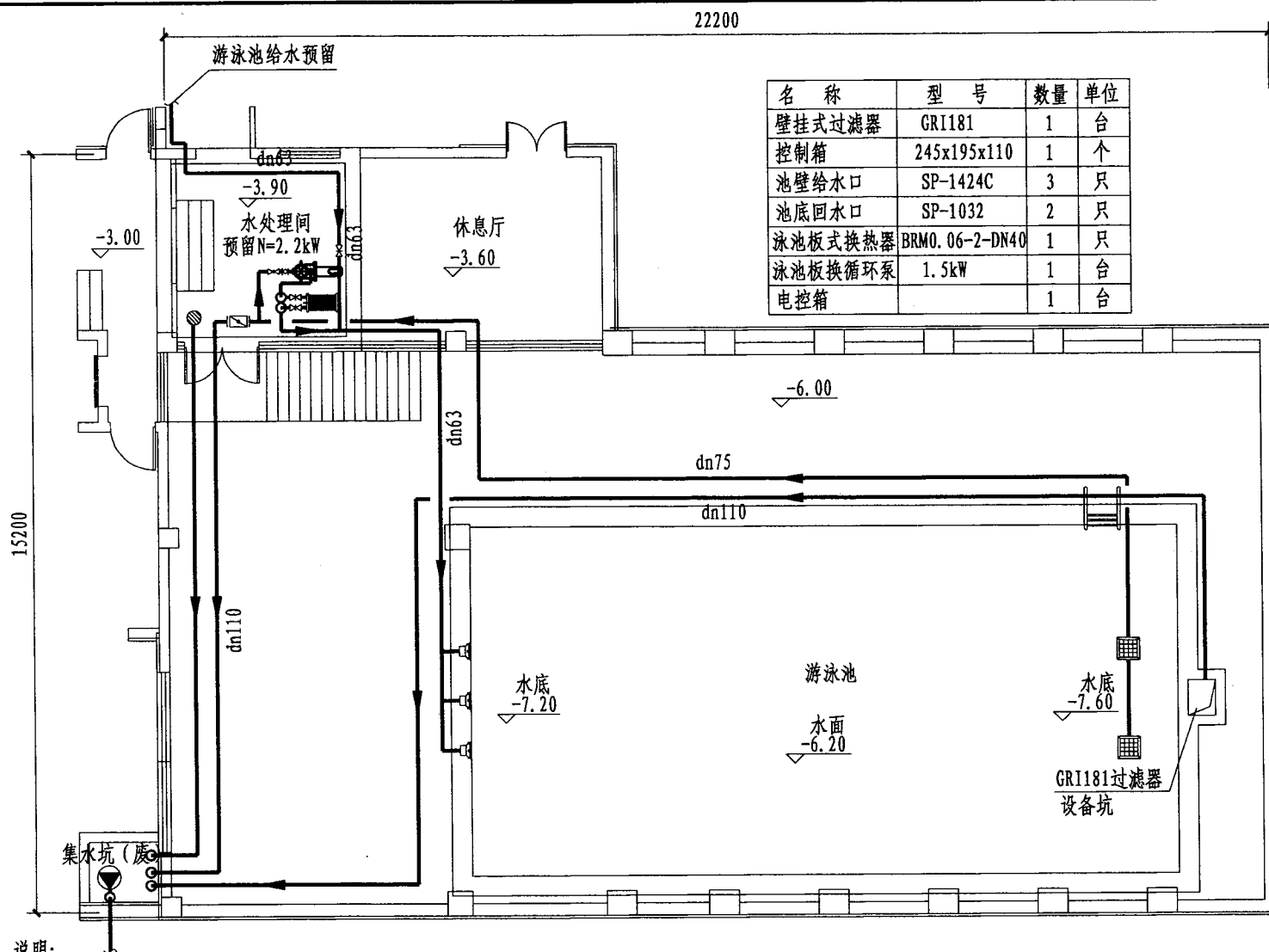
工程案例一：泳池给排水管道平面图
