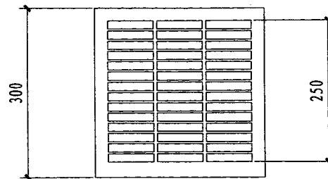
SP-1032回水口
