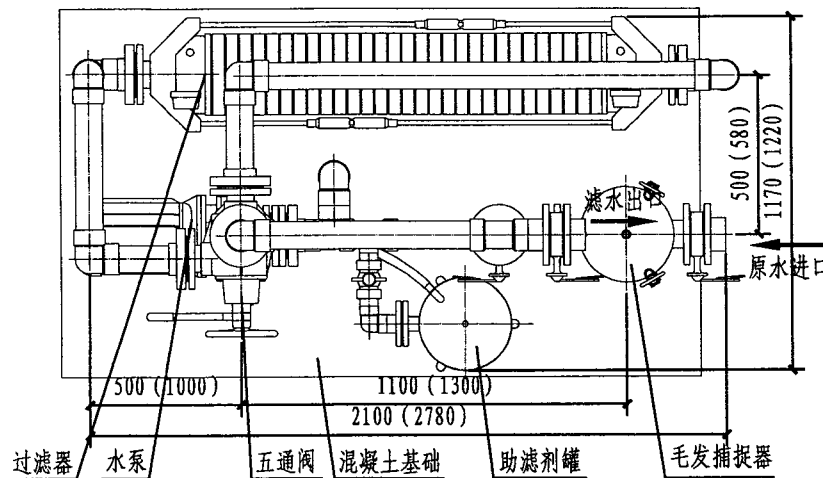
平面图
