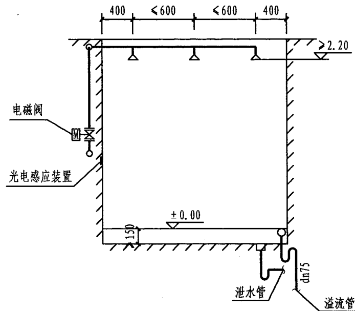
A-A剖面图
