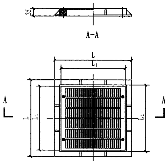
WL-ADP263回水口
