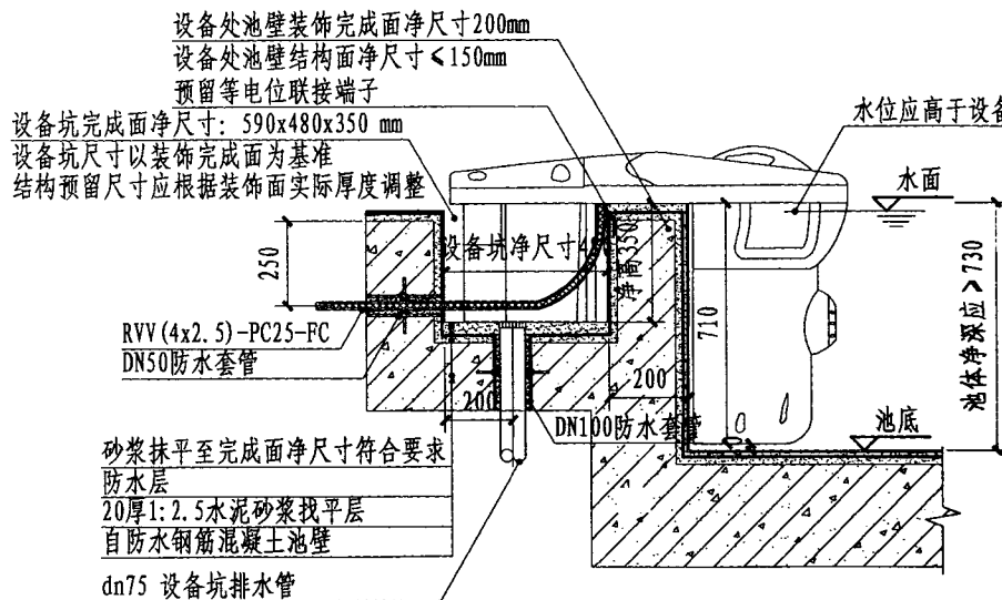
A-A 剖面图
