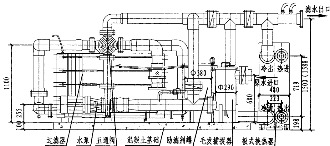
立视图
