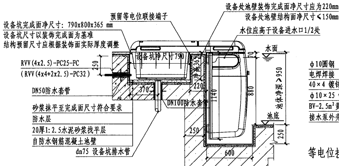
A-A 剖面图
