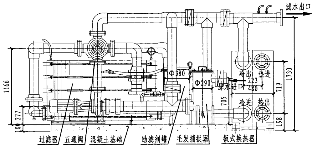
立面图
