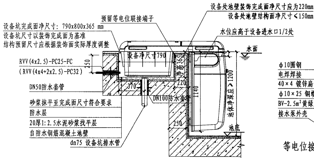
A-A 剖面图
