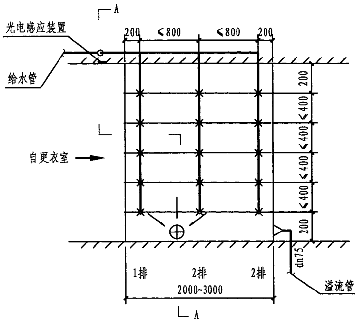
平面图
