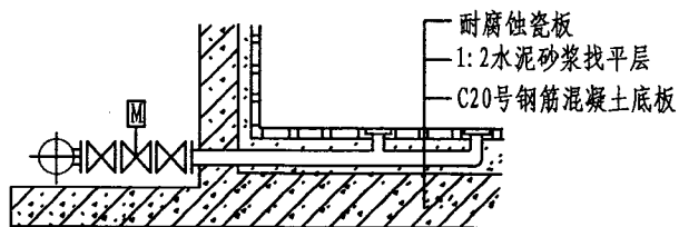
A-A剖面图
