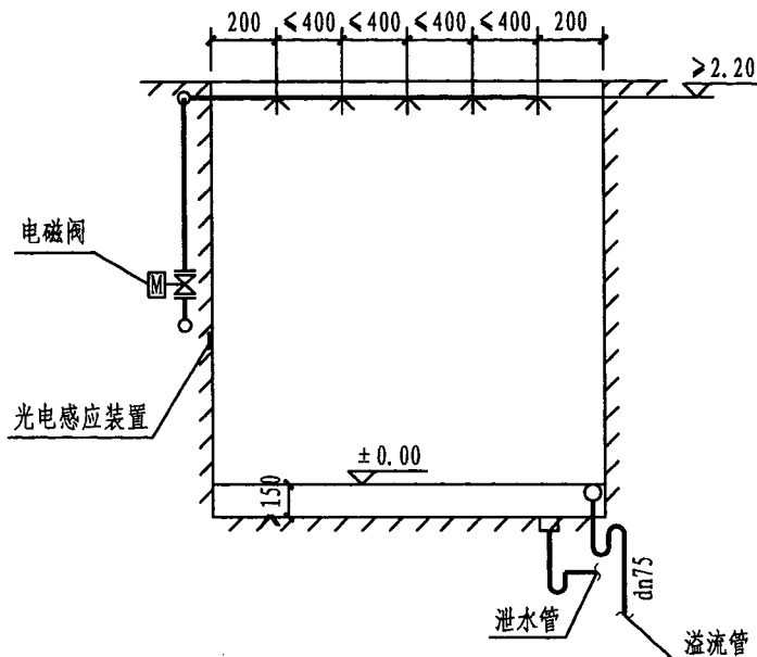
A-A剖面图
