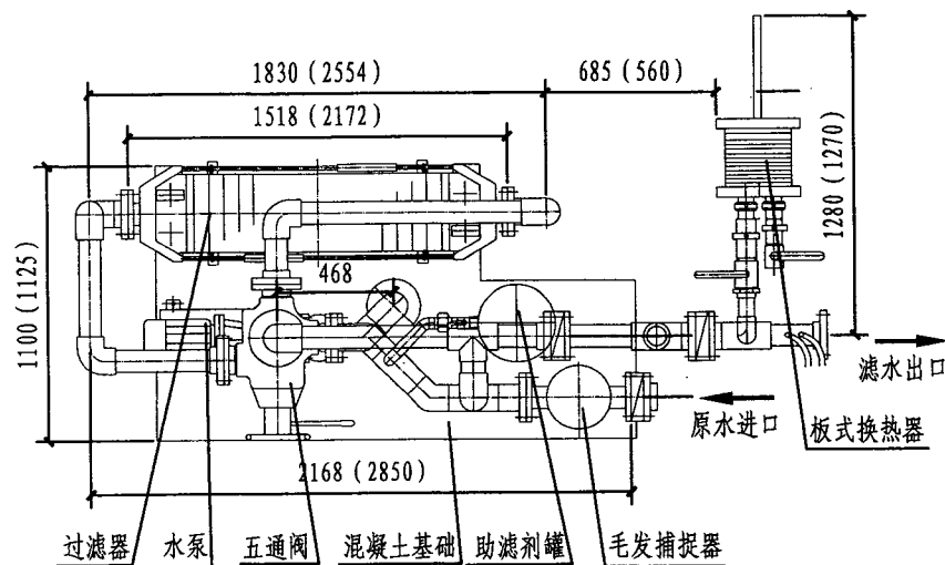
平面图
