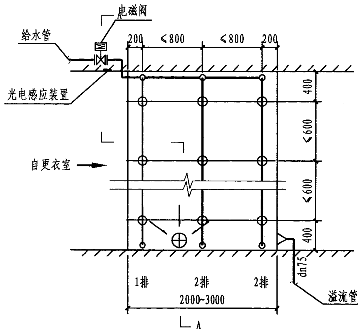
平面图
