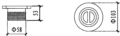
WL-ACW02吸污口
