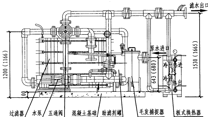
立面图
