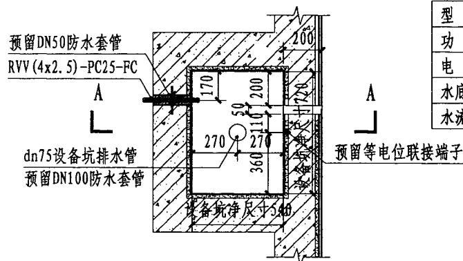
设备坑平面图
