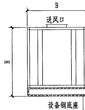
B-B 侧视图
