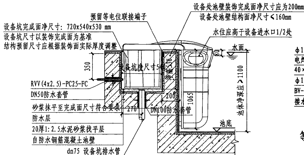
A-A 剖面图
