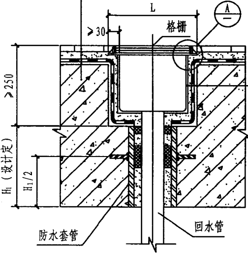
回水口安装 (a)
