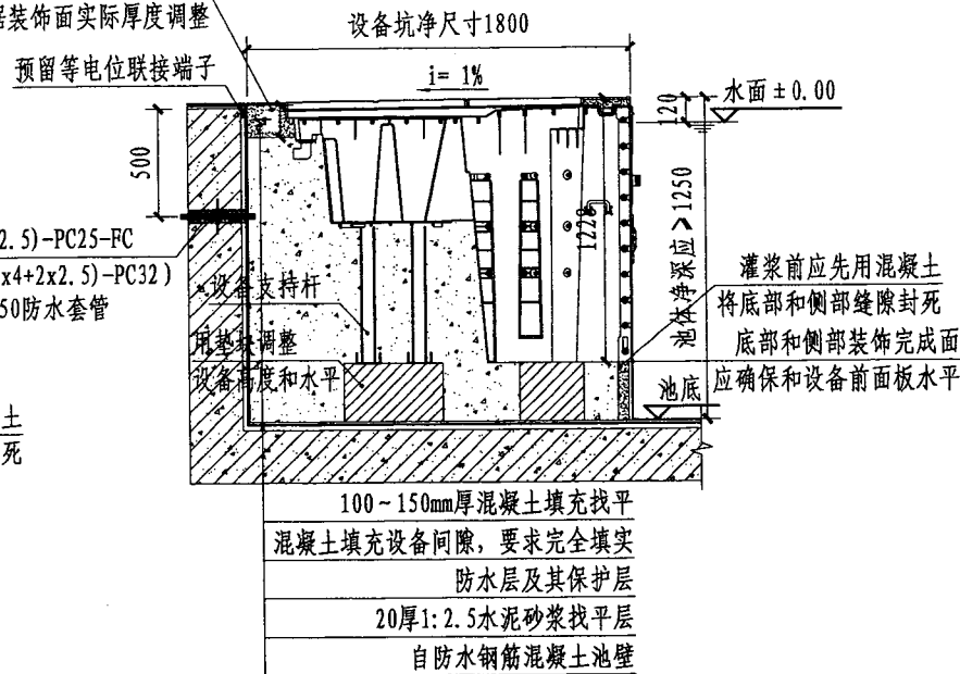
A-A 剖面图
