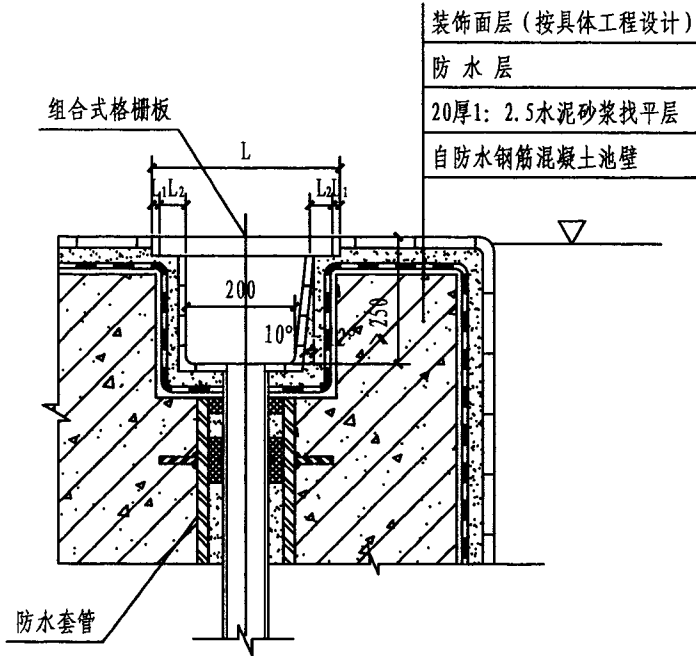
溢水槽格栅板及排水管安装图
