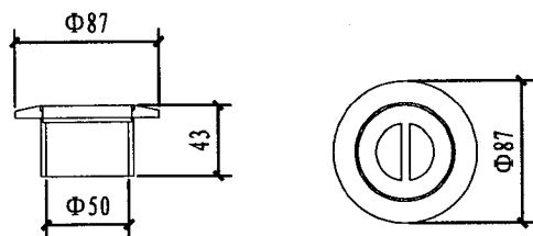
SP-1022吸污口
