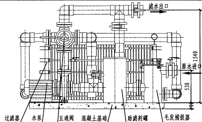
立视图
