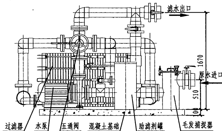
立面图
