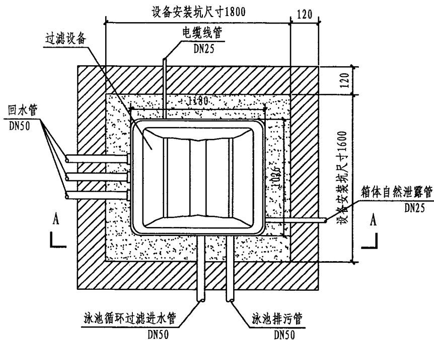
设备坑平面图
