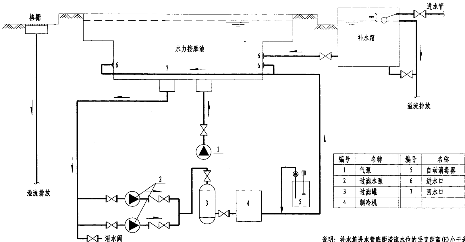
冷水池工艺流程
