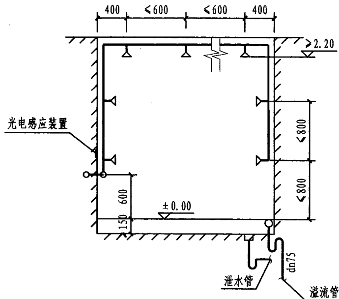
A-A剖面图
