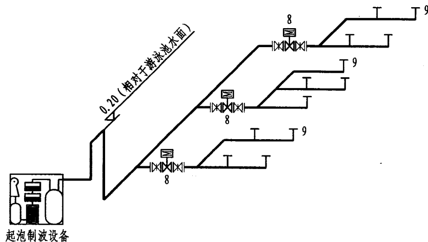
跳台或跳板前方局部制波系统图
