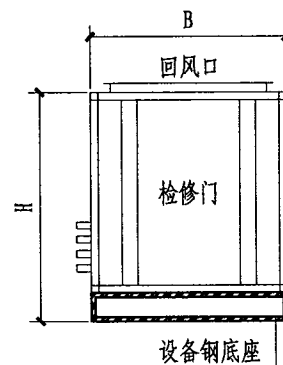
C-C 侧视图
