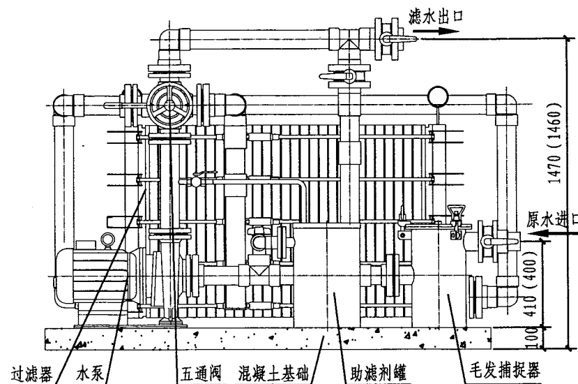
立面图
