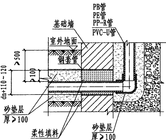
穿基础墙
