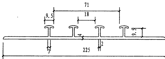
PE内接管截面尺寸
