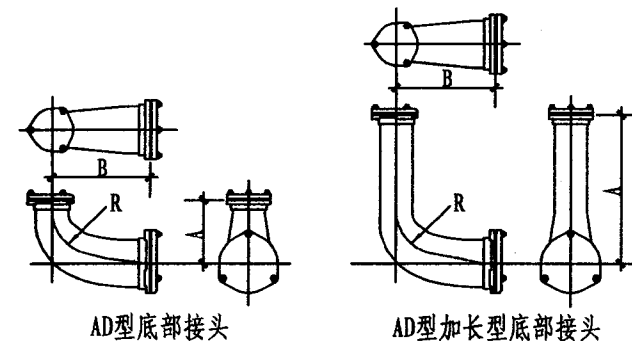
AD型底部接头规格尺寸 (mm)
