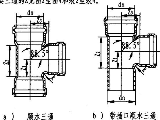
图2 顺水三通
