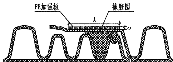
连接示意图
