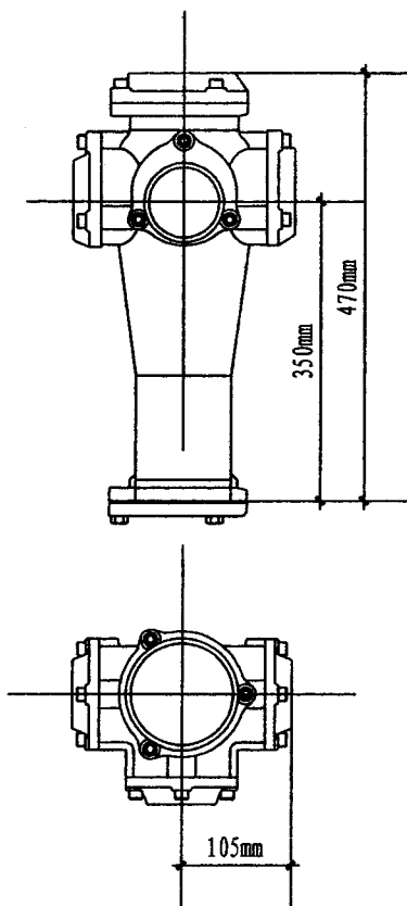
五通加强型接头 型号: C-5005
