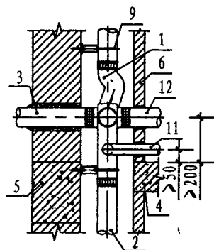
竖向安装图II
