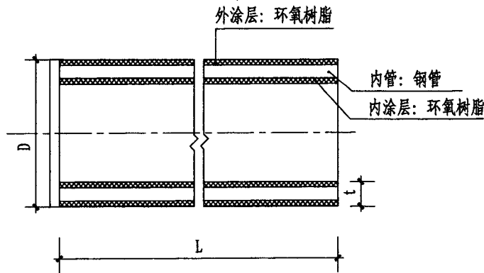
涂塑环氧树脂复合钢管结构图
