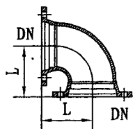
等径90°弯头
