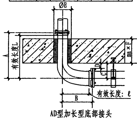
AD型加长型底部接头规格尺寸 (mm)
