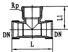
内螺纹三通
