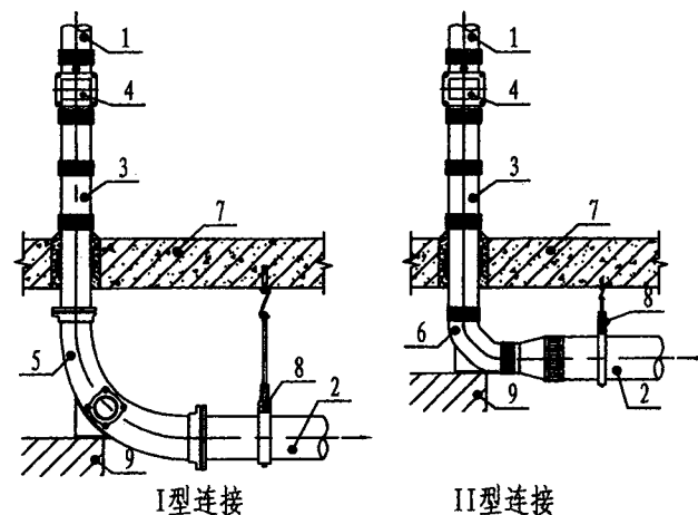
排水立管底部弯头及横干管(排水出户管)连接型式
