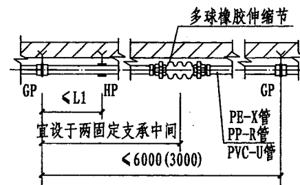
多球橡胶伸缩节补偿
