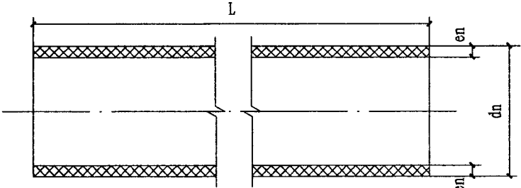
管材规格系列及壁厚基本尺寸
