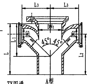
TY四通
