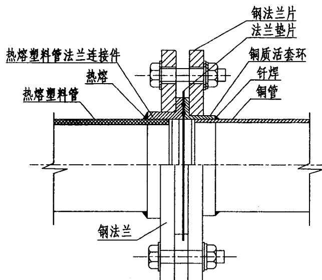
热熔塑料管与铜管
