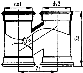
图8 H型管件
