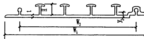
PE板材截面示意图
