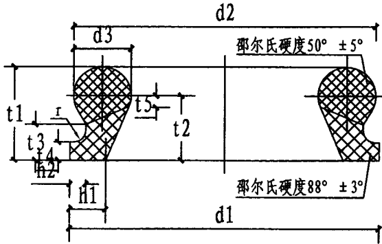
T型接口胶圈
