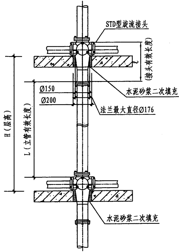
同层安装
