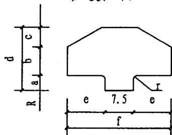
橡胶圈截面图
