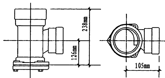
三通智能型接头 型号: D-3003A
