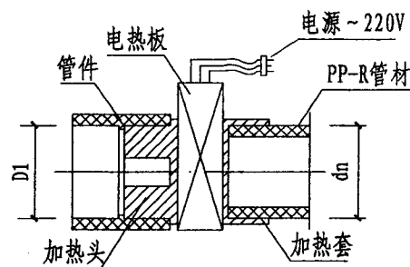
承口插口加热
