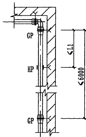
PVC-U管橡胶圈连接
