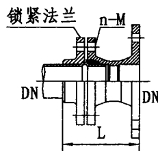
标准连接法兰
