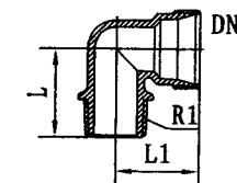
外螺纹90°弯头
