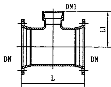
法兰-螺纹
