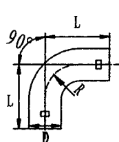
W型短弯头
