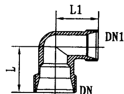
异径90°弯头
