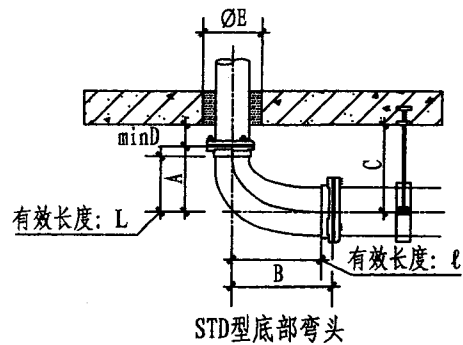
STD型底部弯头规格尺寸 (mm)
