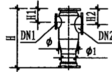
立面图
