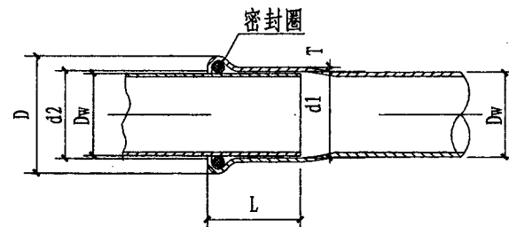
管件承口
