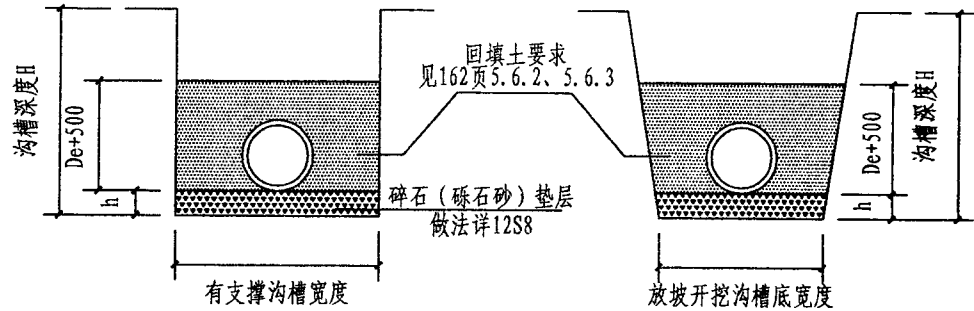
管道基础图
