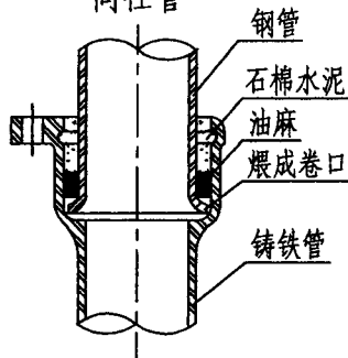
同径管
