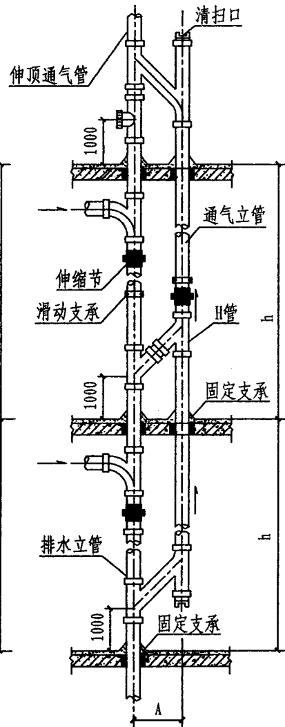
II 型
