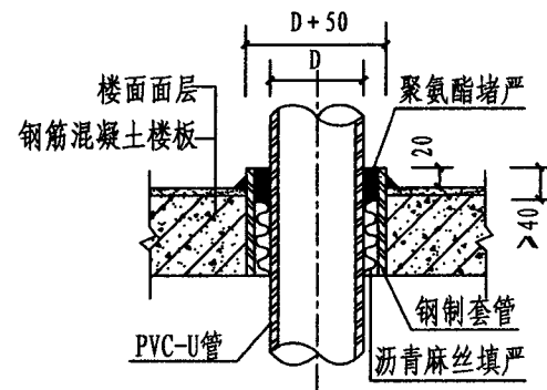
穿楼板 III
