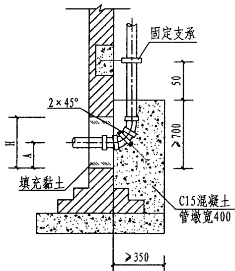
墙基留洞
