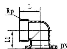
内螺纹90°弯头
