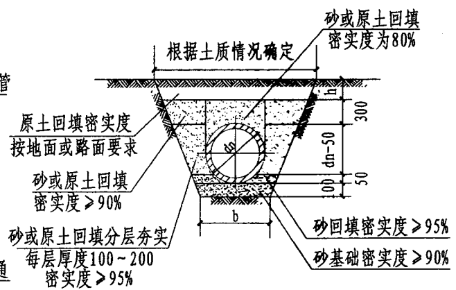
直埋或直埋穿越车行道
