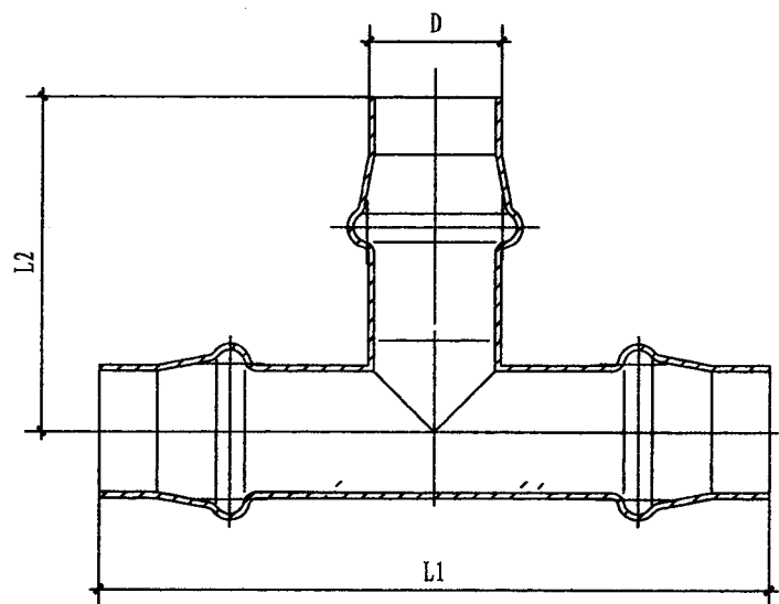
同径三通的基本尺寸 (单位: mm)
