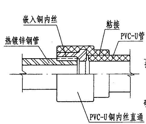
与衬塑热镀锌钢管连接
