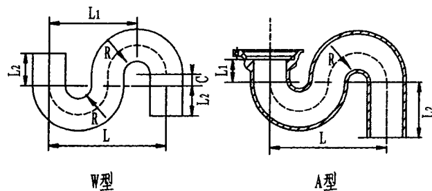
S型存水弯
