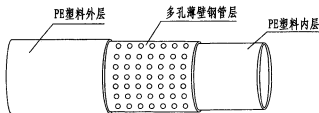
孔网钢带管结构图
