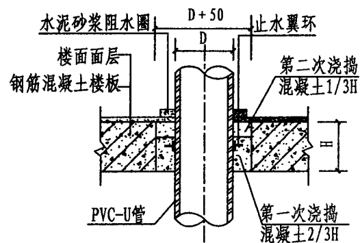
穿楼板 I
