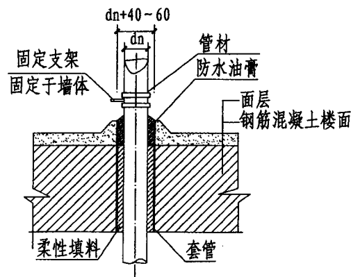
穿楼面 (二)
