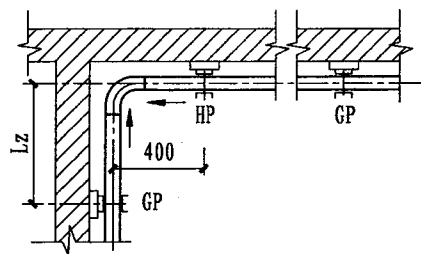
自由臂补偿
