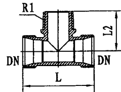
外螺纹三通
