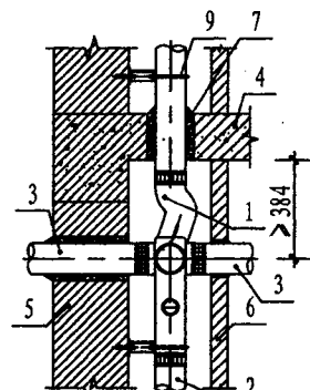
竖向安装图
