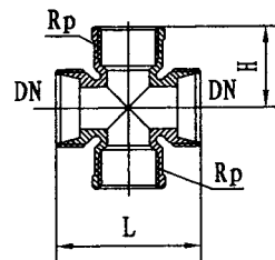
内螺纹四通
