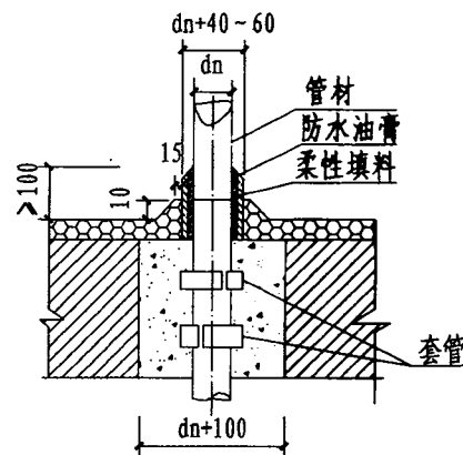
穿楼面 (一)
