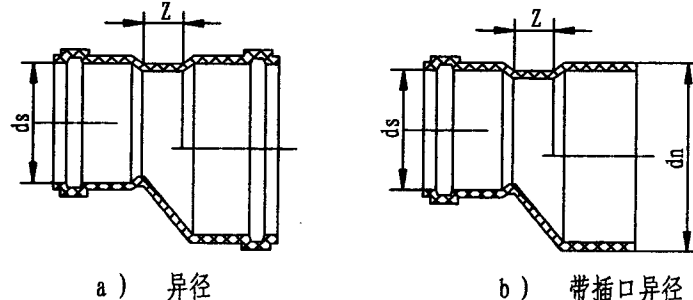
图6 异径
