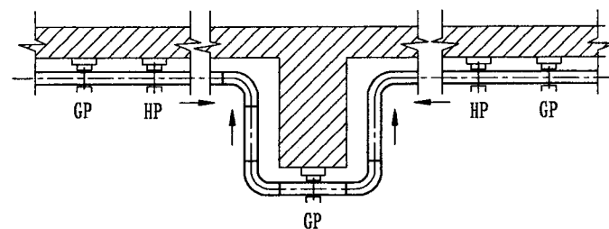
U形补偿
