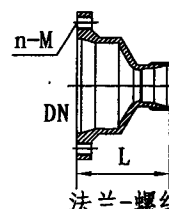
法兰-螺纹
