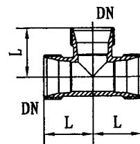
等径三通
