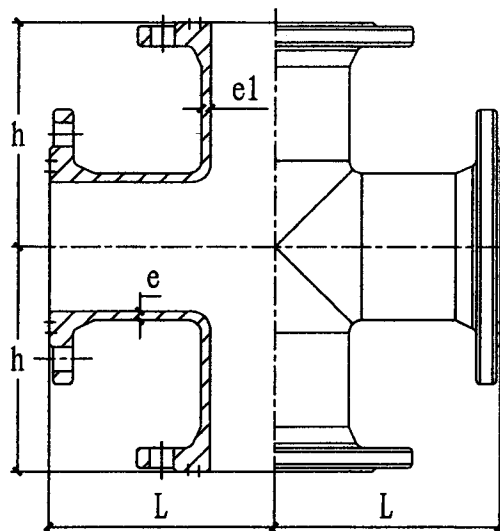
全盘四通管件
