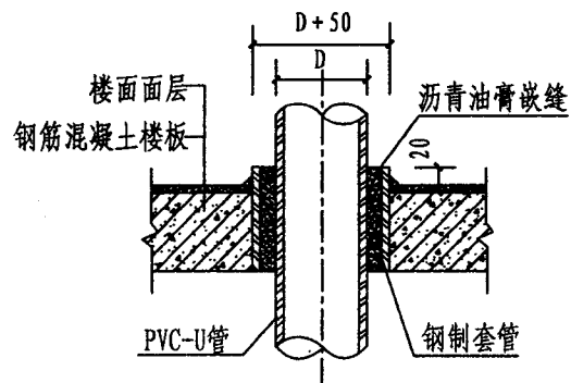
穿楼板 II
