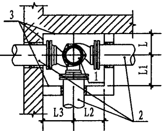
GYB4型
