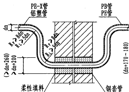
穿抗震、伸缩、沉降缝(二)
