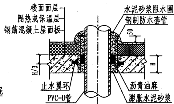
穿屋面板
