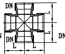
等径四通
