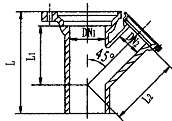
A型Y三通
