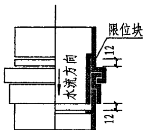
II 型伸缩节大样
