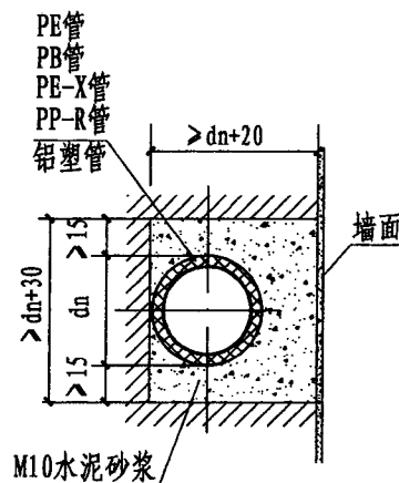
嵌墙安装
