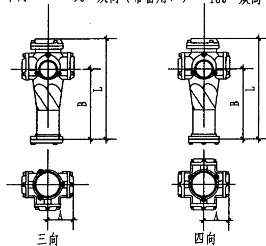
AD型细长接头
