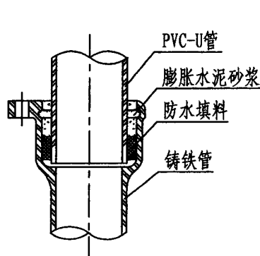
同径管
