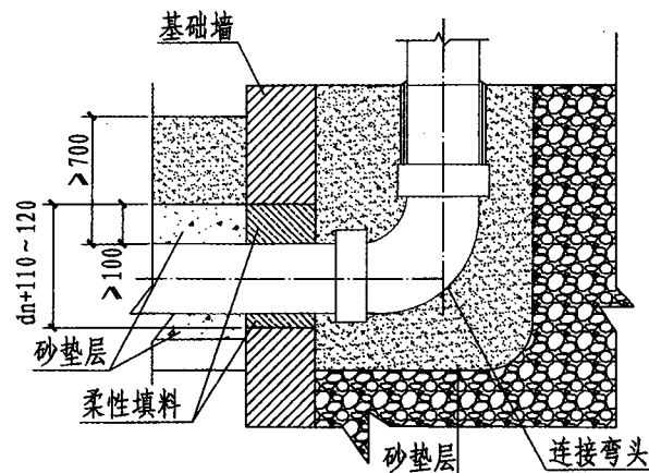
穿基础墙
