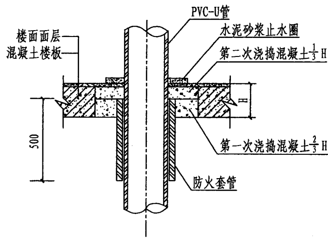
II型立管防火套管
