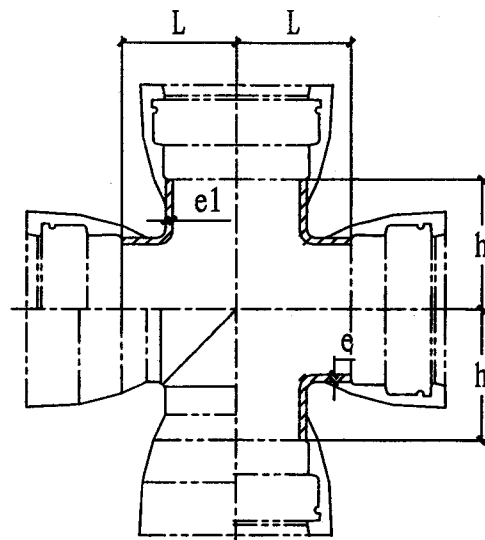
全承四通管件
