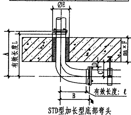
STD型加长型底部弯头规格尺寸 (mm)
