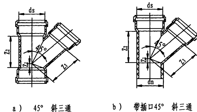
图3 45° 斜三通
