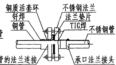
与铜管的法兰连接
