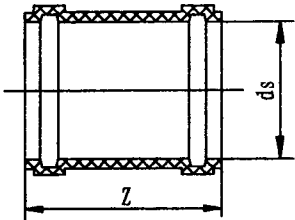
图7 直通
