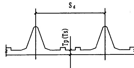
管肋大样图
