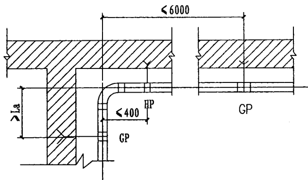
自由臂补偿
