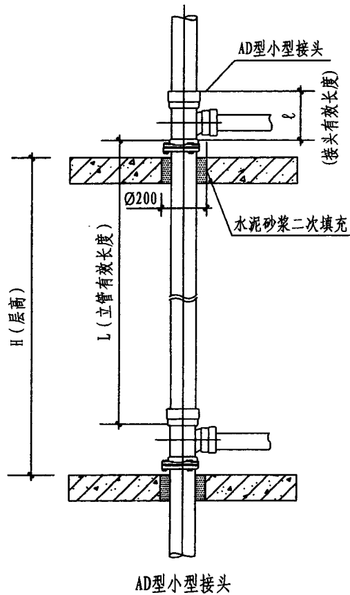
AD型小型接头规格尺寸 (mm)
