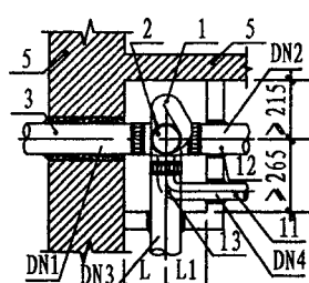
平面安装图II
