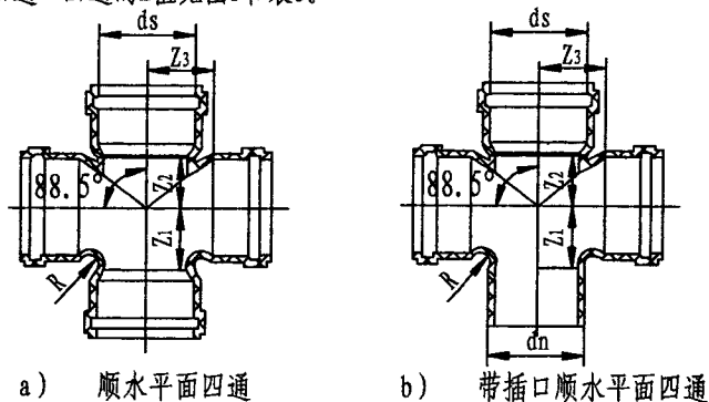
图5 顺水平面四通
