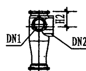
侧面图
