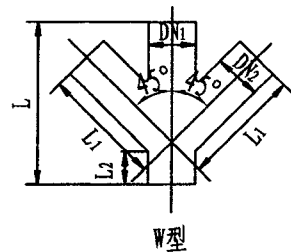
W型Y四通尺寸
