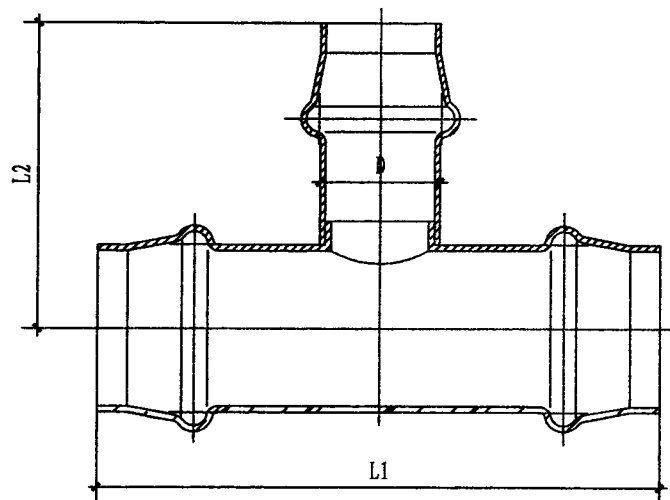
异径三通的基本尺寸 (单位: mm)
