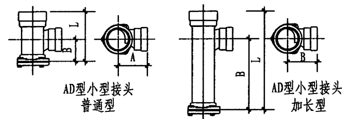
AD型小型接头规格尺寸 (mm)
