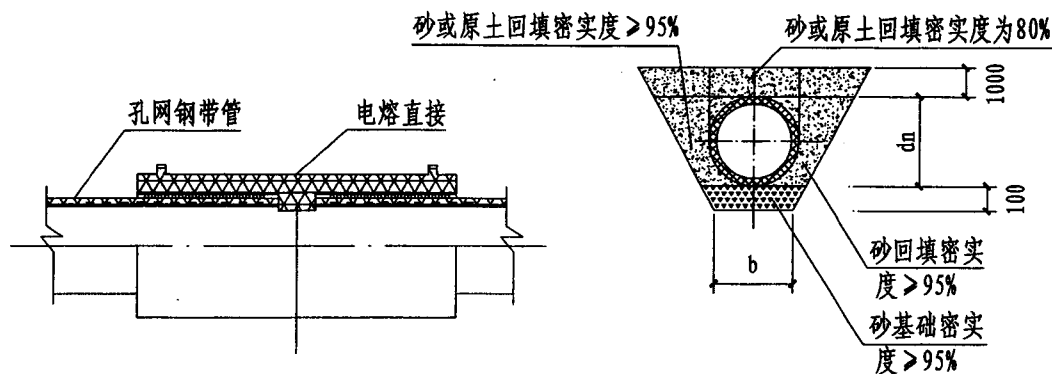
电熔直接连接
