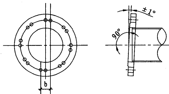
法兰面对钢管 轴线垂直度示意图
