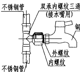
管件与附件连接
