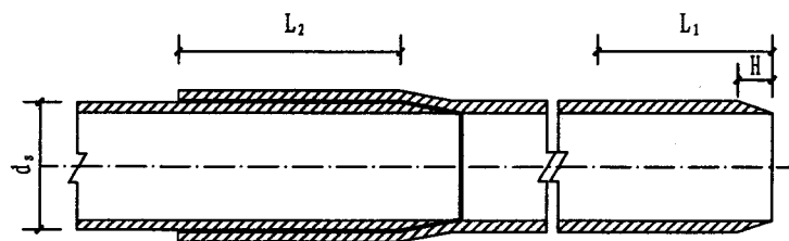
胶粘剂接口
