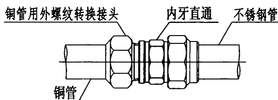
与铜管的螺纹连接
