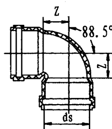
c) 90° 弯头
