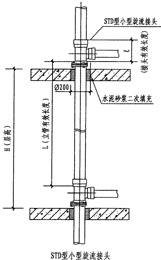
STD型小型旋流接头规格尺寸 (mm)
