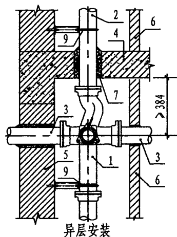
GY型旋流式铸铁苏维托特殊管件 (SVA系列、A型接口) 竖向安装图
