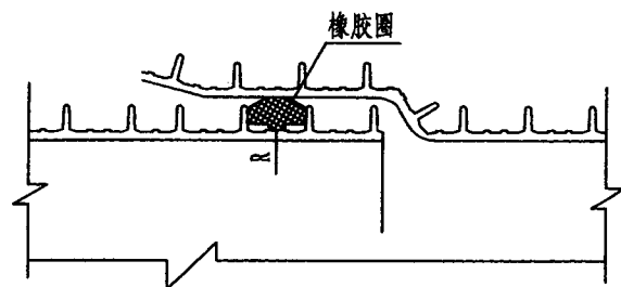
管道接口图
