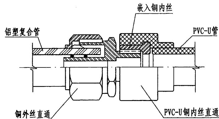
与铝塑复合管连接
