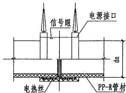
电熔连接
