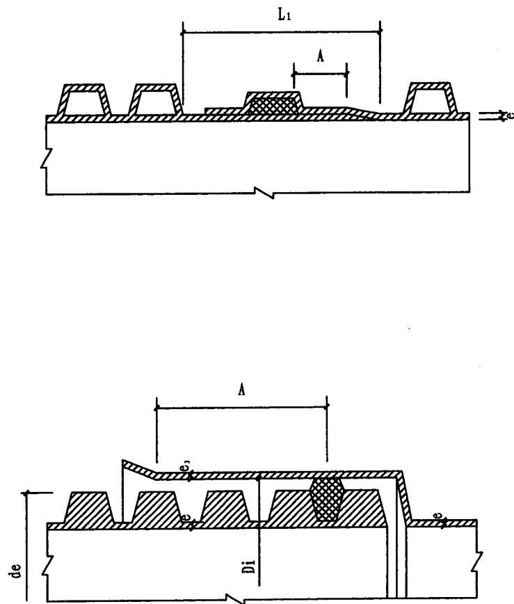
管材承插口
