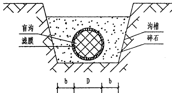
塑料盲沟施工回填图
