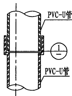
PVC-U承插管
