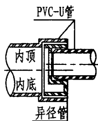
异径管横管安装
