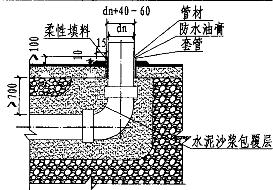
穿室内地面
