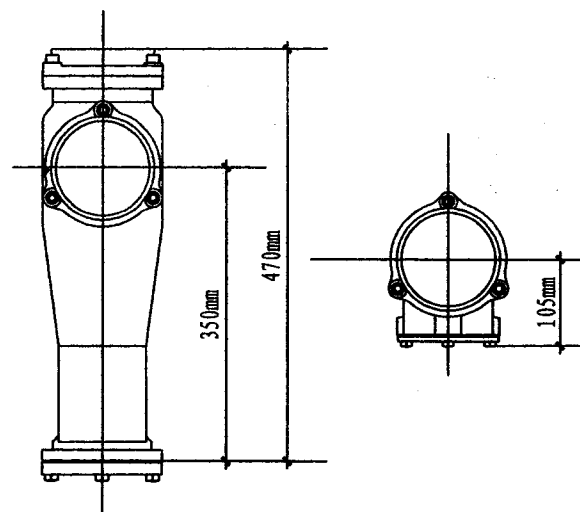
三通加强型接头 型号: C-5003
