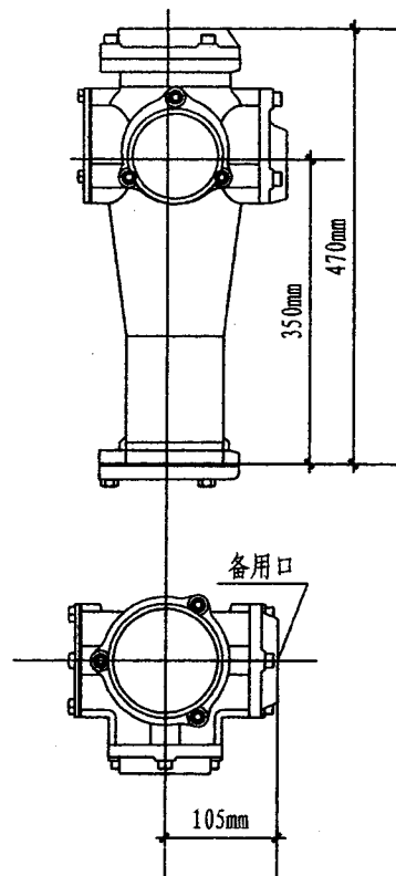
四通加强型接头 型号: C-5005A
