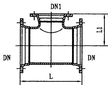
法兰-法兰 异径法兰三通
