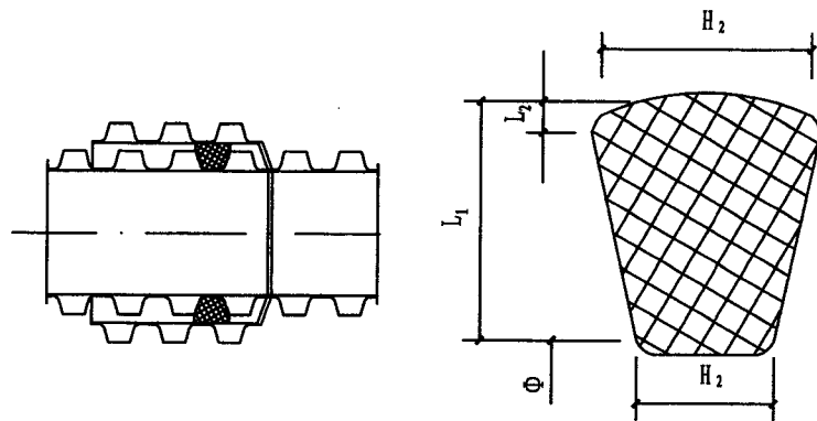
管道接口图
