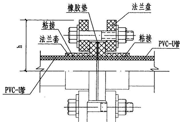
法兰连接
