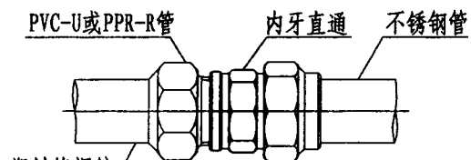
与塑料管的螺纹连接
