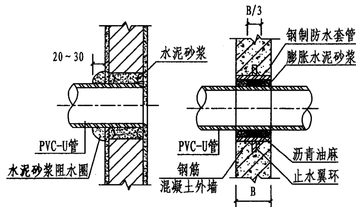
穿检查井壁
