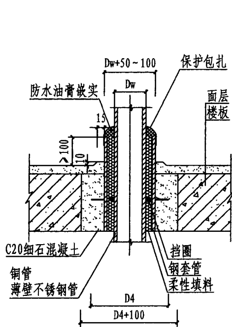
穿楼板 现浇刚性防水套管
