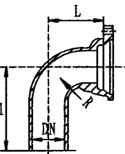
A型
