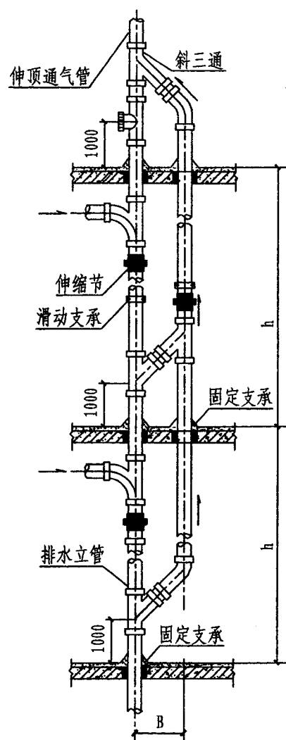
I 型
