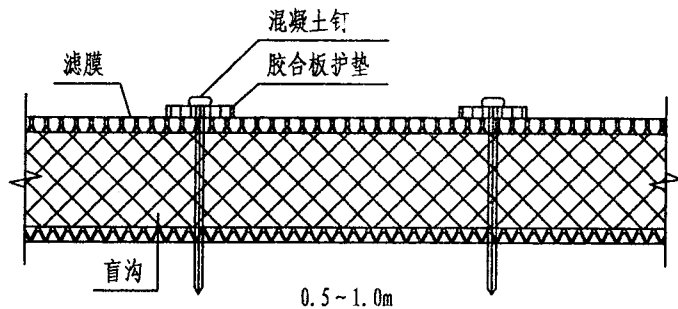
塑料盲沟与岩石体固定大样图
