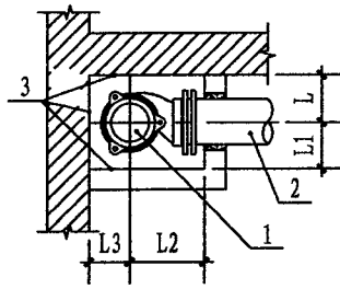
GYA4型
