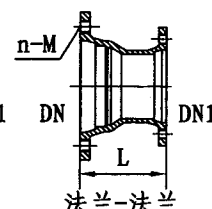
法兰异径直通
