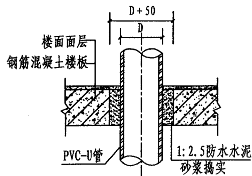
穿楼板 IV
