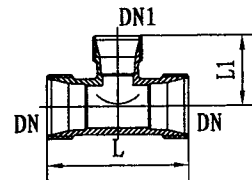
异径支流三通
