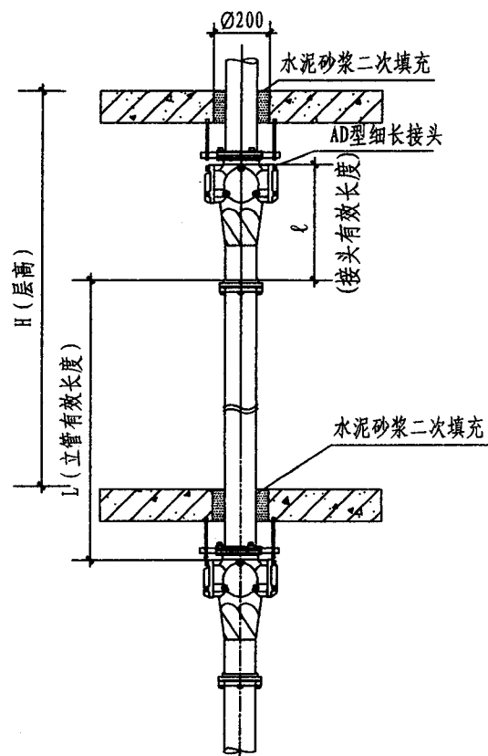
隔层安装
