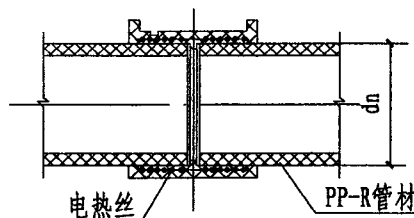
管道连接剖面
