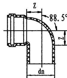
d) 带插口90° 弯头
