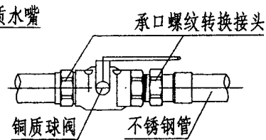
与球阀的螺纹连接(或活接球阀)
