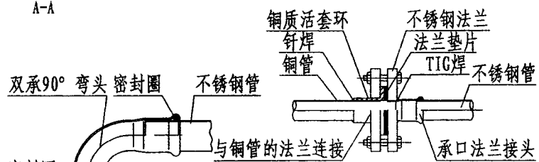
与铜管的法兰连接
