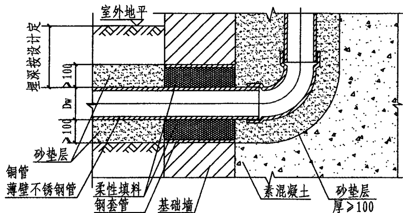
穿基础墙
