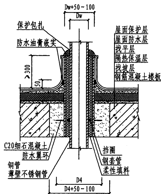
穿屋面(二) 现浇刚性防水套管
