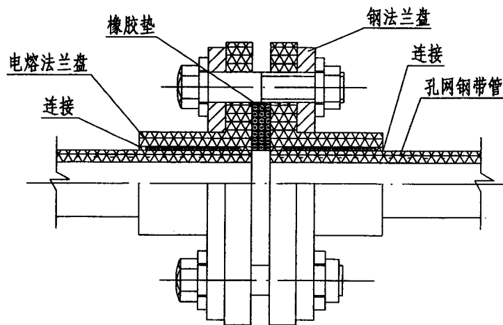
法兰连接
