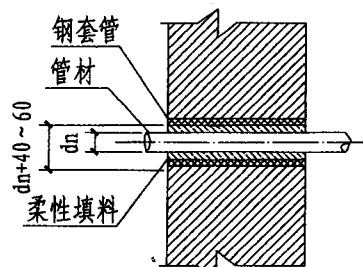
穿内墙
