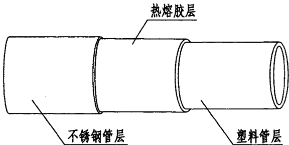
不锈钢塑料复合管结构图
