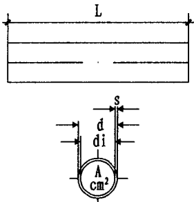
双层(双色)高密度聚乙烯(HDPE)管道
