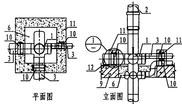
苏维托穿越楼板安装防水措施
