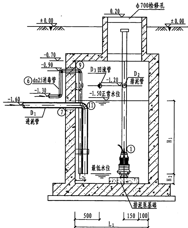
I-I 剖面图
