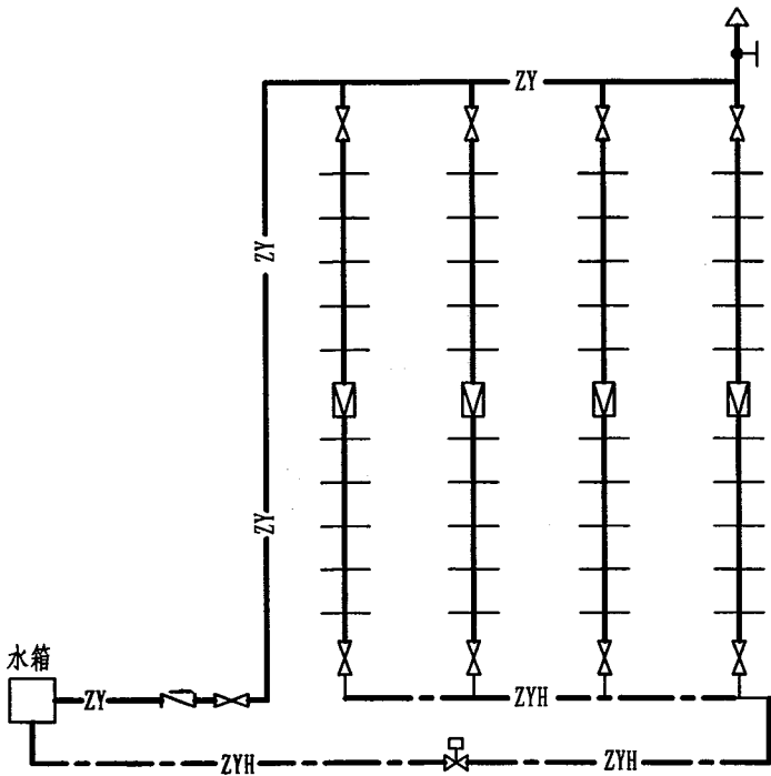
适用于高度小于50m、立管数较少的建筑物 (低区亦可用支管可调式减压阀)
