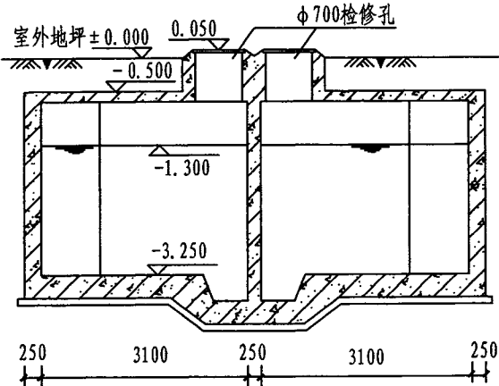
II-II 剖面图
