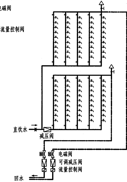
直饮水供水系统原理示意图
