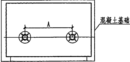
平面
