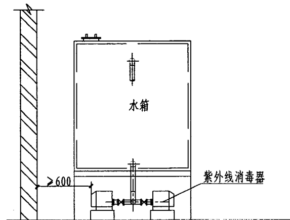
II-II 剖面图
