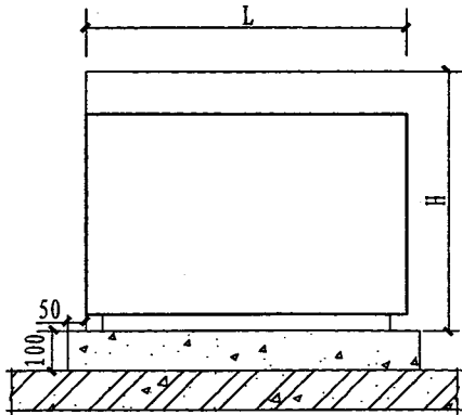
立面
