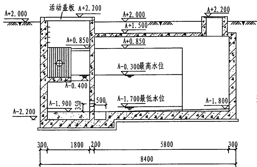
I-I 剖面图
