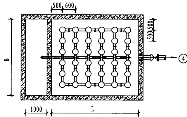
底层平面图
