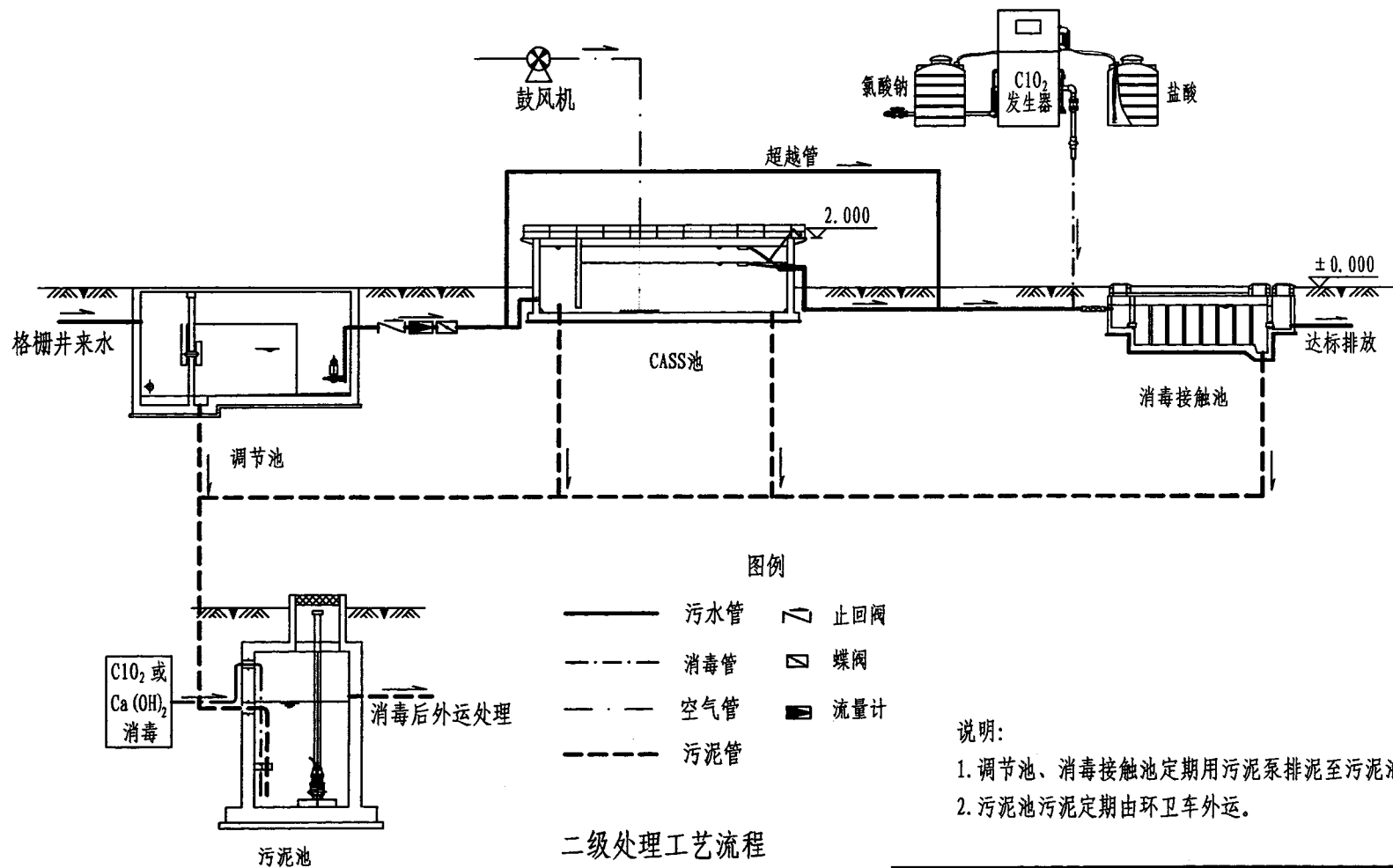
二级处理工艺流程 (三)
