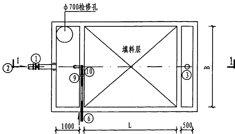
顶层平面图
