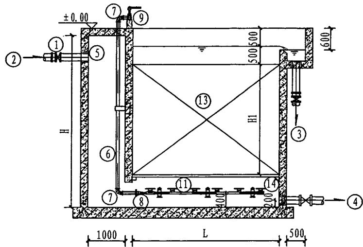
I-I 剖面图
