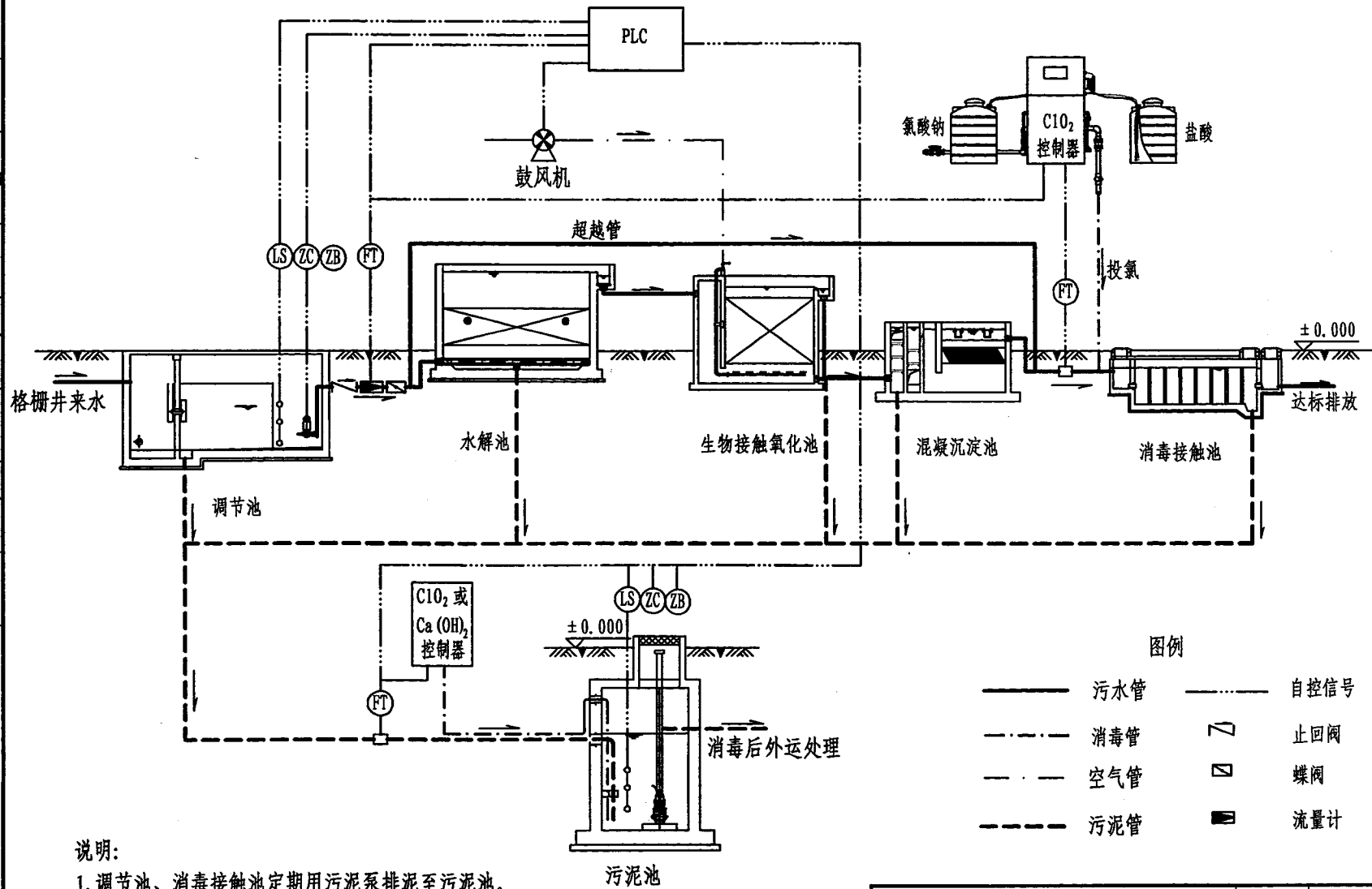
二级处理监测流程图
