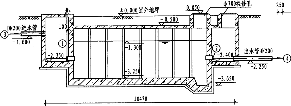
I-I 剖面图
