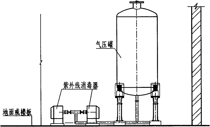
II-II 剖面图
