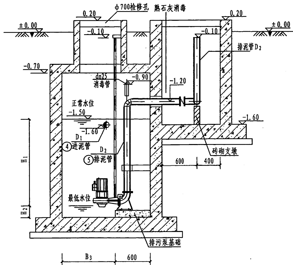
II-II 剖面图
