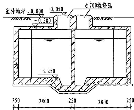
II-II 剖面图
