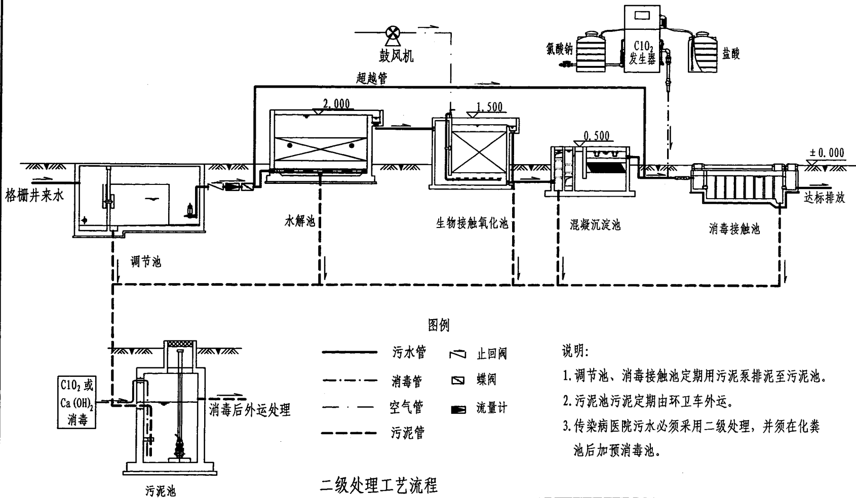
二级处理工艺流程 (一)
