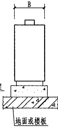
侧面
