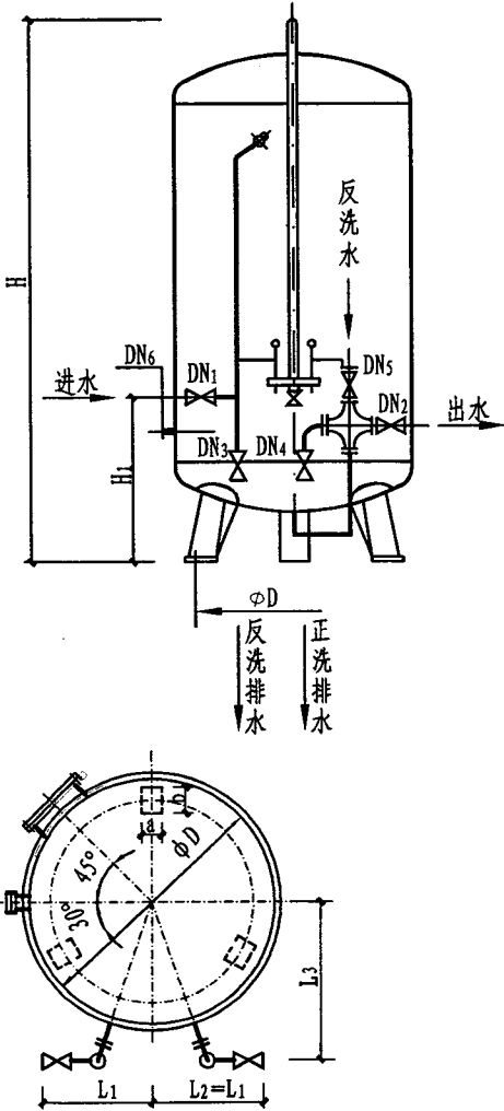
活性炭过滤器
