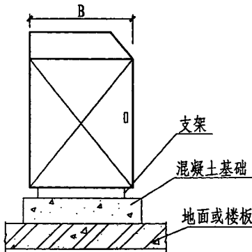
侧面
