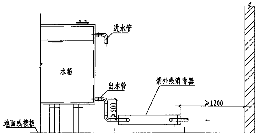
I-I 剖面图
