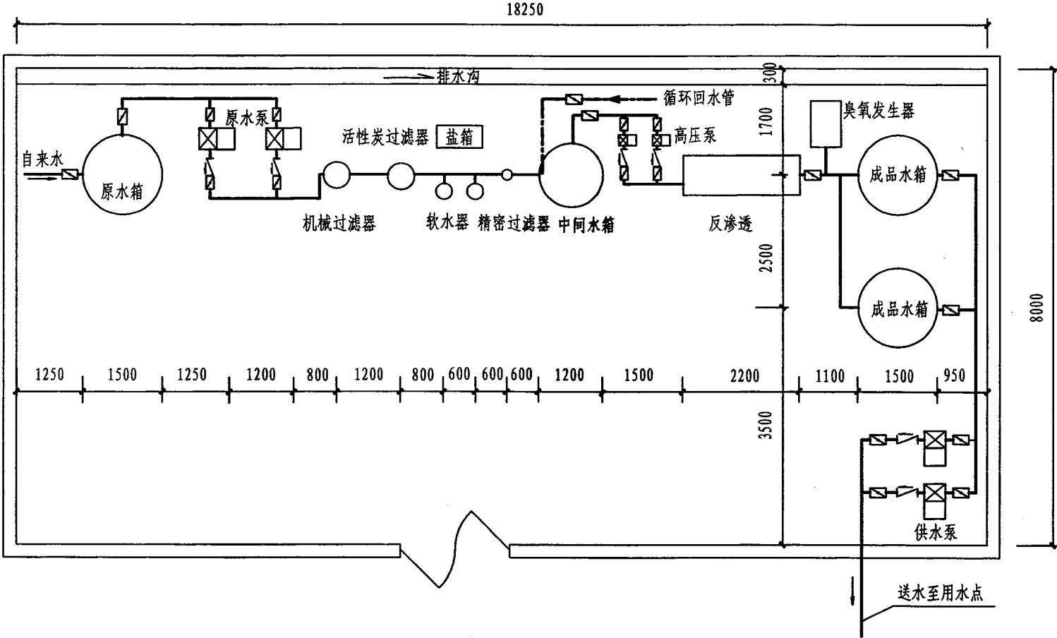
平面布置图
