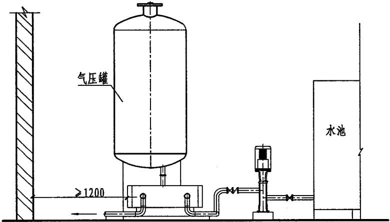
I-I 剖面图
