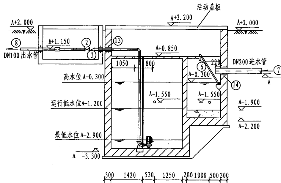
III-III 剖面图
