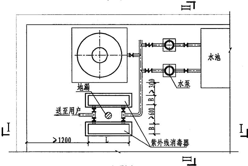
平面图
