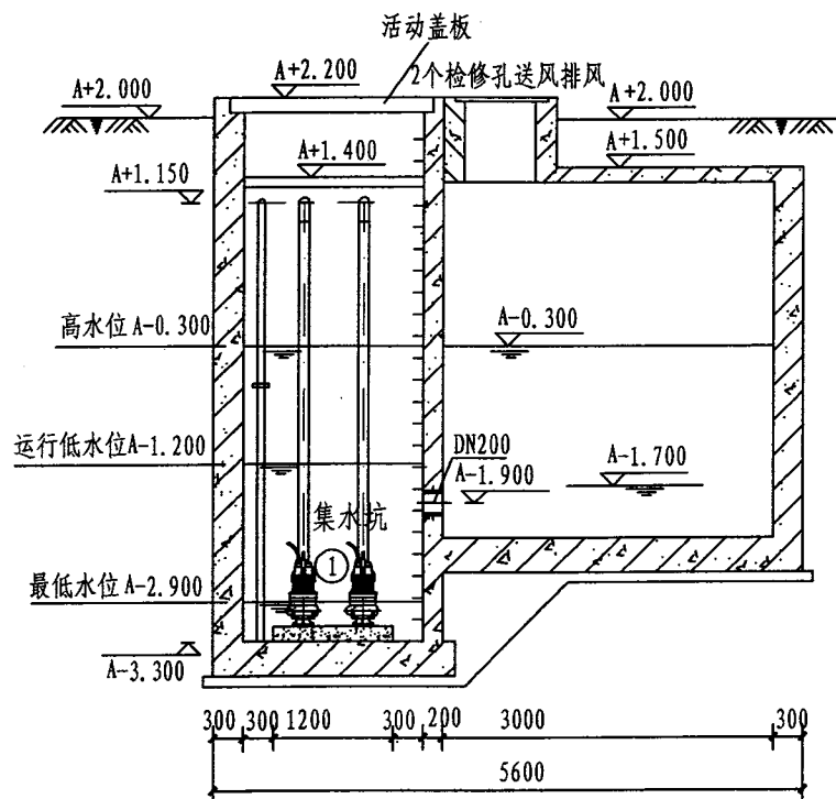
II-II 剖面图
