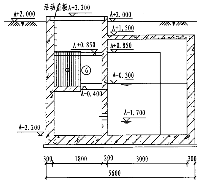
I-I 剖面图
