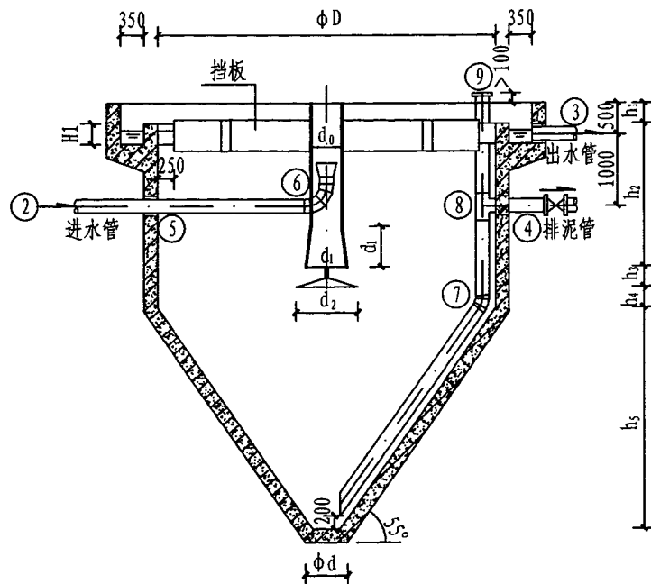
I-I 剖面图
