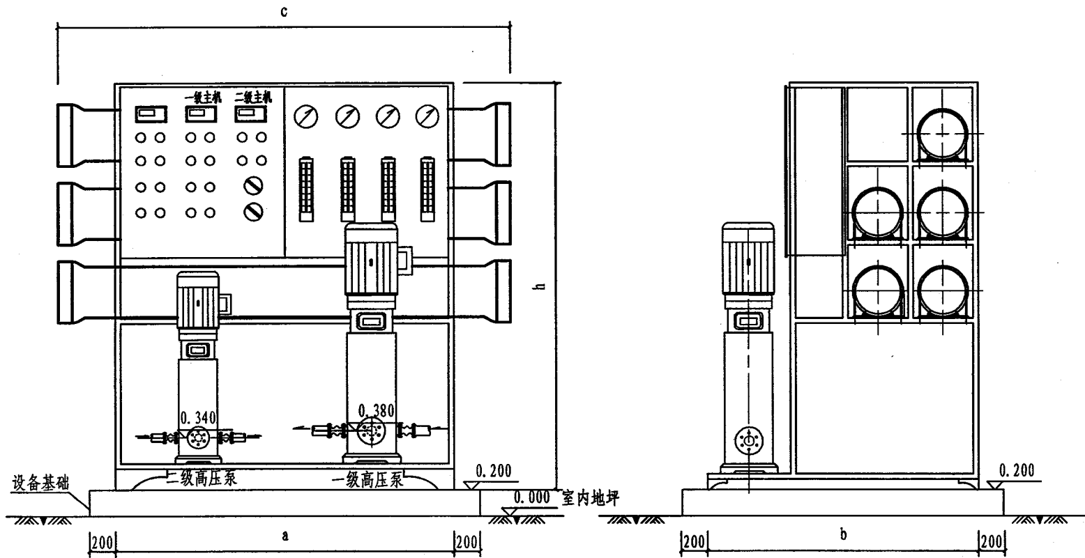
R0主机正视图
