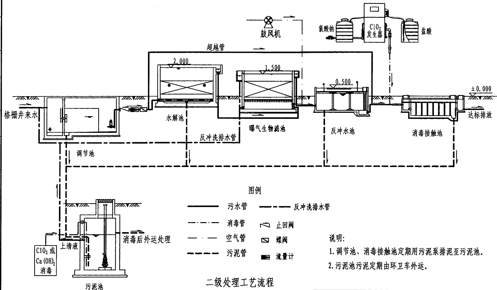
二级处理工艺流程 (二)
