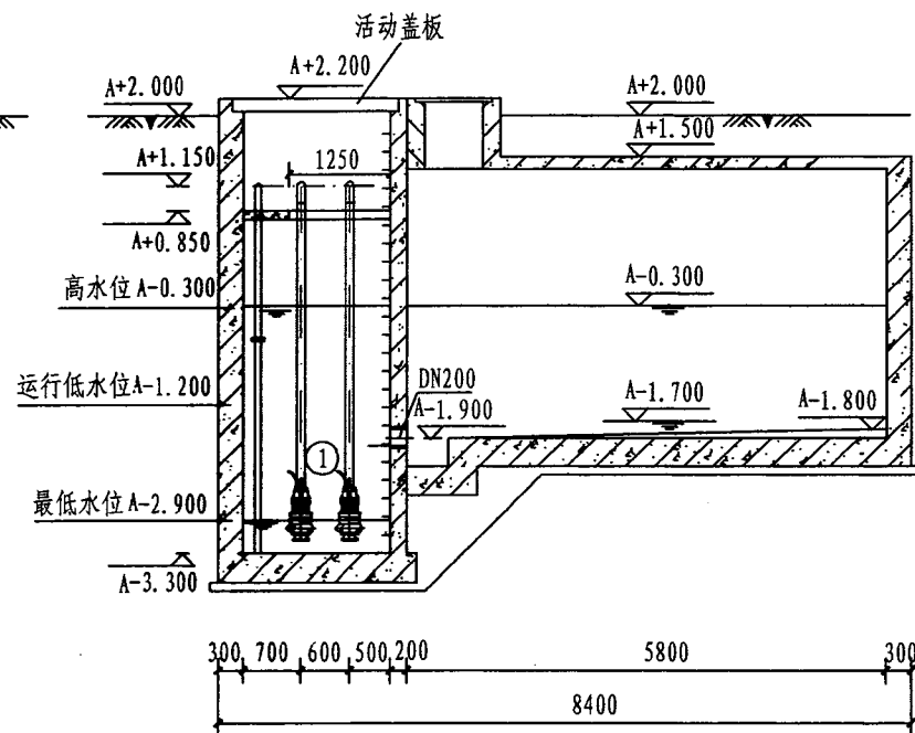
II-II 剖面图
