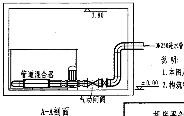
机房平剖面布置图
