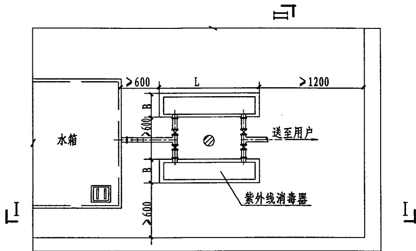
平面图
