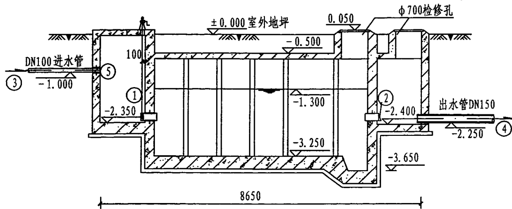
I-I 剖面图
