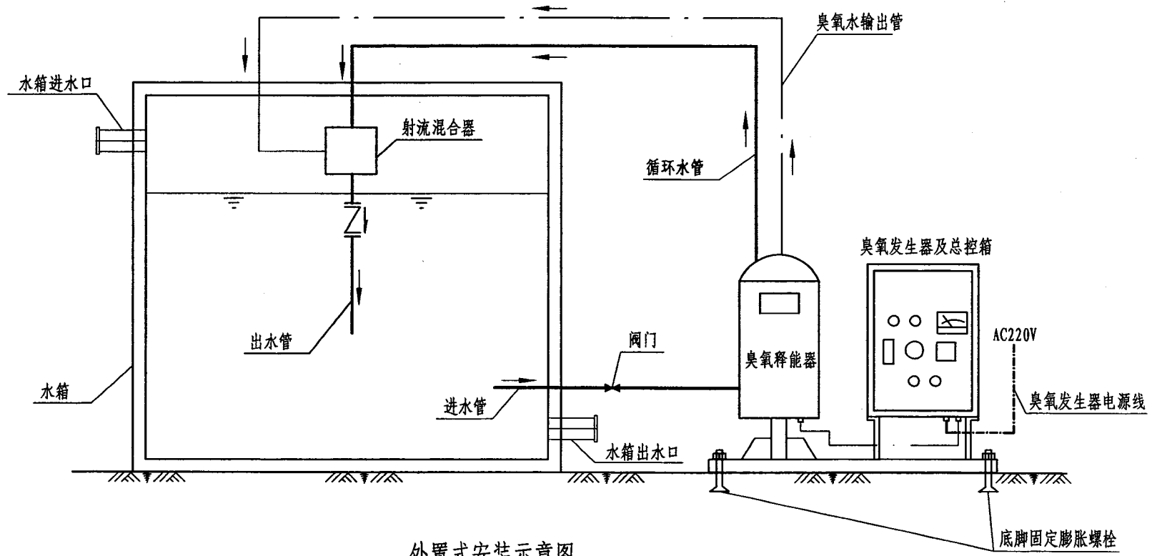
外置式安装示意图
