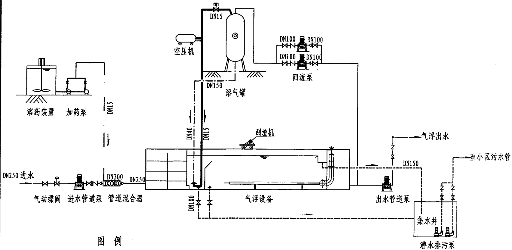
工艺流程图
