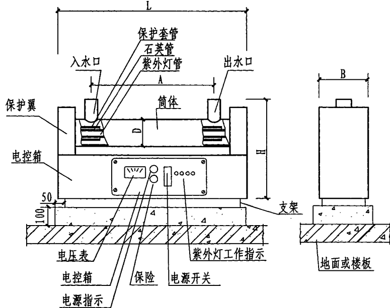
立面
