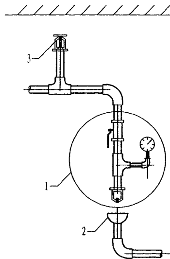
末端试水装置安装图
