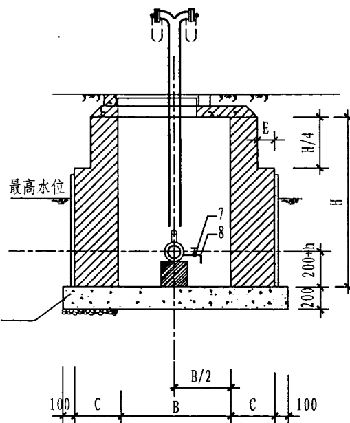
B-B剖面图
