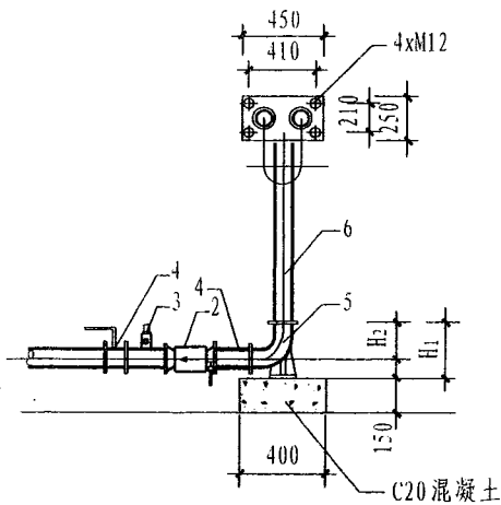
A-A剖面图
