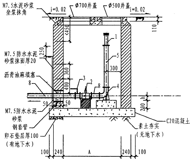
A-A剖面图
