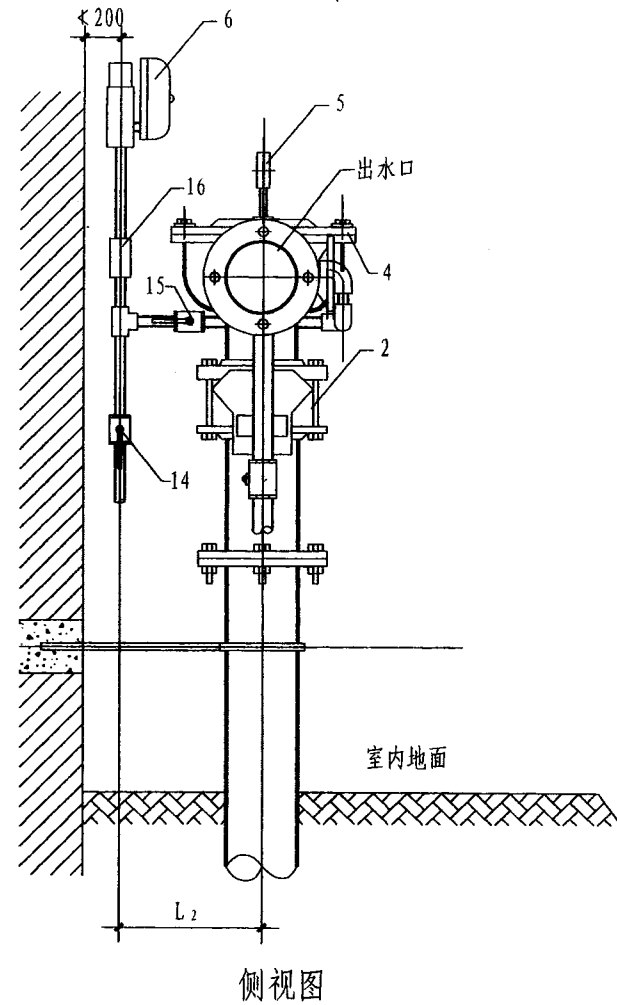
ZSFM系列雨淋自动喷水 报警装置安装图(一)
