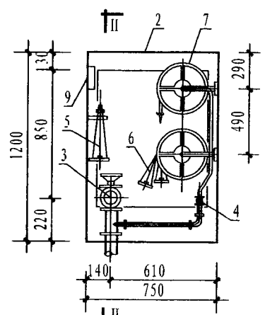
I-I 剖面图
