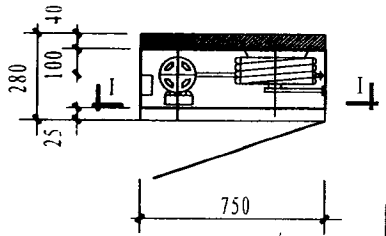
平面图
