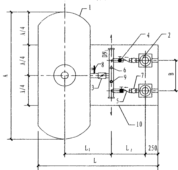
平面图
