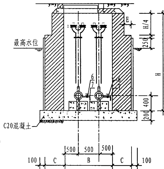
B-B剖面图
