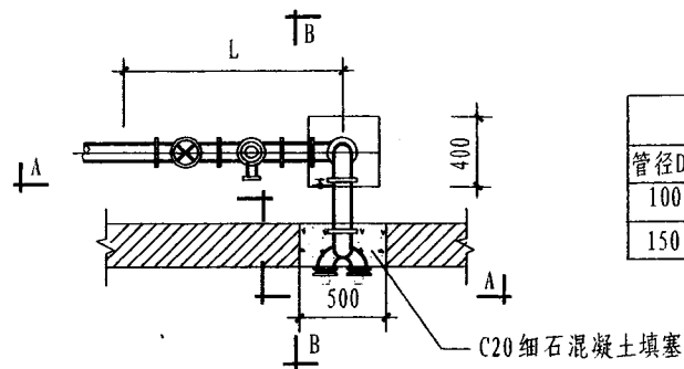
甲型平面图
