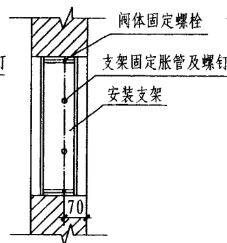
FXY-III 型泄压阀支架安装图
