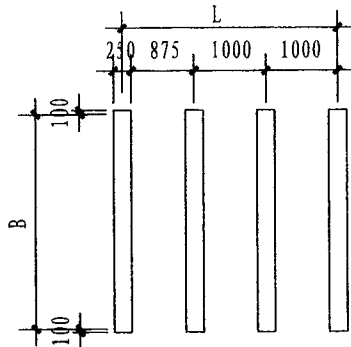
侧立面图
