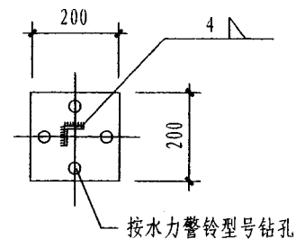
I - I 剖面图
