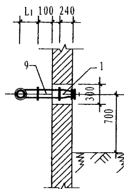
B-B剖面图
