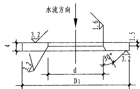
倒角扩口型减压孔板
