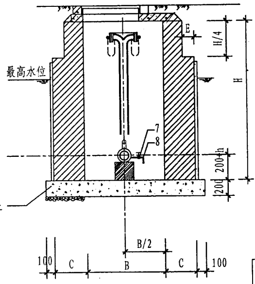
B-B剖面图
