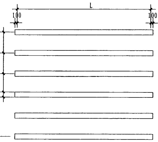
水箱基础平面图
