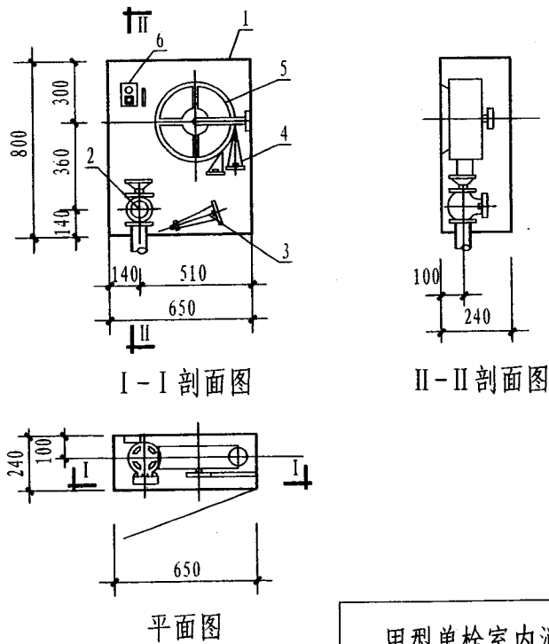
甲型单栓室内消火栓箱
