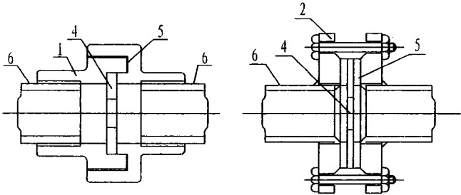
孔板安装在活接头中
