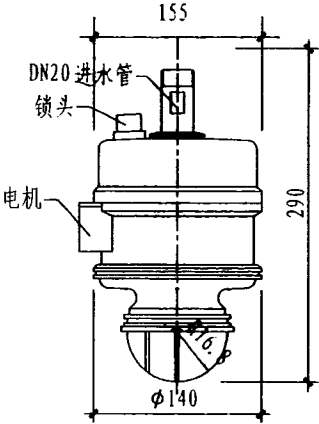
ZSS-20型灭火装置 外形尺寸图(单位mm)
