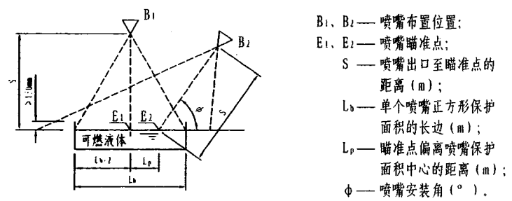
架空型喷嘴的布置方法
