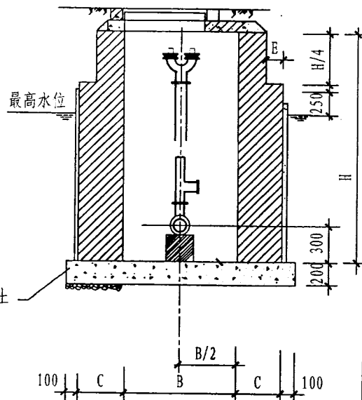
B-B剖面图
