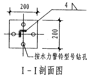
水力警铃支架大样图
