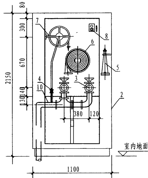
双栓带消防 软管卷盘组合式消防柜
