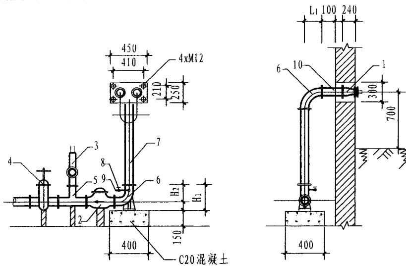
A-A剖面图
