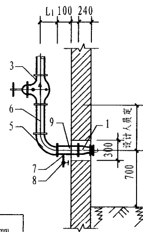
丙型安装图
