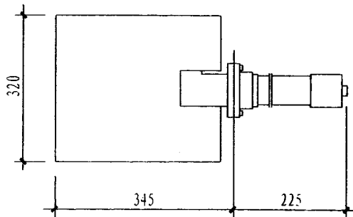
平面图
