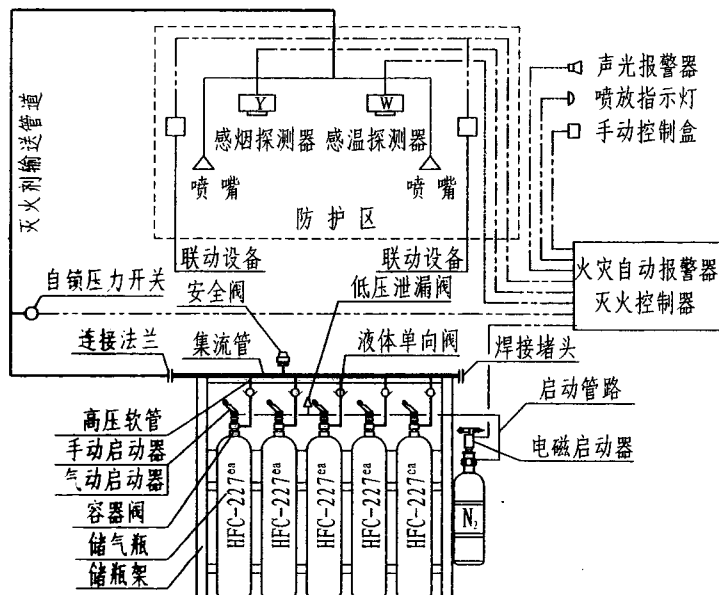
七氟丙烷单元独立系统原理图 (氮气驱动)
