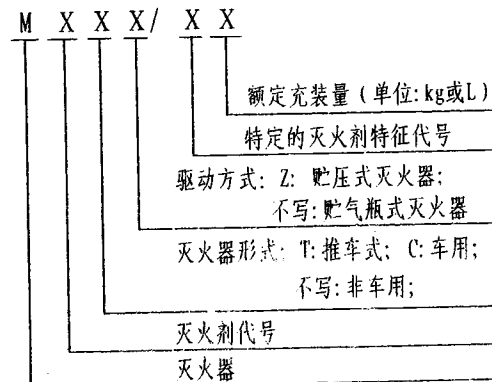
灭火器灭火剂代号和特定灭火剂特征代号表
