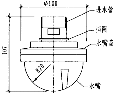
ZSD-40A型灭火装置 外形尺寸图(单位mm)
