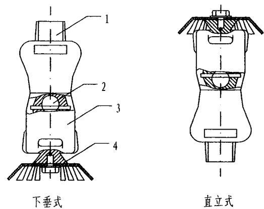
三、PT系列空气泡沫喷头结构图
