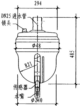
ZSS-25型灭火装置 外形尺寸图(单位mm)
