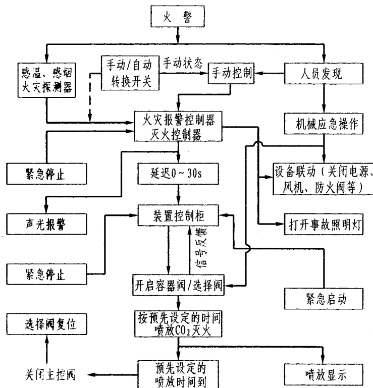
低压CO 2 灭火系统动作程序图
