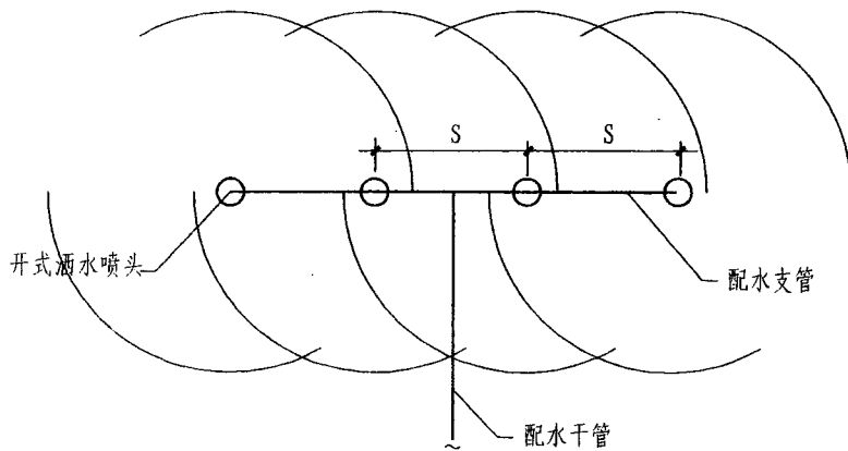
开式洒水喷头防护冷却水幕布置图
