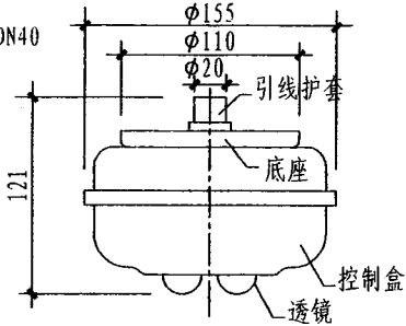
ZSD-40A型灭火装置控制器 外形尺寸图(单位mm)
