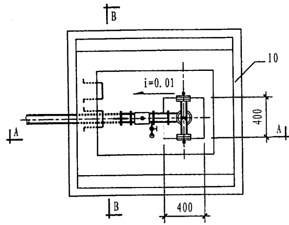
平面图
