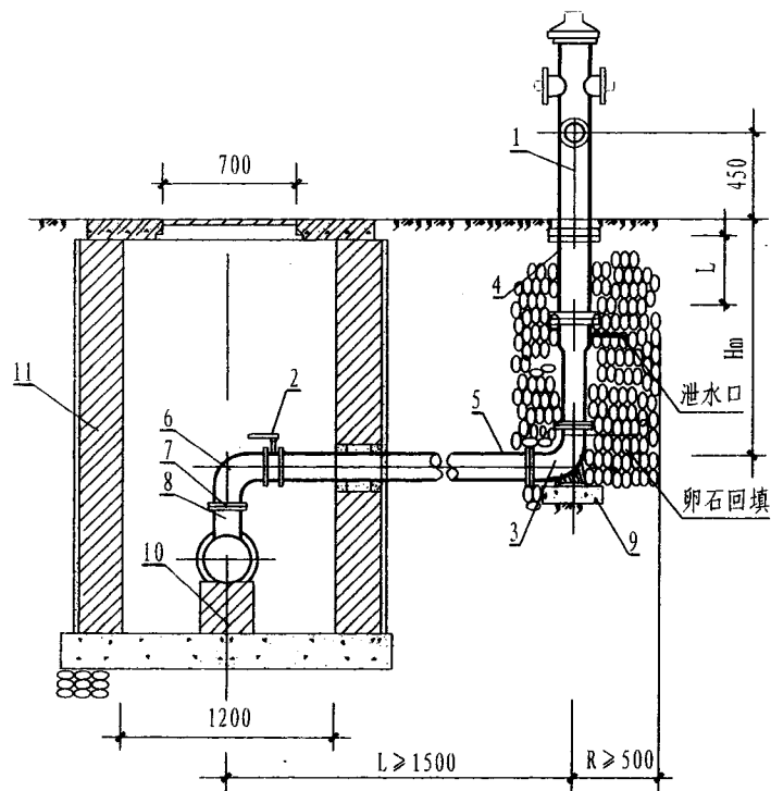
1-1 剖面图
