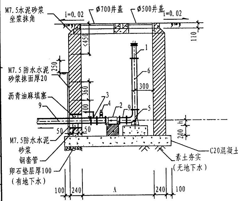
A-A剖面图
