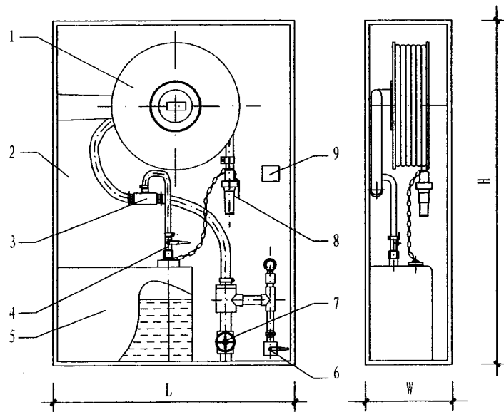
结构图
