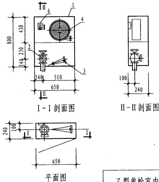
乙型单栓室内消火栓箱
