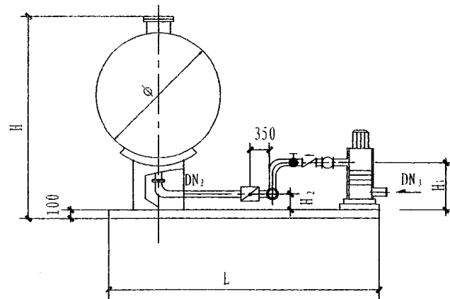
立视图
