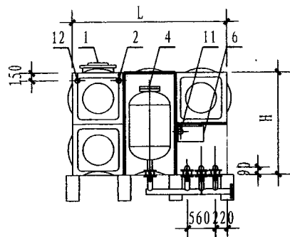
正立面图
