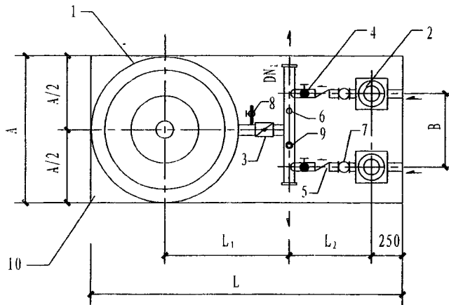
平面图
