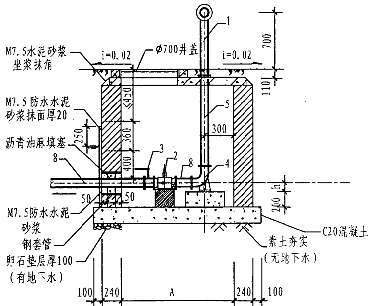
A-A剖面图
