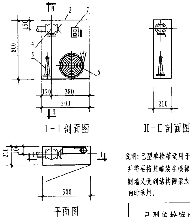
己型单栓室内消火栓箱
