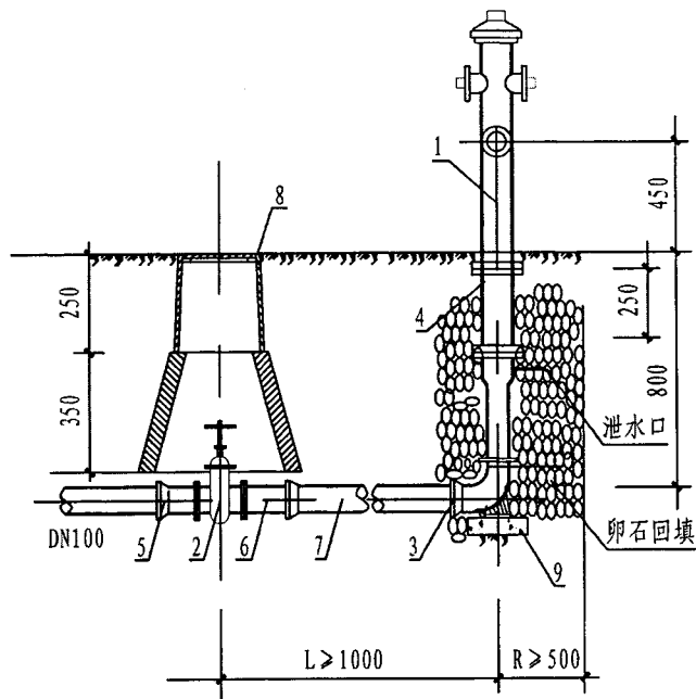
1-1 剖面图
