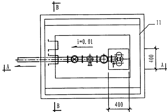
平面图
