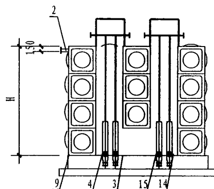
侧立面图
