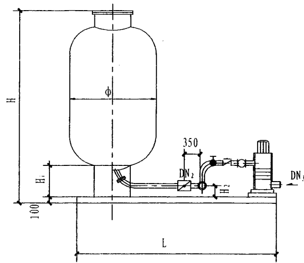
立视图
