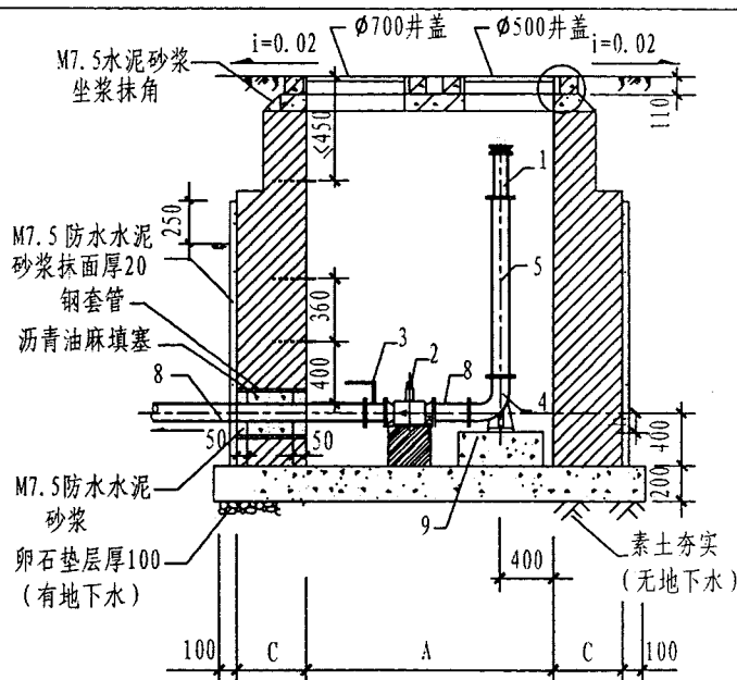
A-A剖面图
