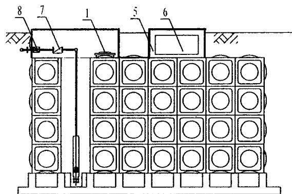
正立面图
