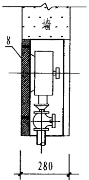
II-II 剖面图
