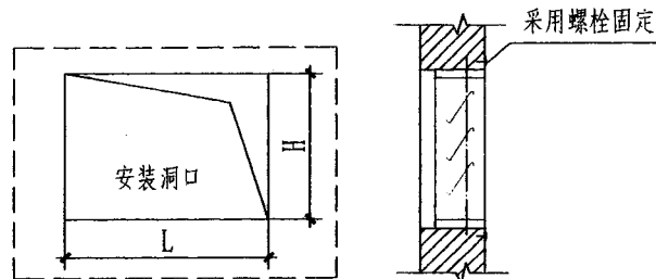
机械式开启泄压阀安装图
