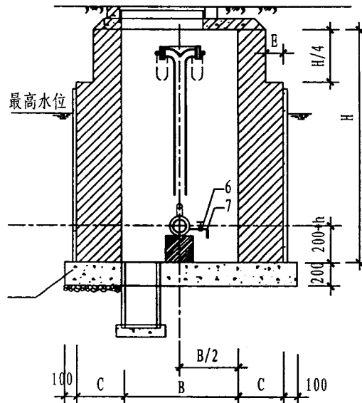
B-B剖面图
