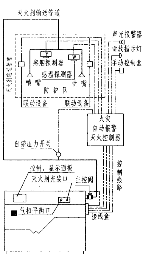
单元独立系统原理图
