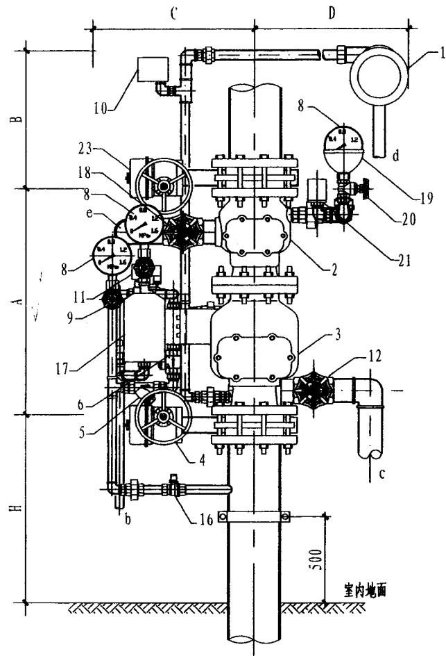
正视图
