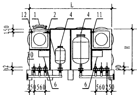
正立面图
