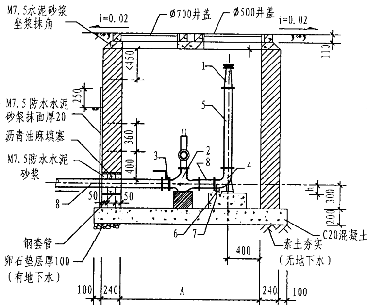
A-A剖面图
