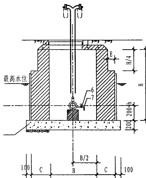
B-B剖面图
