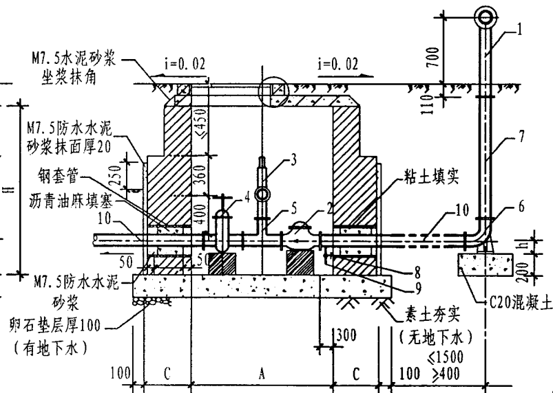
B-B剖面图
