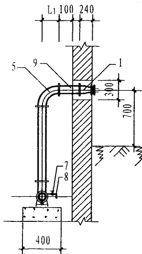
B-B剖面图
