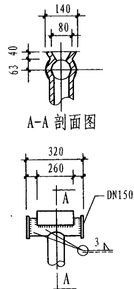
排水漏斗节点详图
