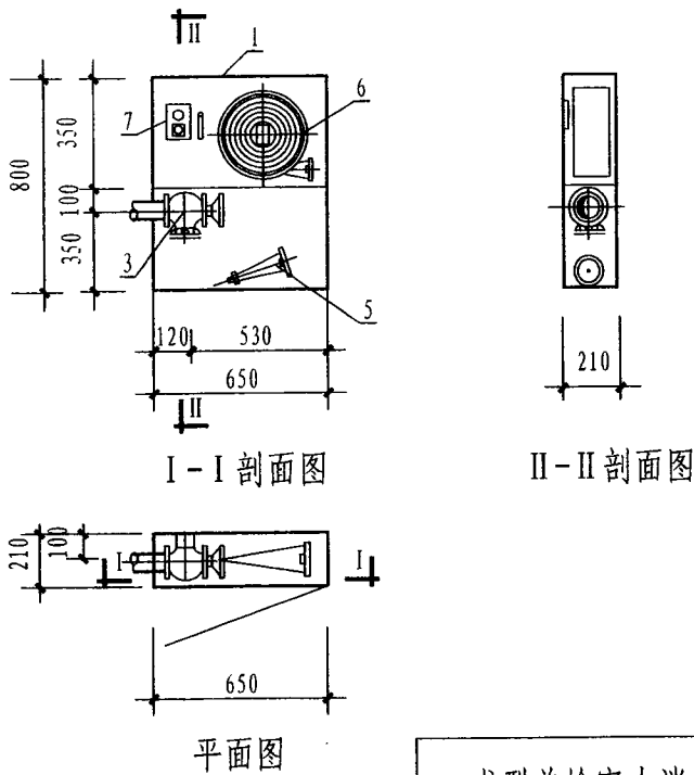
戊型单栓室内消火栓箱
