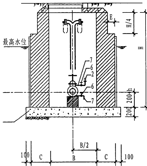
B-B剖面图
