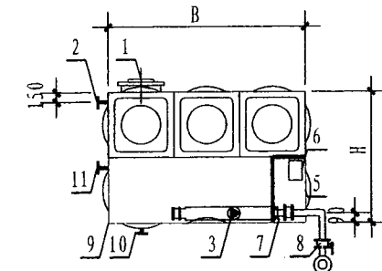
侧立面图
