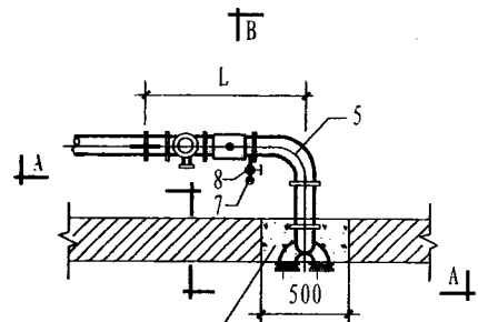
乙型平面图
