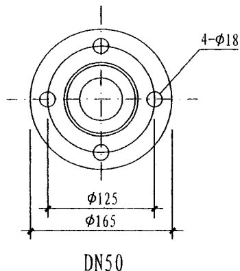
DN50 入口法兰外形尺寸图
