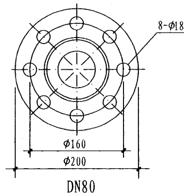
DN80 入口法兰外形尺寸图
