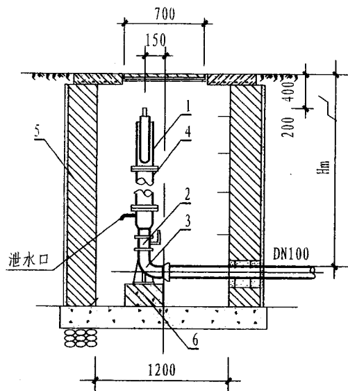
1-1 剖面图
