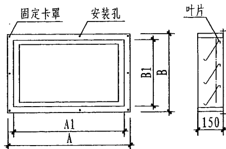
XYK系列机械式开启泄压阀外形图
