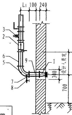
丙型安装图
