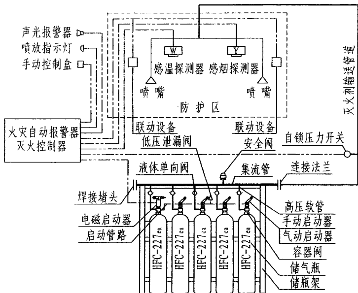
七氟丙烷单元独立系统原理图 (灭火剂自身驱动)
