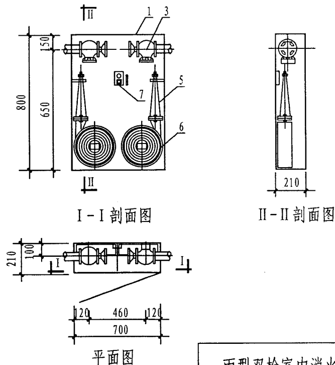
丙型双栓室内消火栓箱
