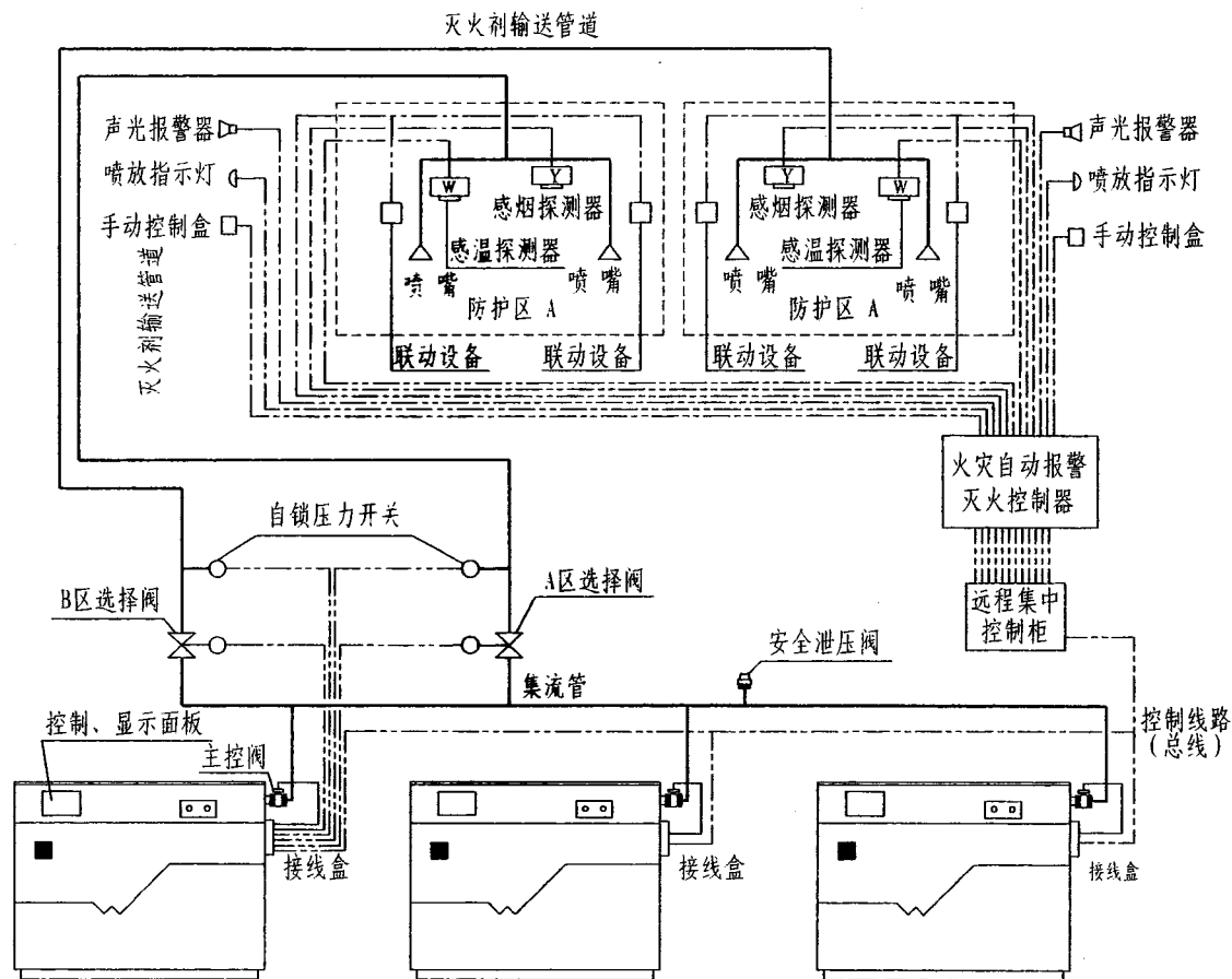
组合分配系统原理图
