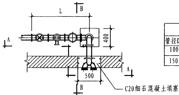
甲型平面图
