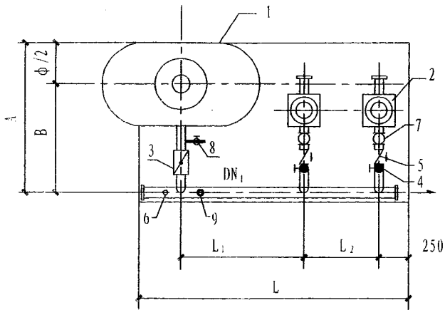
平面图
