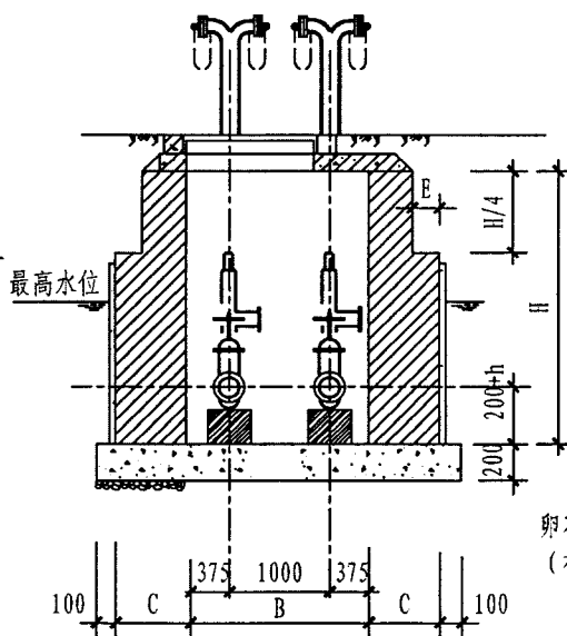
A-A剖面图
