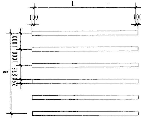
水箱基础平面图
