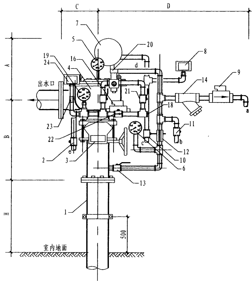
正视图
