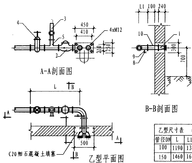
乙型平面图
