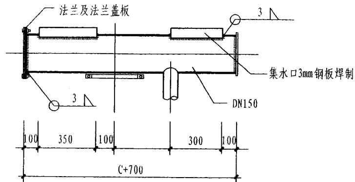
正视图
