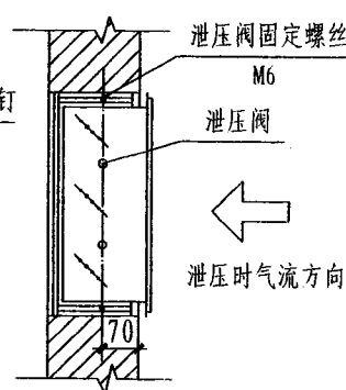
泄压阀安装图 (以FXY-III型为例)
