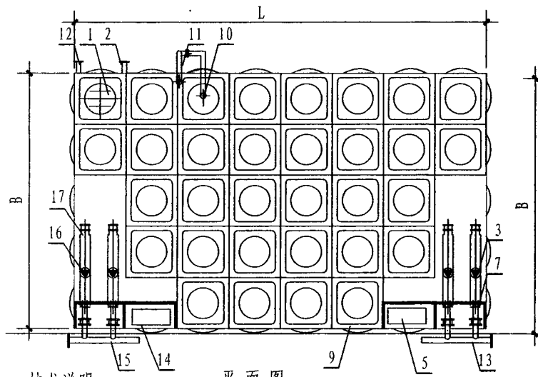
平面图
