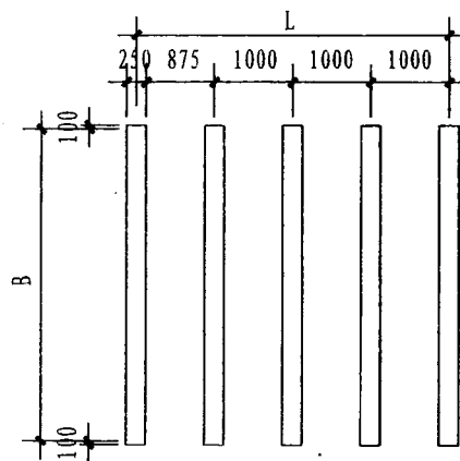
②侧立面图
