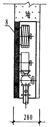
II-II 剖面图
