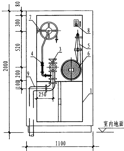
单栓带消防 软管卷盘组合式消防柜
