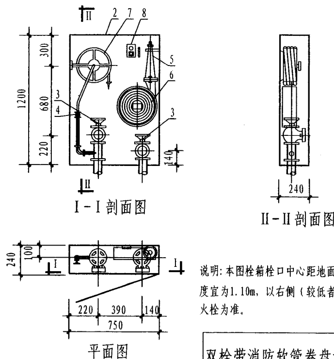
单栓带消防软管卷盘灭火栓箱
