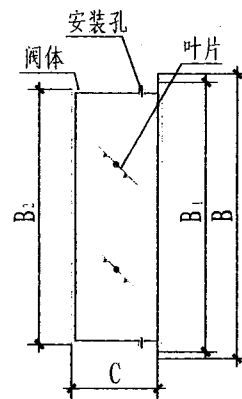
FXY-I (II) WLZX-013(025) 型剖面图
