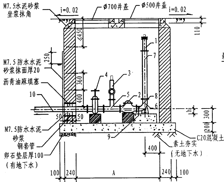
A-A剖面图
