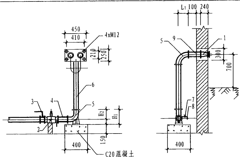
A-A剖面图
