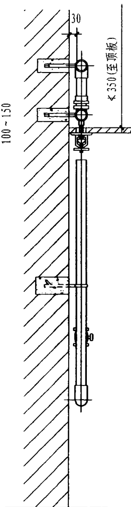
A-A剖面图
