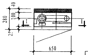
平面图
