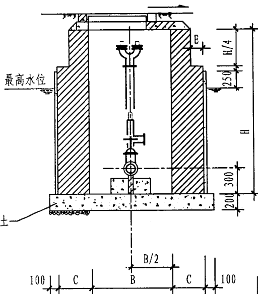
B-B剖面图
