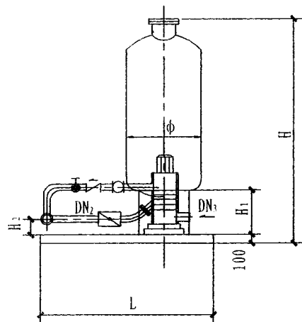
右立式图
