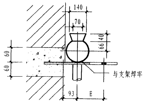
侧视图
