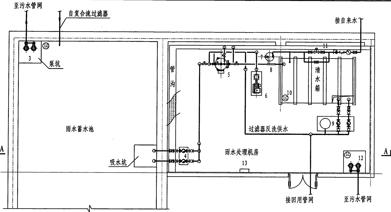
雨水（过滤）处理系统平面图
