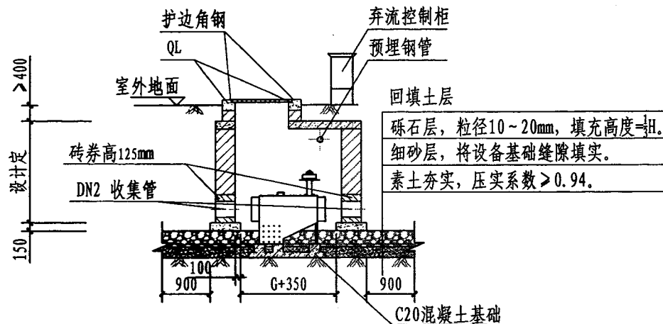
3-3剖面图 (做法I)
