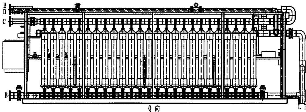
设备后视图
