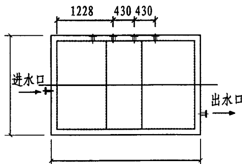
III型设备俯视图
