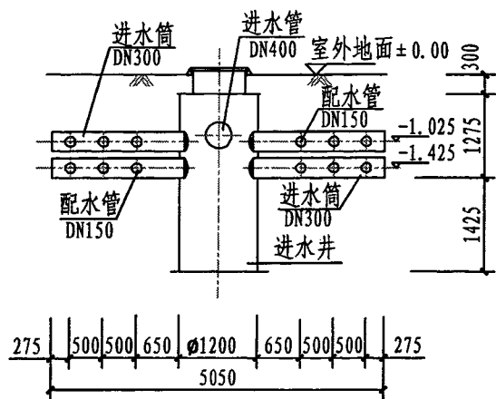
3-3剖面图
