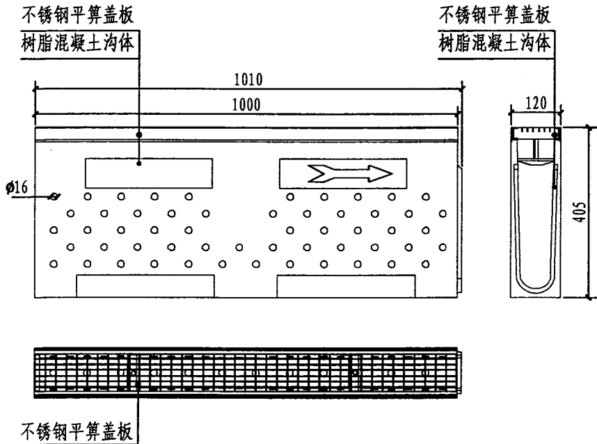
渗透式树脂混凝土排水沟示意图
