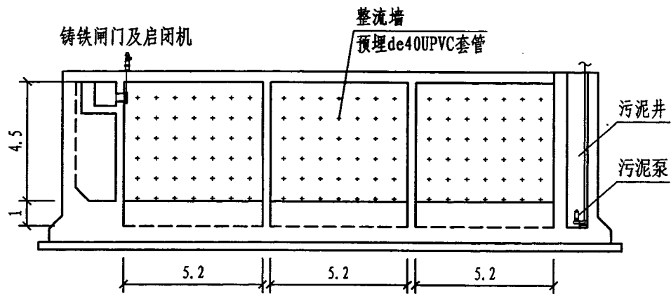
D-D剖面图
