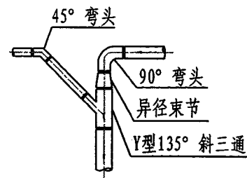
两条悬吊管接入同一立管大样图
