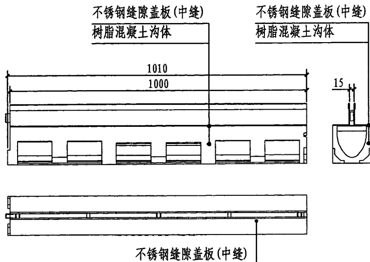
中缝缝隙式排水沟示意图
