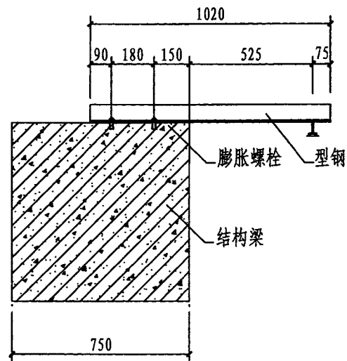
固定大样图
