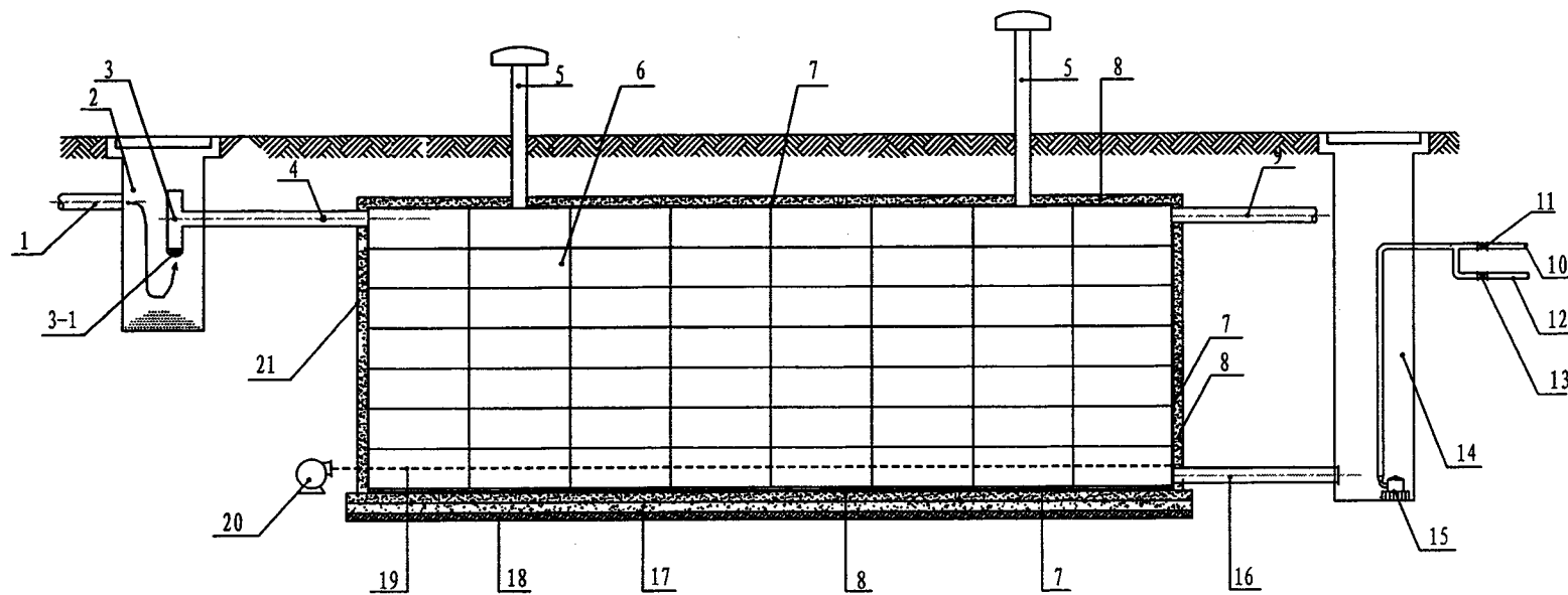
塑料模块蓄水池安装示意图
