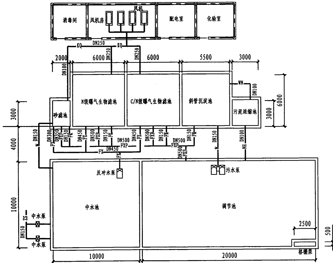
曝气生物滤池工艺管线平面图 (50m³/h)
