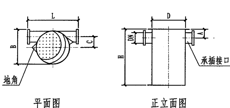
复合流过滤器外形图
