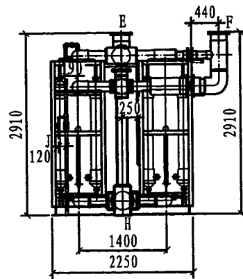
设备左视图
