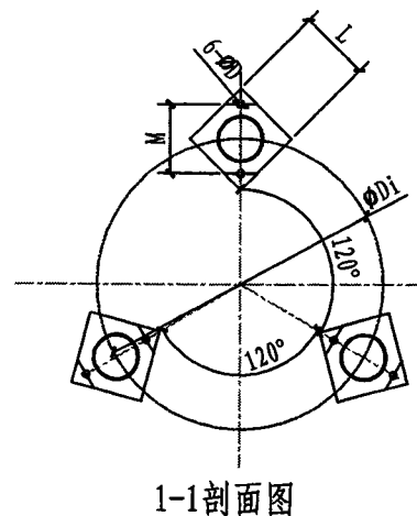
混凝反应器外形及基础尺寸图
