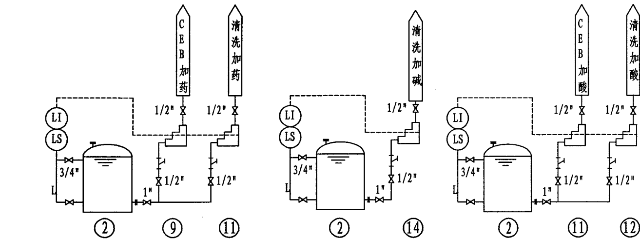
超滤加药系统图
