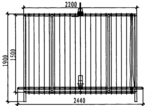
正视图
