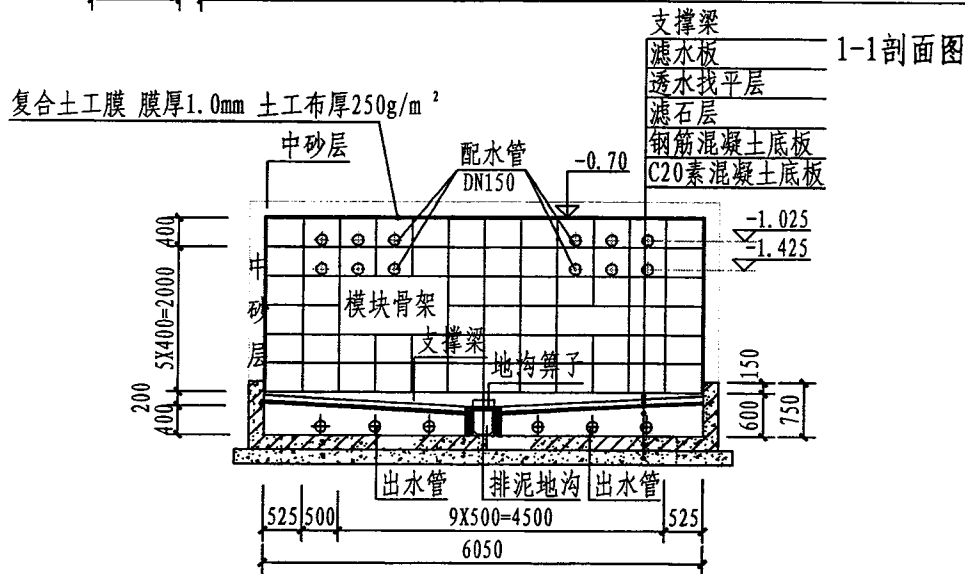
2-2剖面图
