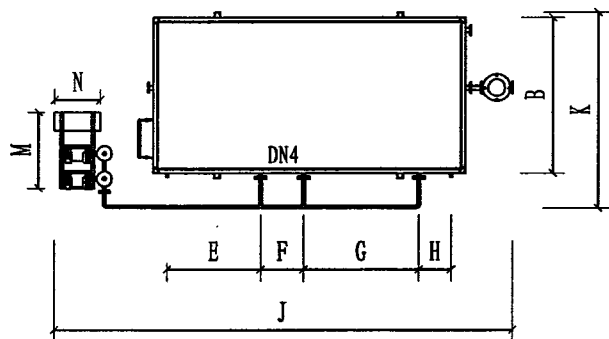
II型设备俯视图
