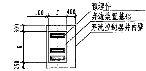
弃流控制器基础平面定位图
