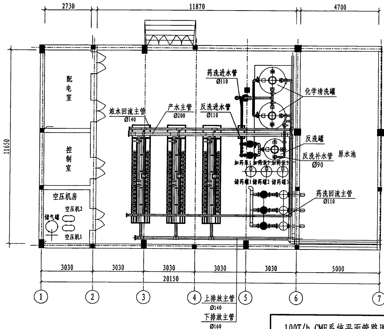
100T/h CMF系统平面管路图
