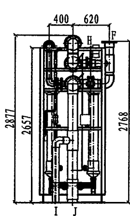
设备左视图
