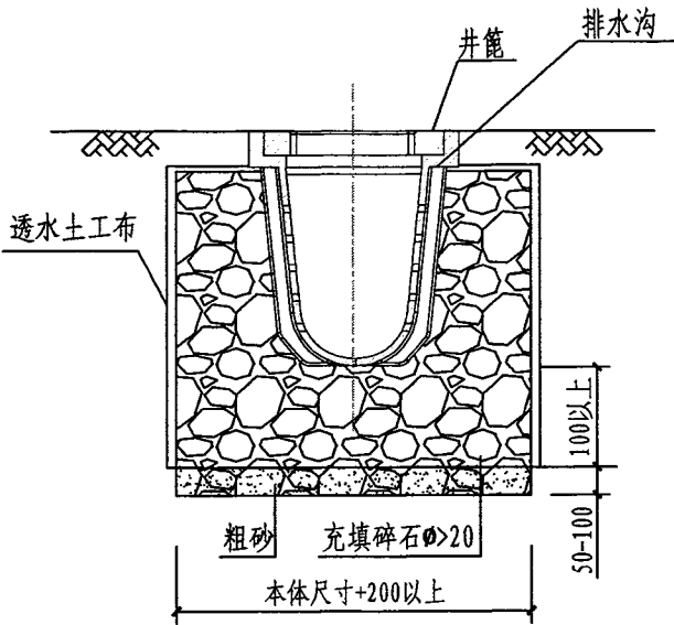
1-1剖面图
