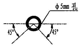
穿孔曝气管开孔剖面图
