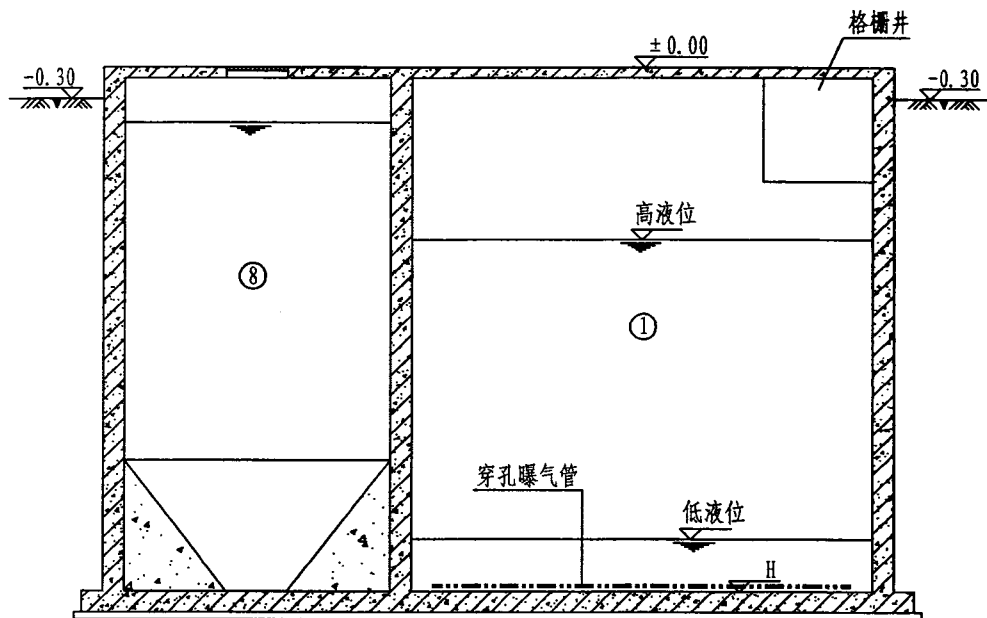
3--3剖面图
