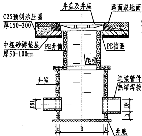
1-1剖面图
