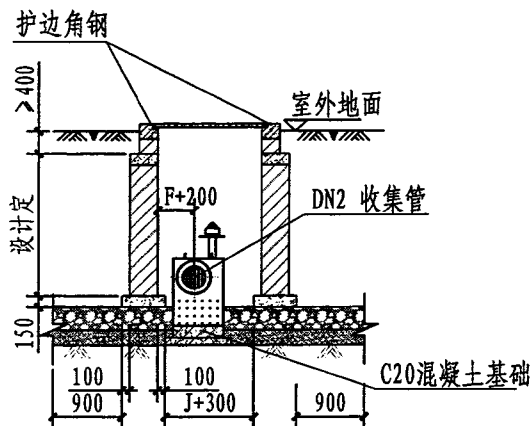
1-1剖面图
