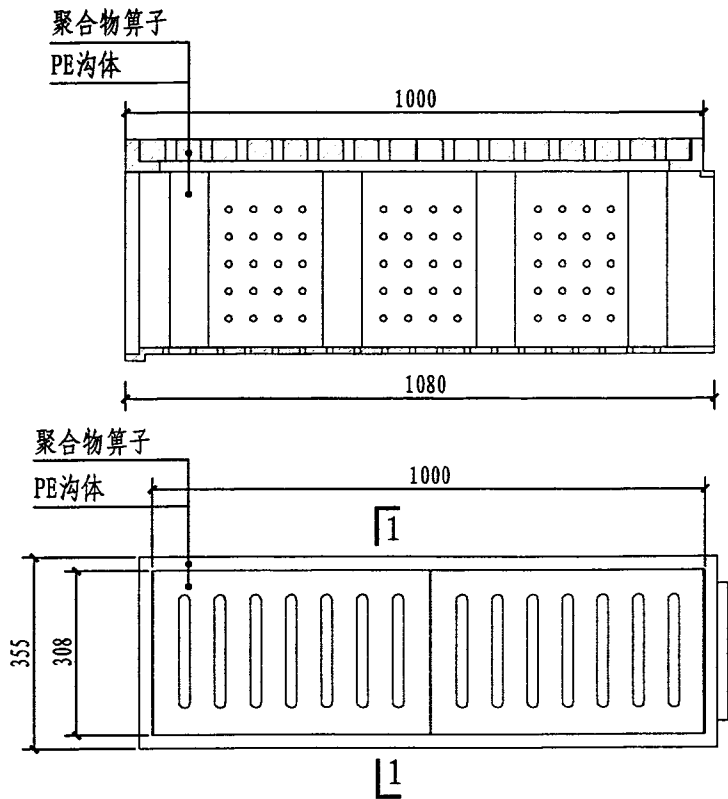
PE渗透式排水沟示意图
