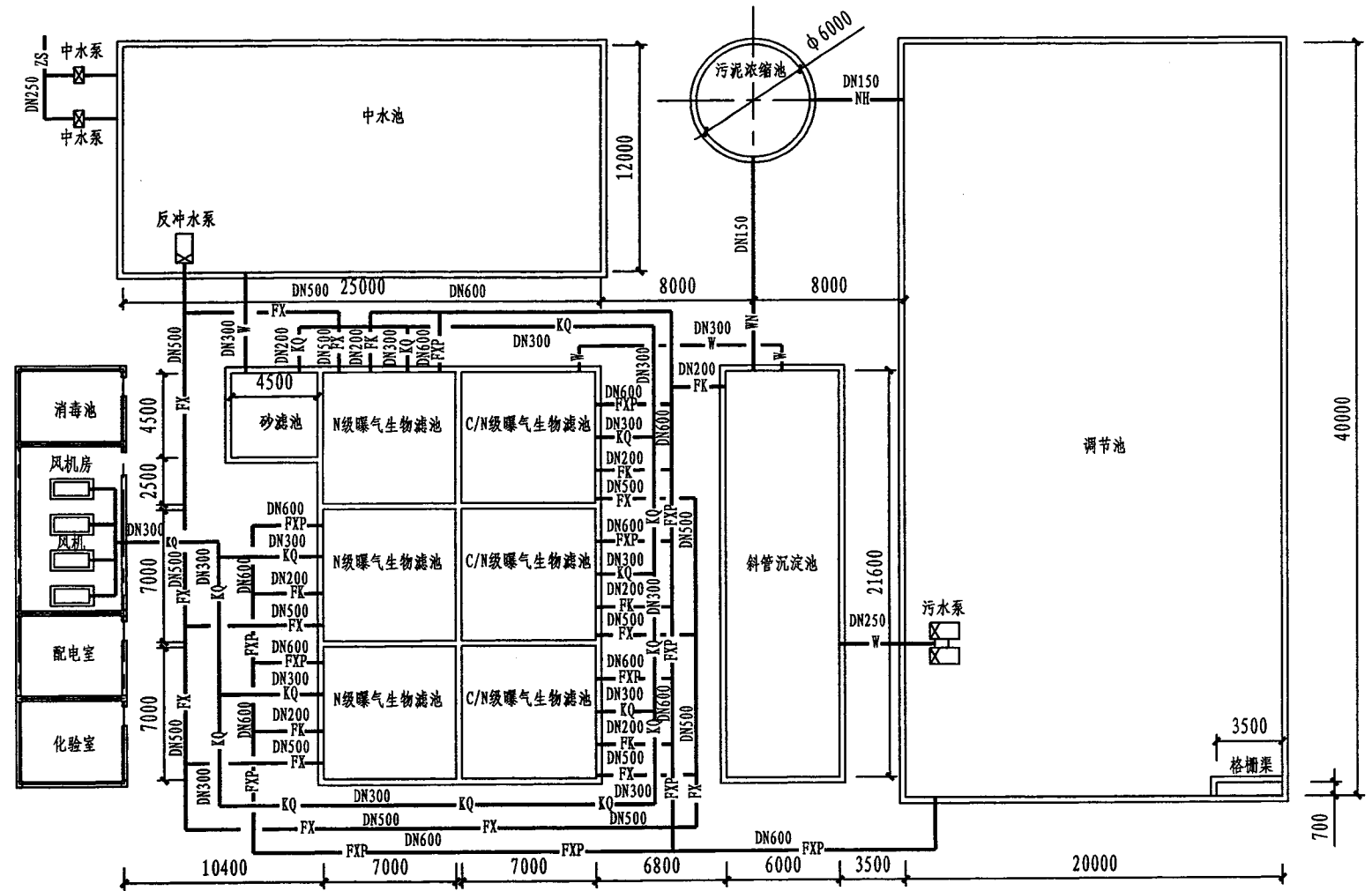
曝气生物滤池工艺管线平面图 (200m³/h)
