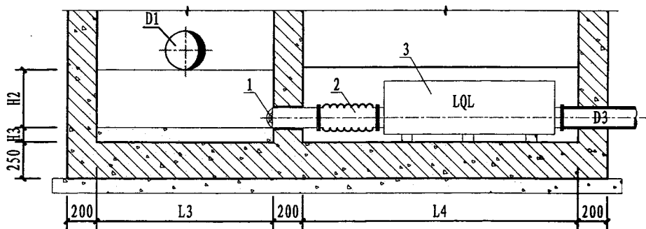
1-1剖面图
