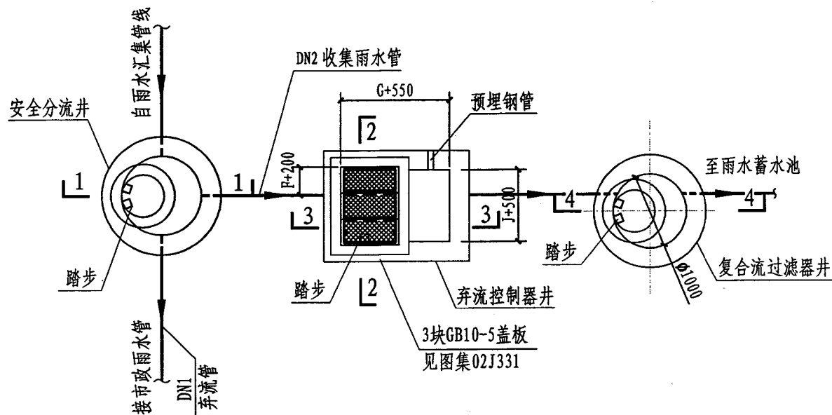
室外弃流系统平面图
