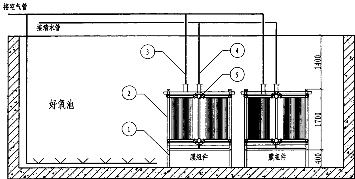
A-A 剖面图
