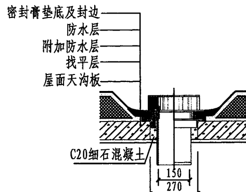
87型雨水斗安装图
