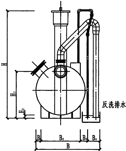
侧面图
