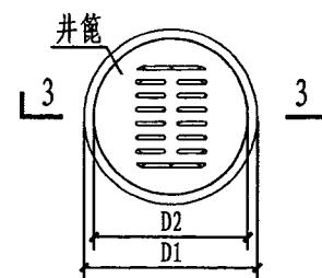
集水渗透检查井安装大样
