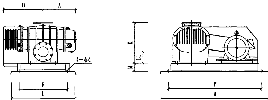
鼓风机安装大样图
