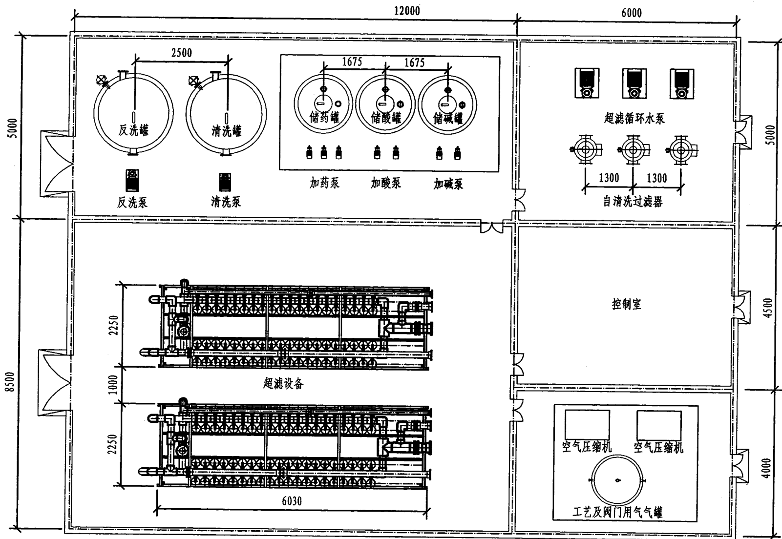
300T/h CMF系统平面布置示意图
