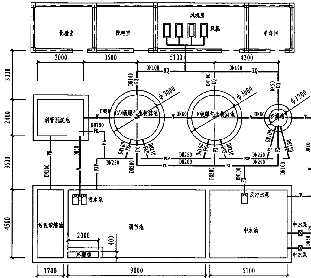
曝气生物滤池工艺管线平面图(10m³/h)
