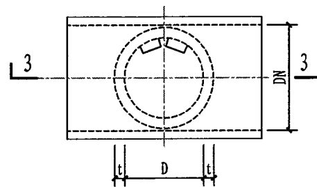
图6 管件式检查井结构图(二)
