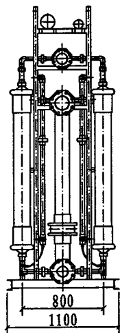
设备左视图
