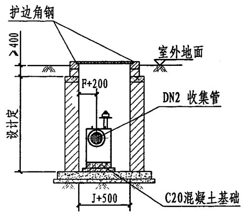
2-2剖面图 (做法II)
