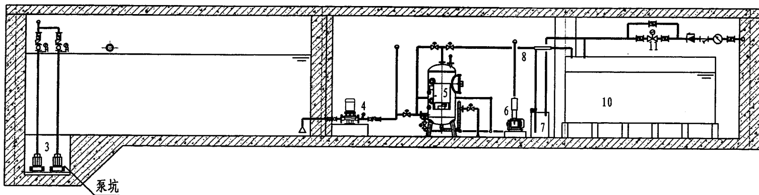
A-A剖面图
