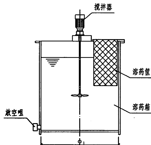
2-2 剖面图
