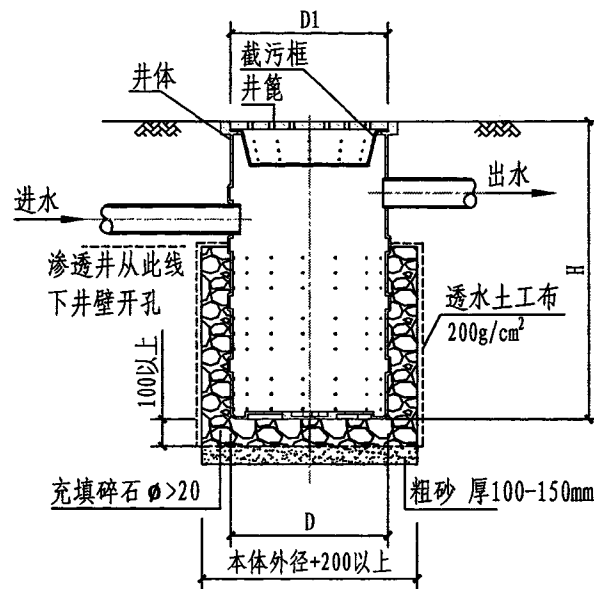
3-3剖面图
