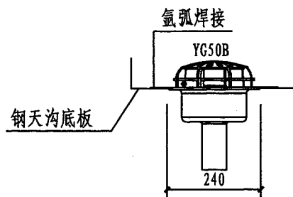
雨水斗安装大样图 (钢天沟内安装)
