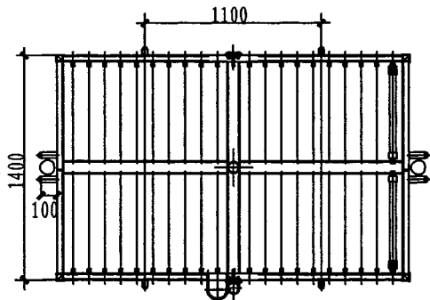
俯视图
