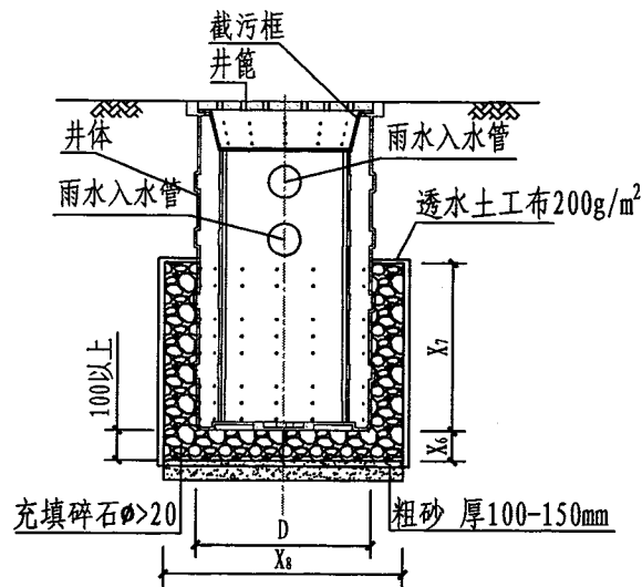
3-3剖面
