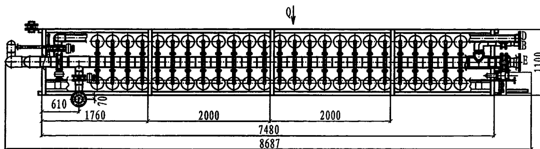
设备俯视图
