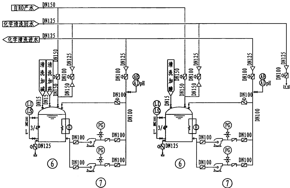
超滤化学清洗系统图
