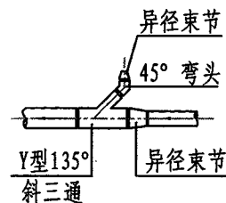
支管接入主悬吊管大样图
