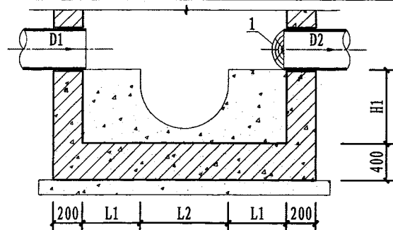
2-2剖面图
