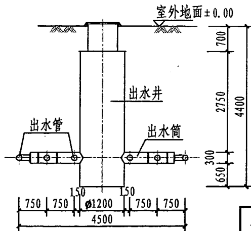
4-4剖面图
