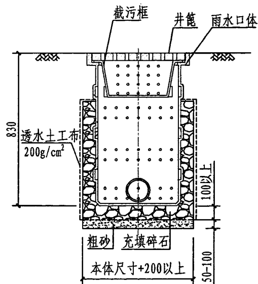
1-1剖面图
