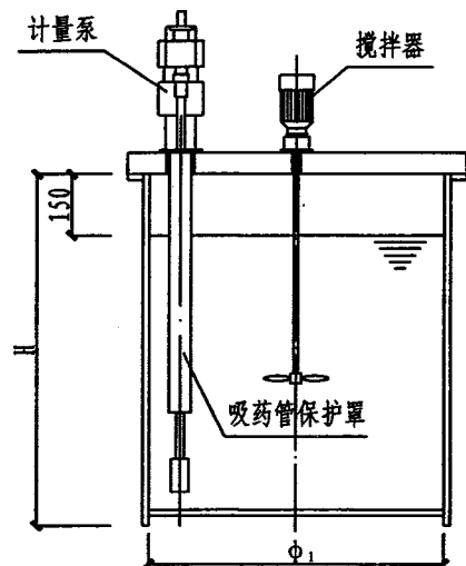
1-1 剖面图
