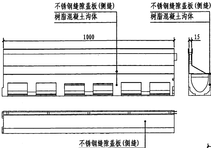
侧缝缝隙式排水沟示意图
