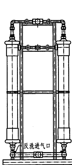
设备左视图
