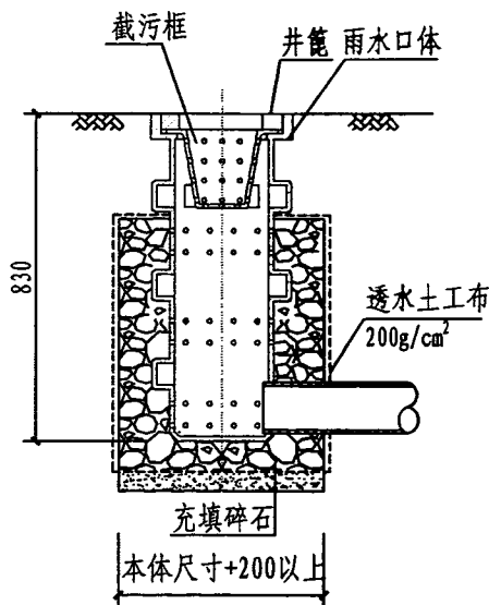
2-2剖面图
