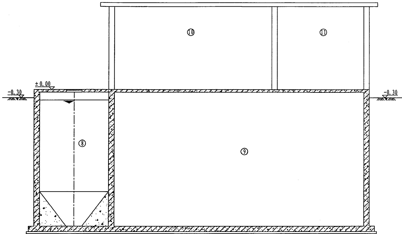
2—2剖面图
