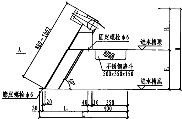
1-1 剖面图
