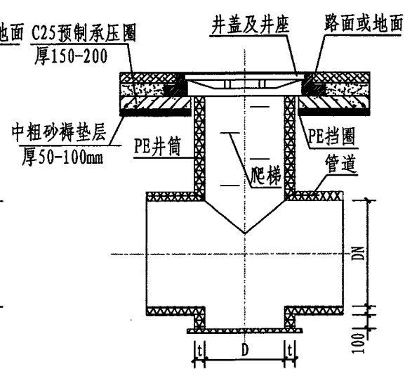
3-3剖面图
