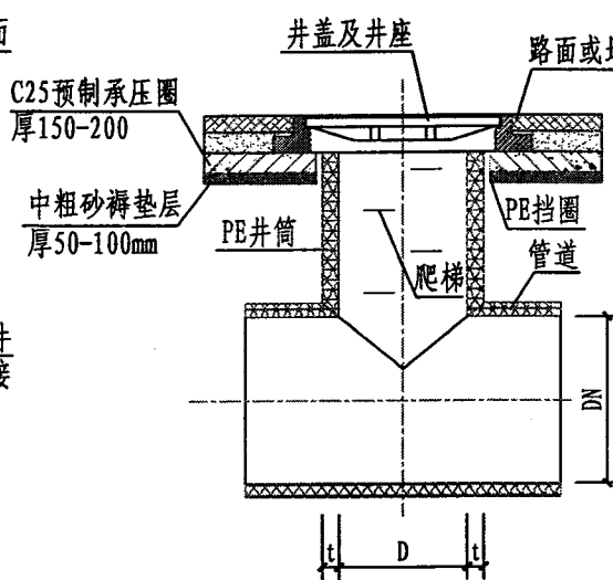
2-2剖面图
