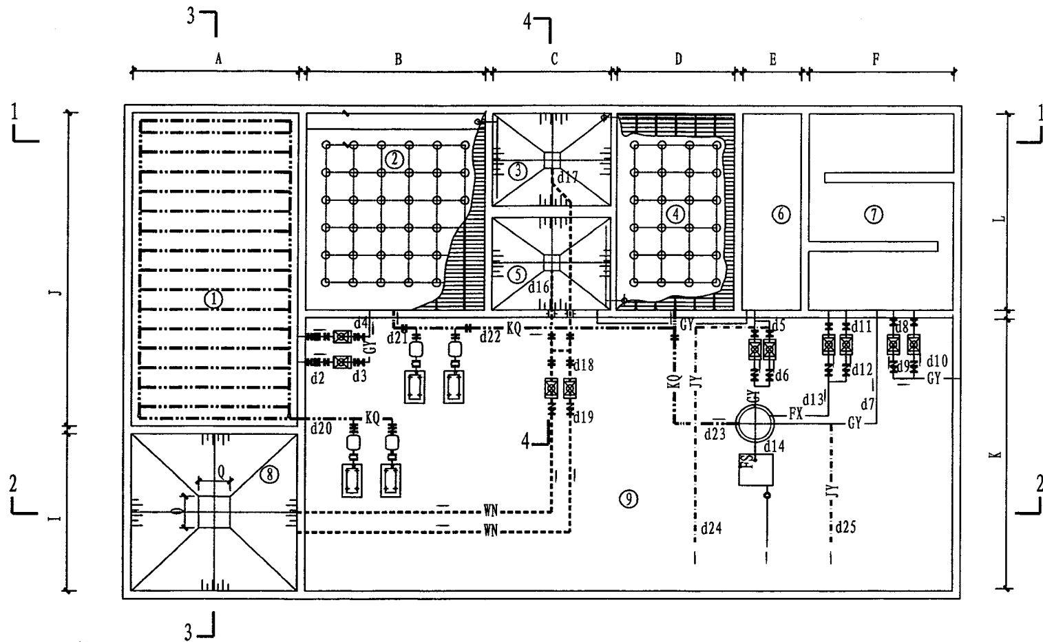
综合处理车间下部平面图
