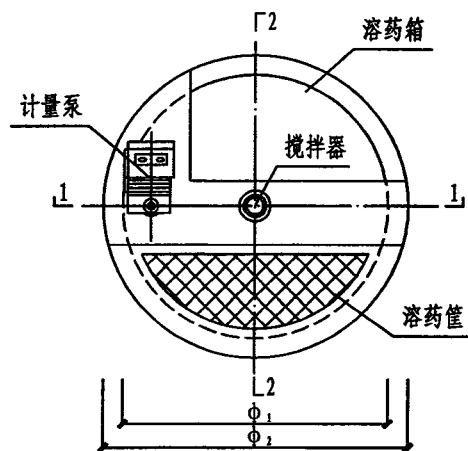
平面图
