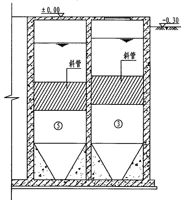
4--4剖面图
