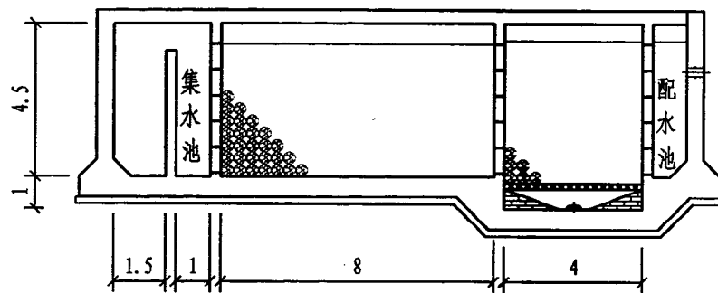
E-E剖面图
