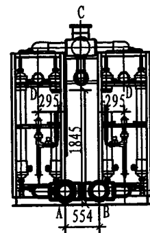
设备右视图
