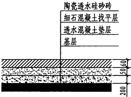
陶瓷透水硅砂砖铺装做法
