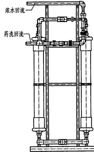
设备右视图
