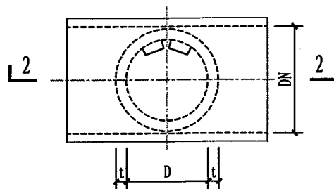
图5 管件式检查井平面图(一)
