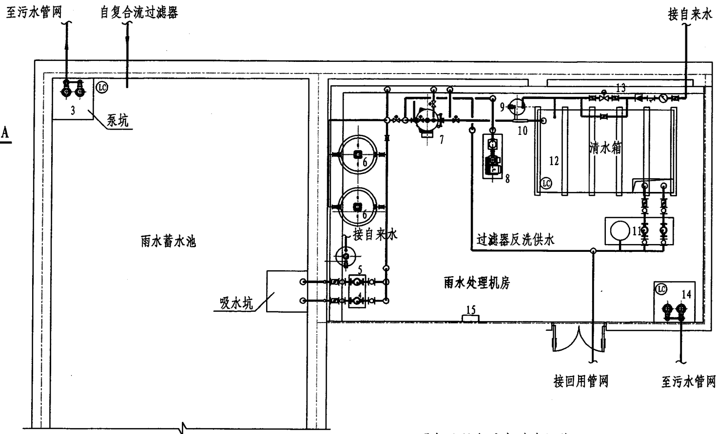
雨水（混合反应过滤）处理平面图
