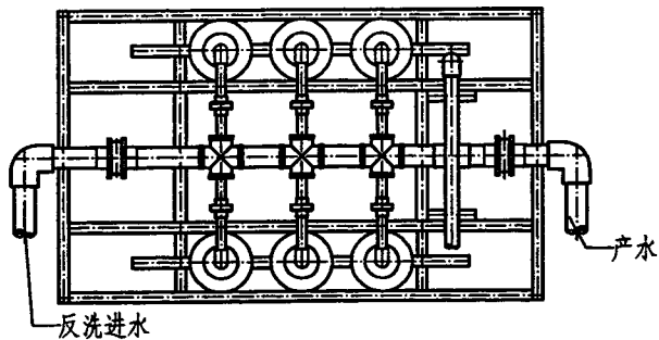
设备俯视图
