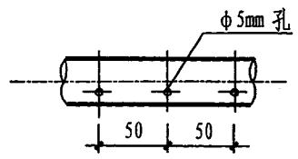
穿孔曝气管大样图
