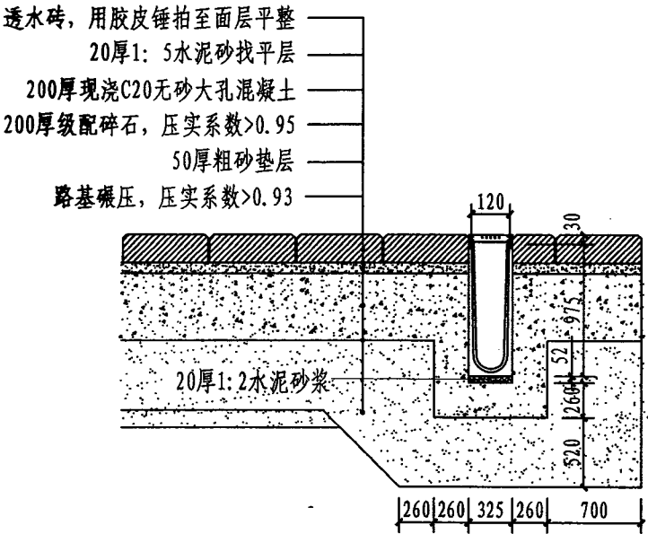
渗透式树脂混凝土排水沟安装图
