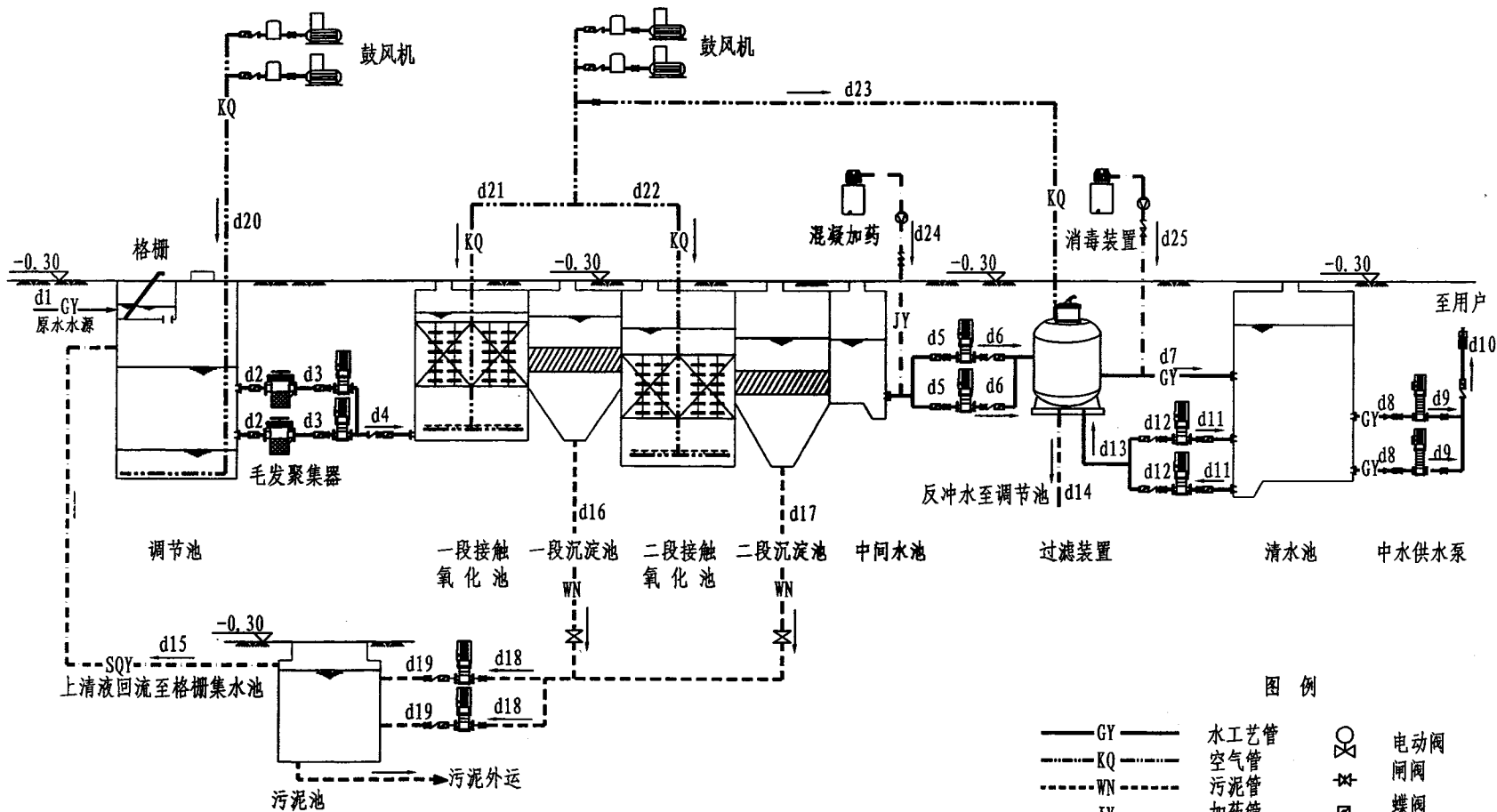
接触氧化法工艺流程图
