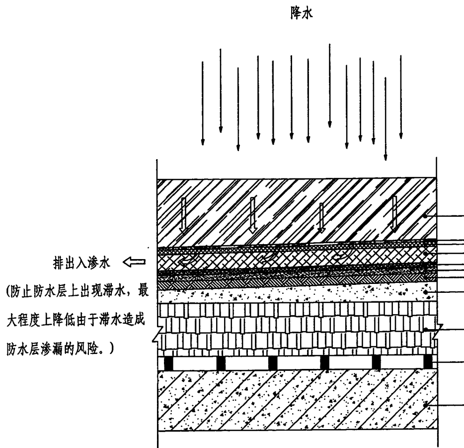
渗排材料安装构造图
