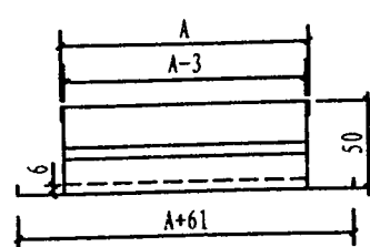
钢/不锈钢防水百叶风口
