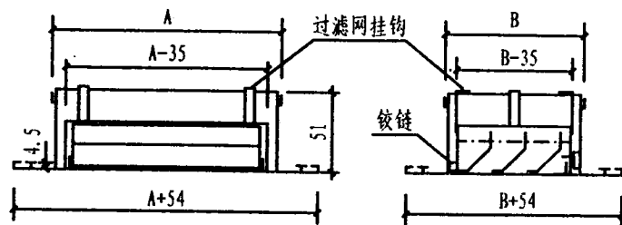
MJ (铝质宽叶片)
