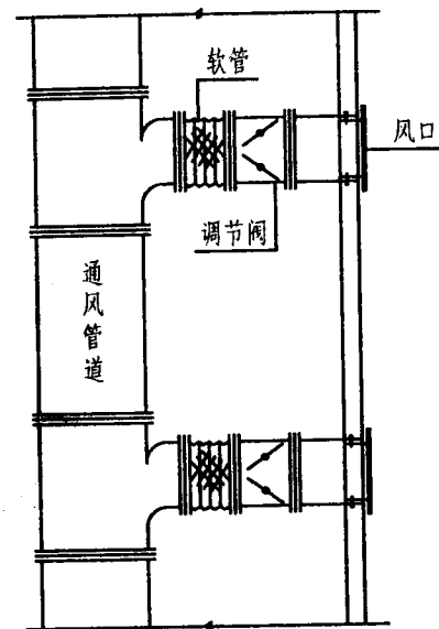
软管与风口连接示意
