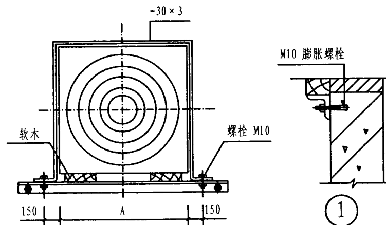
配用角钢规格
