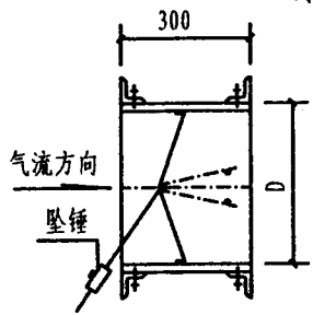
HA圆形止回阀规格表 (mm)
