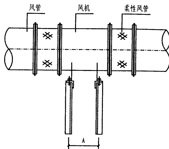
墙上支架安装
