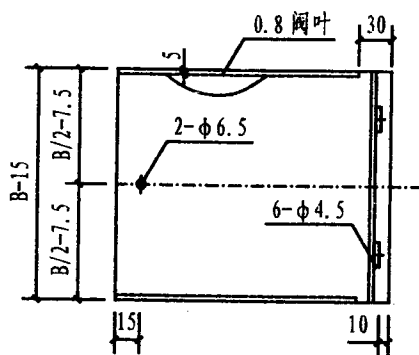
阀叶立面
