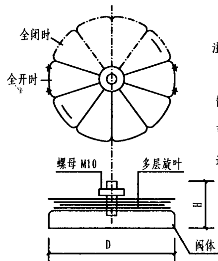
旋叶式圆形风闸
