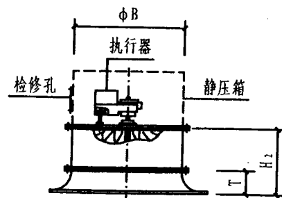
电动型
