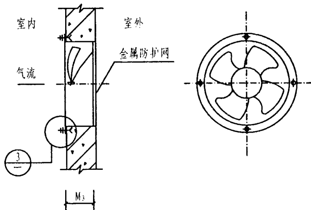
墙上安装
