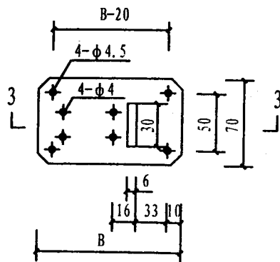
垫板
