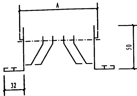
TF (B 型)
