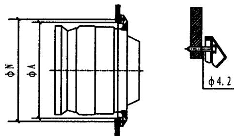
安装于墙上
