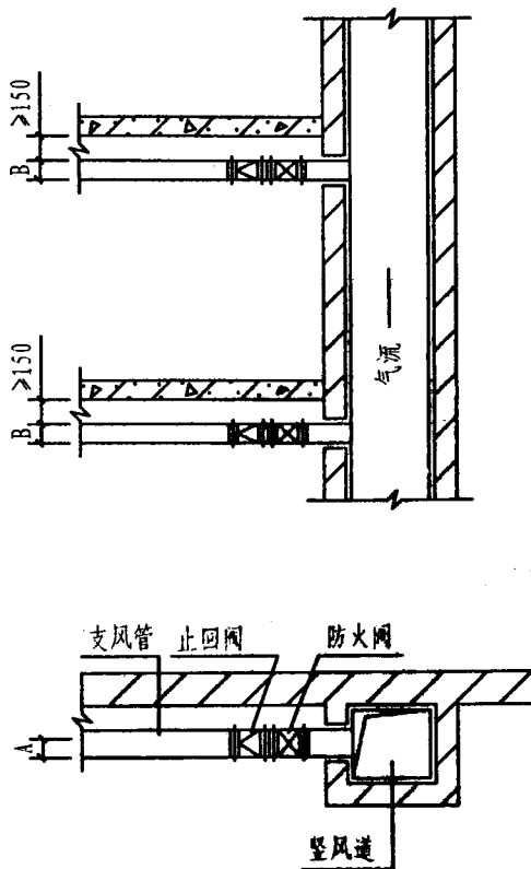
做法 (2)
