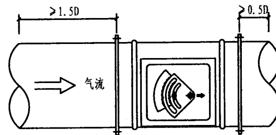
安装示意
