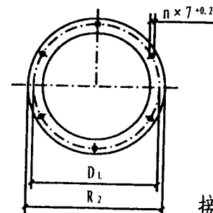
垂直接管型
