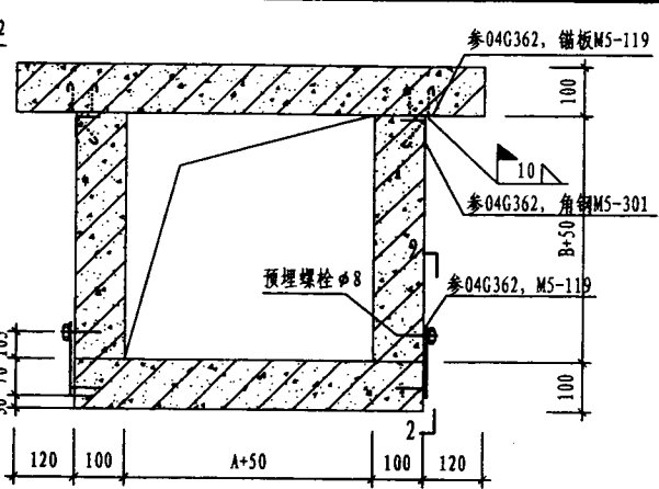
混凝土预制框埋件示意图
