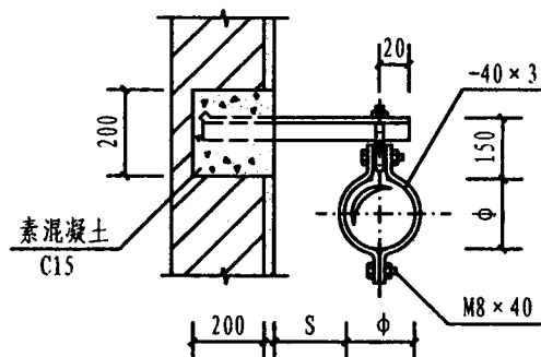
圆形不保温风管墙上吊架
