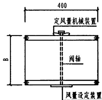
俯 视
