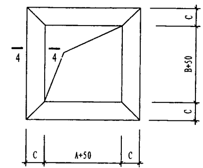
预埋钢框立面图
