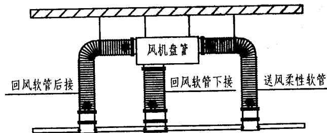
风机盘管与风管连接示意
