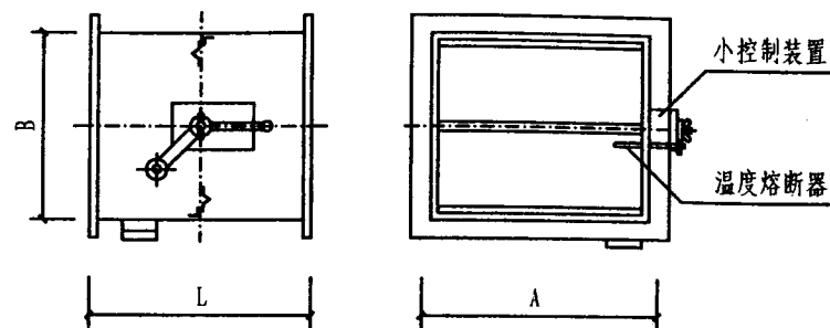
小型防火调节阀 HAFH-4 型
