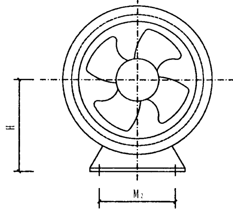
GYF-I 型
