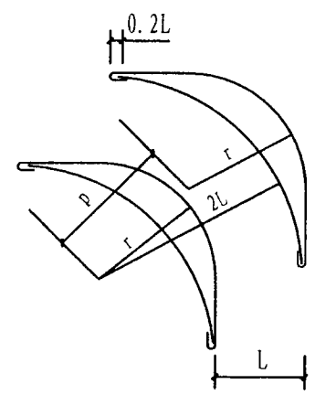
双层做法
