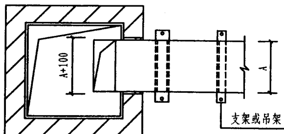
D. 土建竖风道与水平风管连接 (二)
