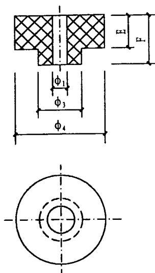
橡胶减振器
