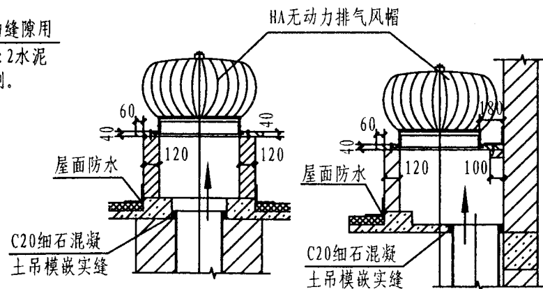
风帽四面不靠墙时
