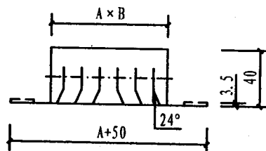
双向送风
