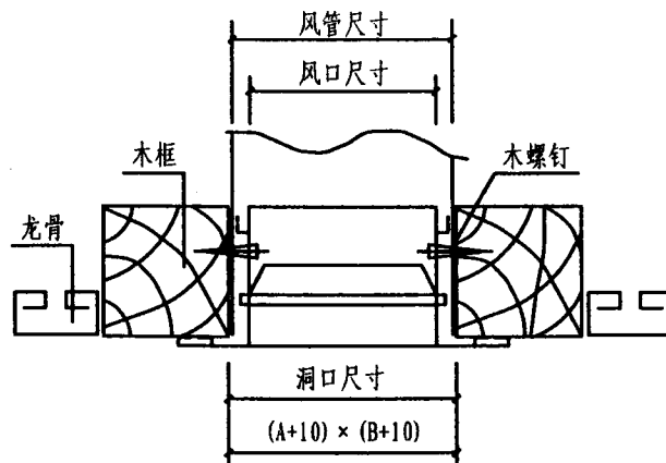
外木框安装法 (二)
