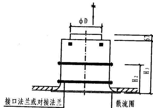
垂直接管型
