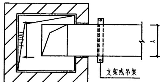
E. 土建竖风道与水平风管连接 (三)
