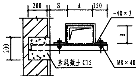
矩形不保温风管墙上支架
