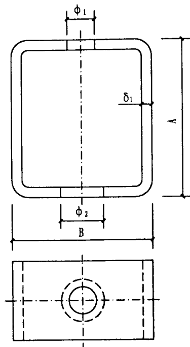
框 架
