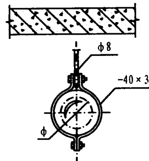
圆形保温风管单杆吊架
