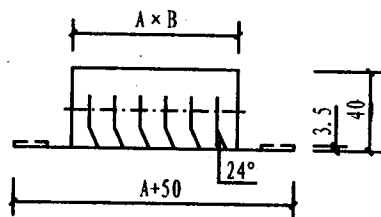
单向送风
