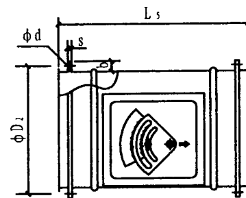
圆形机械式定风量阀 (法兰口)
