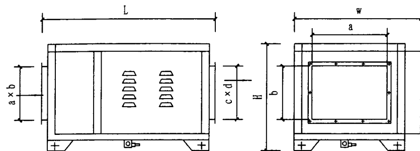
CF2~10油烟净化器外形图
