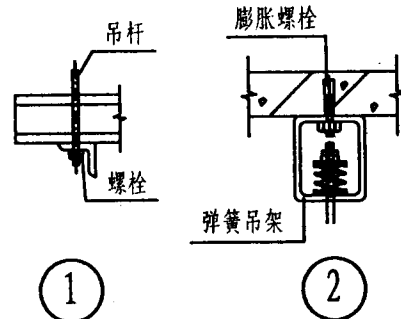
吊装
