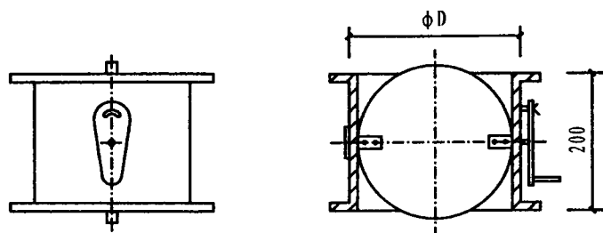
圆形手柄钢制蝶阀
