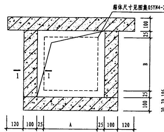
混凝土预制框立面图
