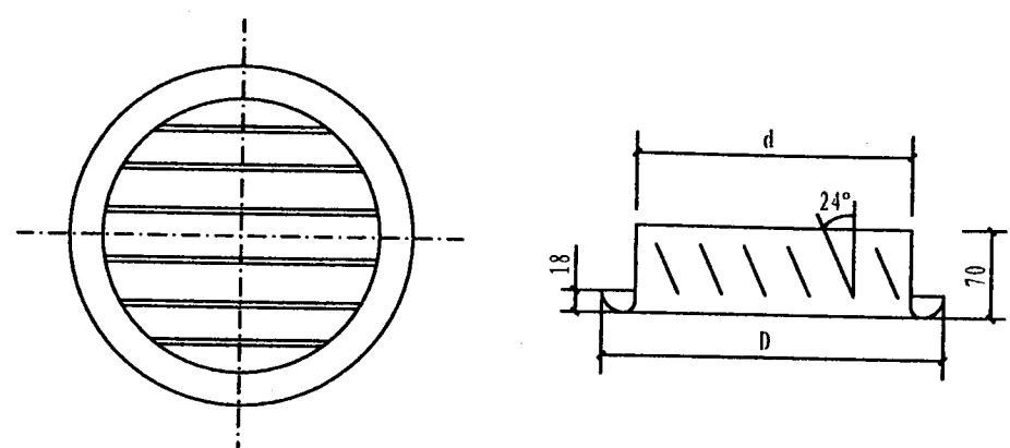
YS (斜片型)
