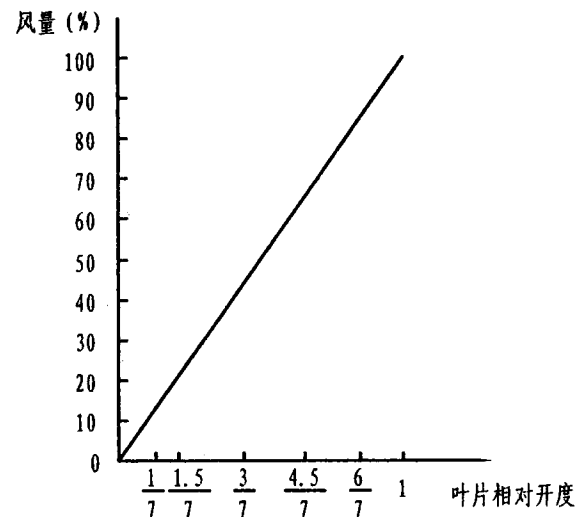
性能曲线
