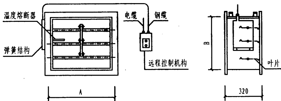
远控防烟防火调节阀 HAFFH-17 型
