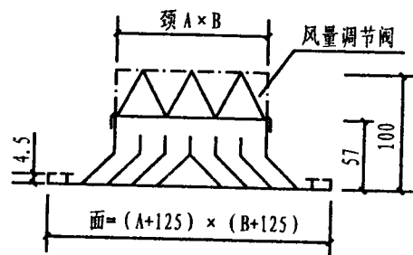
JS (铝)
