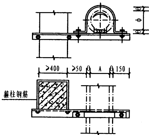
圆形保温风管柱上支架 (一)
