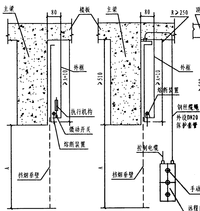
HA-FA型翻板式挡烟垂壁 安装示意图
