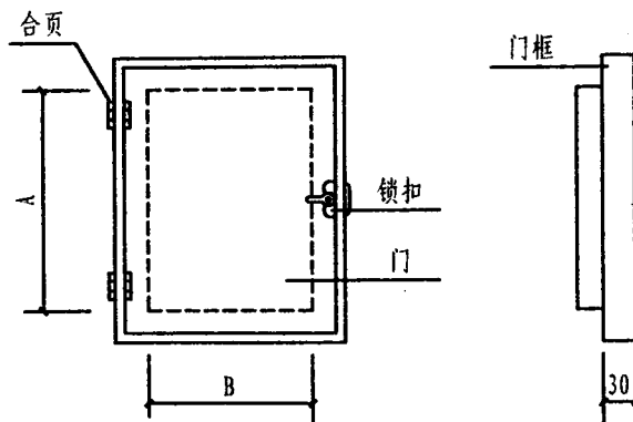
管道修理门
