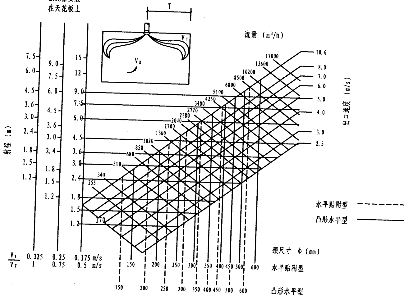
圆形散流器性能曲线
