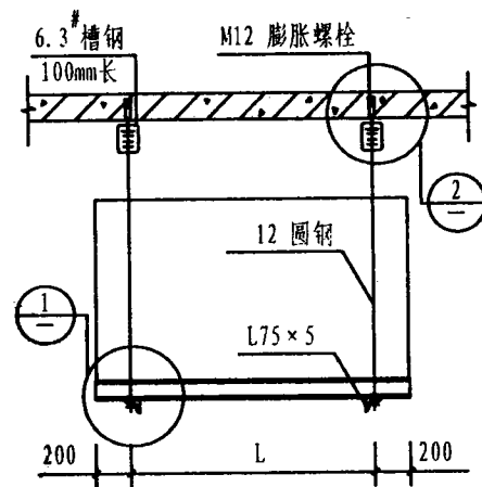
吊装
