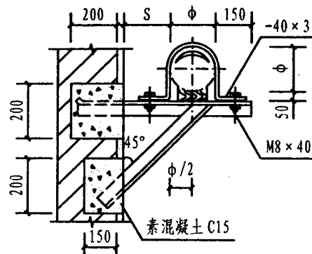
圆形保温风管墙上斜撑支架
