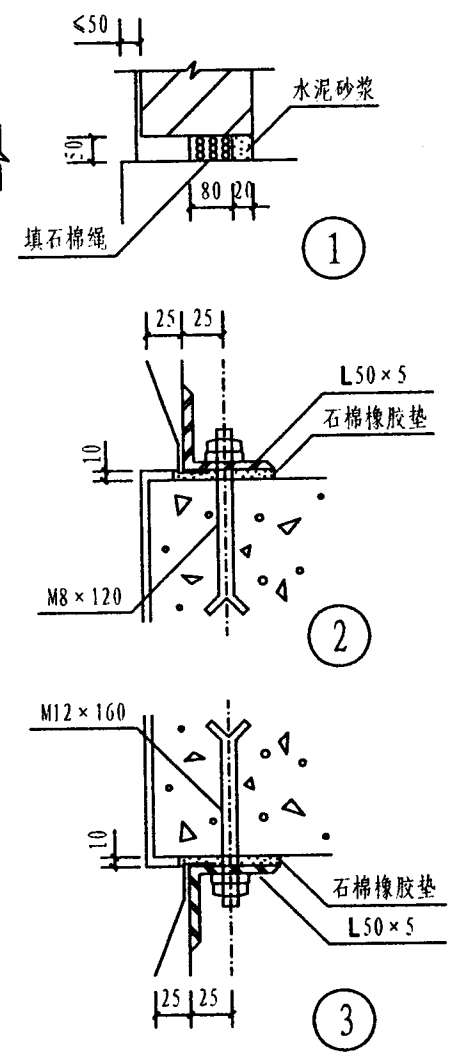
C. 土建风道下接风管
