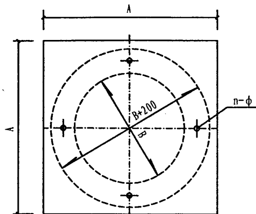
轴流式屋顶风机
