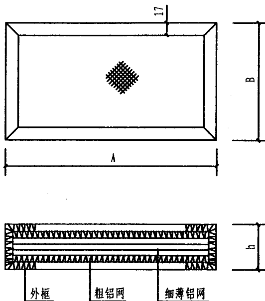
铝合金风口过滤器
