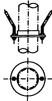
圆形不保温竖向风管吊架
