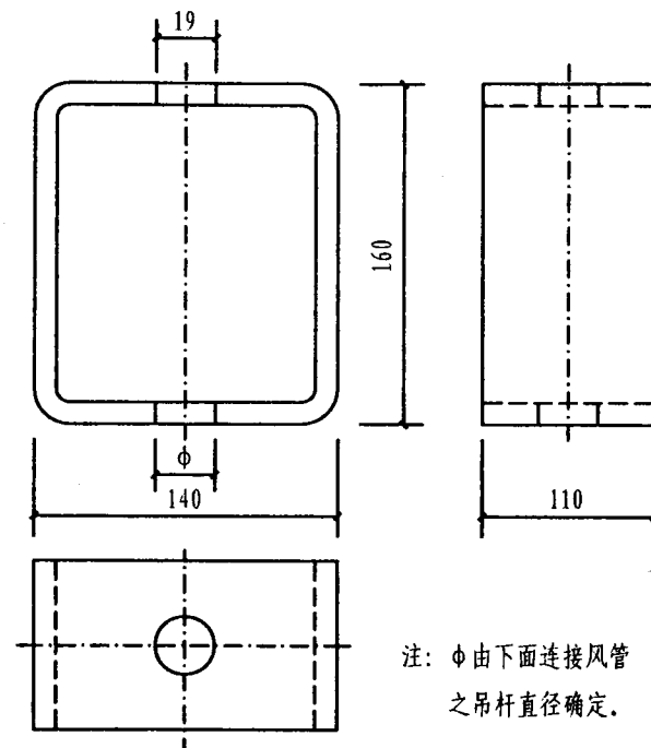
连接件
