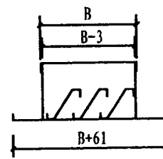
钢/不锈钢防水百叶风口
