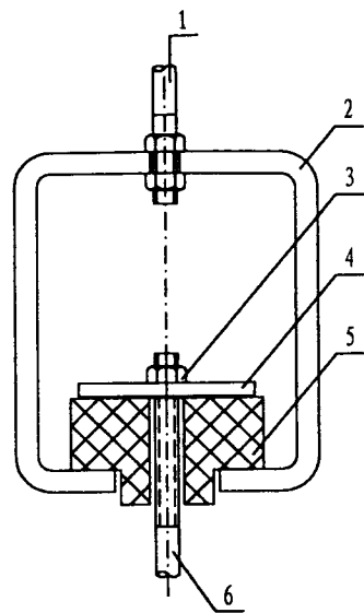
XTG 型弹性吊架
