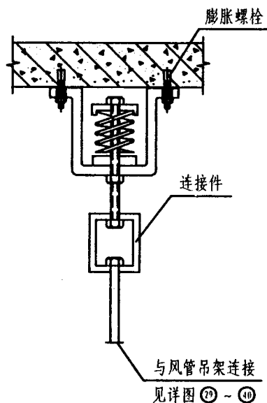
安装示意图
