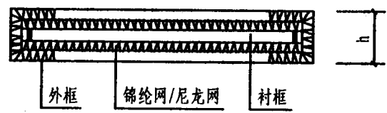
锦纶风口过滤器
