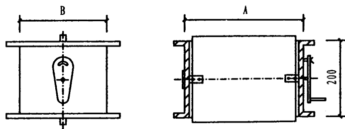
方、矩形手柄钢制蝶阀
