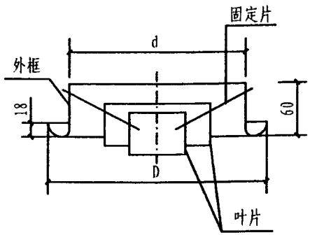
YS (圆环型)
