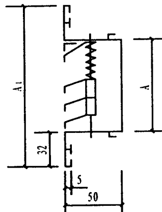
TF (活芯式)
