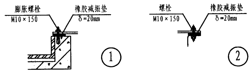
排烟(厨房)屋顶风机安装
