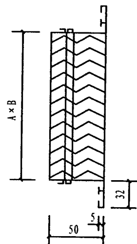
遮光百叶
