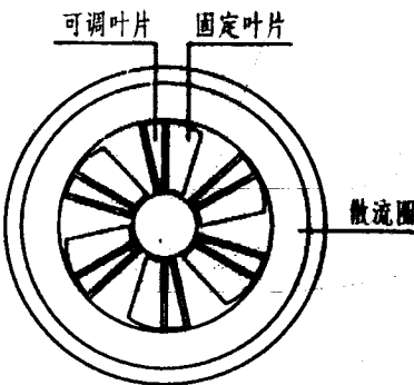
送风方向 45^{\circ} 时的叶片状态 (等温送风)
