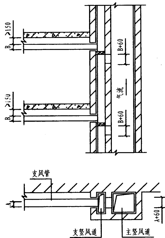
做法 (3)
