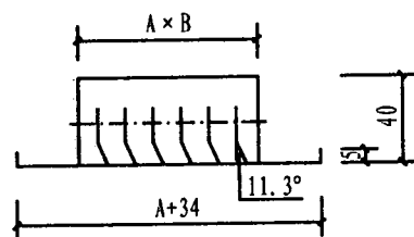
单向送风
