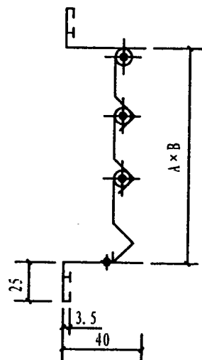
自垂百叶
