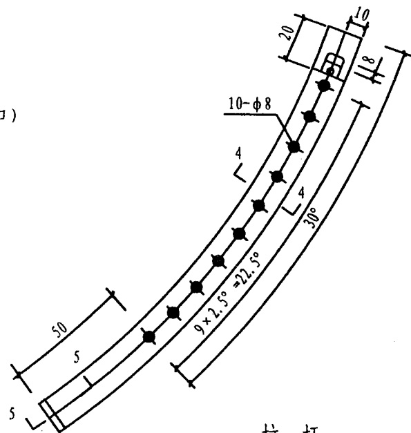
拉杆
