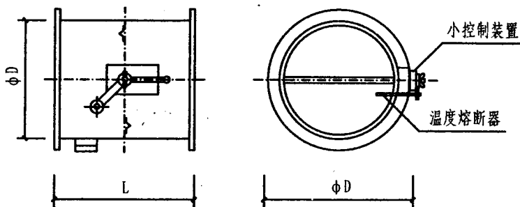
小型防火调节阀 HAFH-5 型
