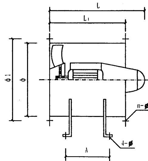
GYF-II 型
